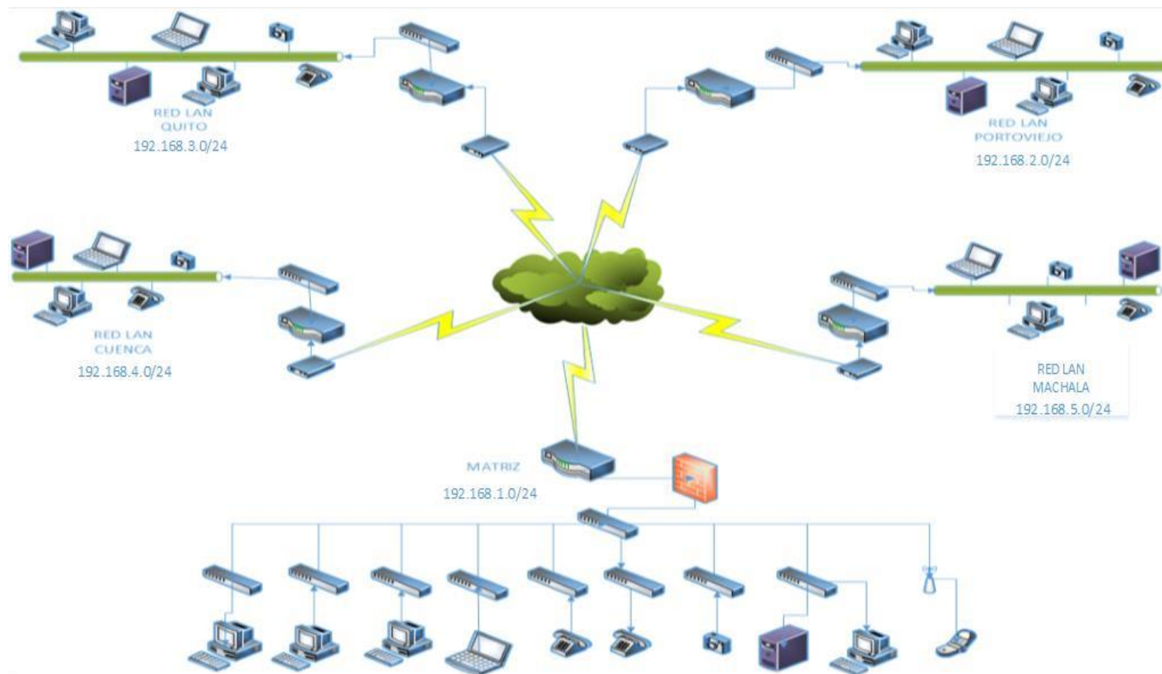
Figura 1.3 Red empresarial existente
