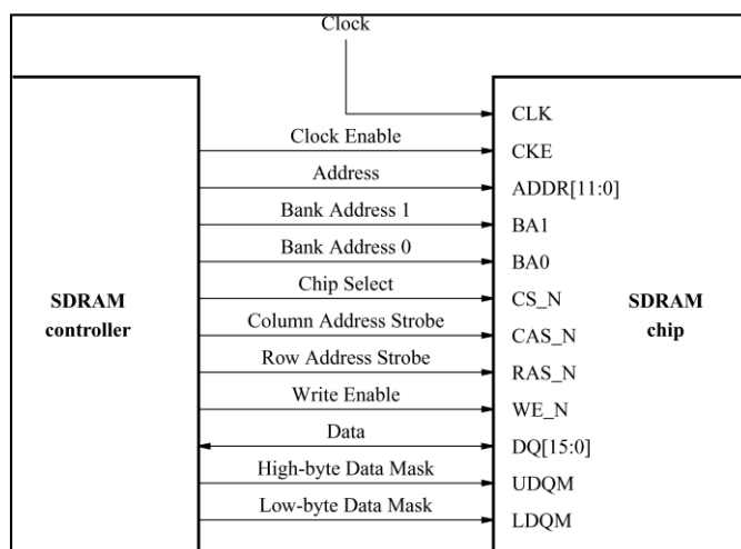
Señales del chip SDRAM y el controlador
