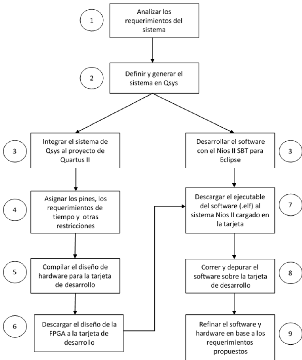
Figura 2.8 Flujo de desarrollo para la creación de un sistema Nios II [13]
