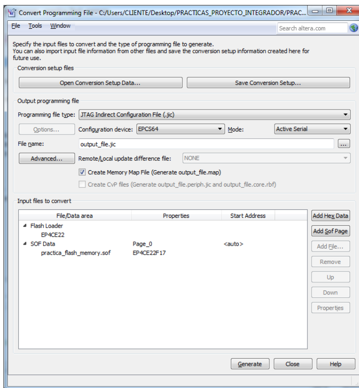
Figura 22. Configuraciones finales para cargar sistema en la EPCS64
