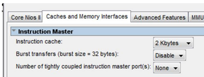
Figura 10. Ajuste de la interfaz de memoria y memoria cache del procesador.
