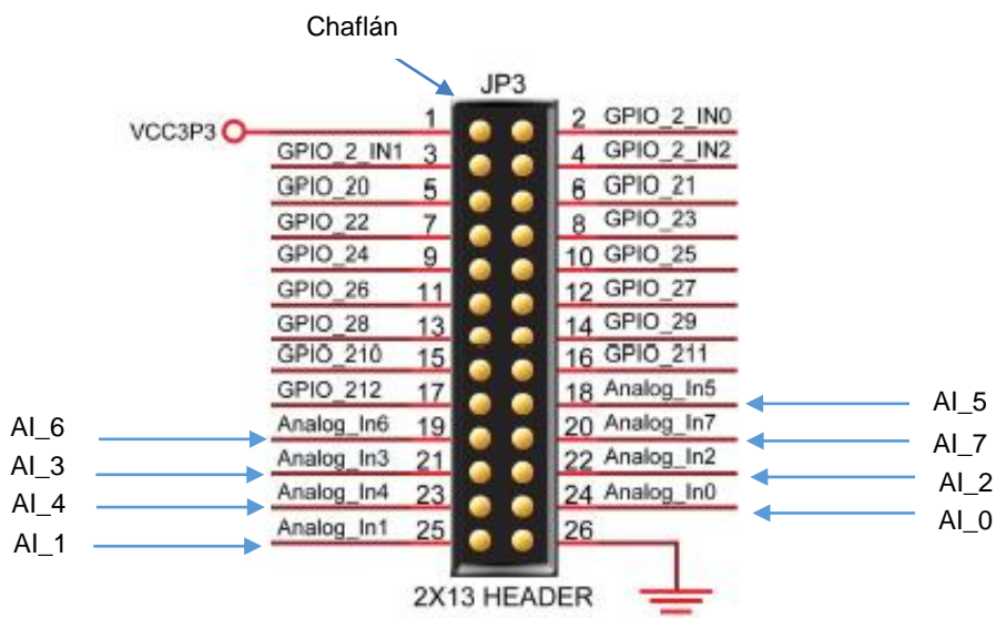
Figura 1. Ubicación de las entradas analógicas en el cabezal de pines 2x13 (vista superior)
