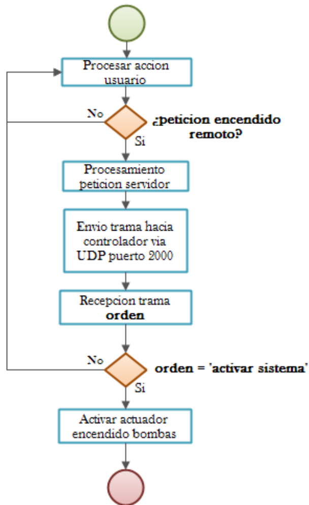
Figura 2. 29: Diagrama de flujo del proceso de envío de orden remota hacia el controlador.
