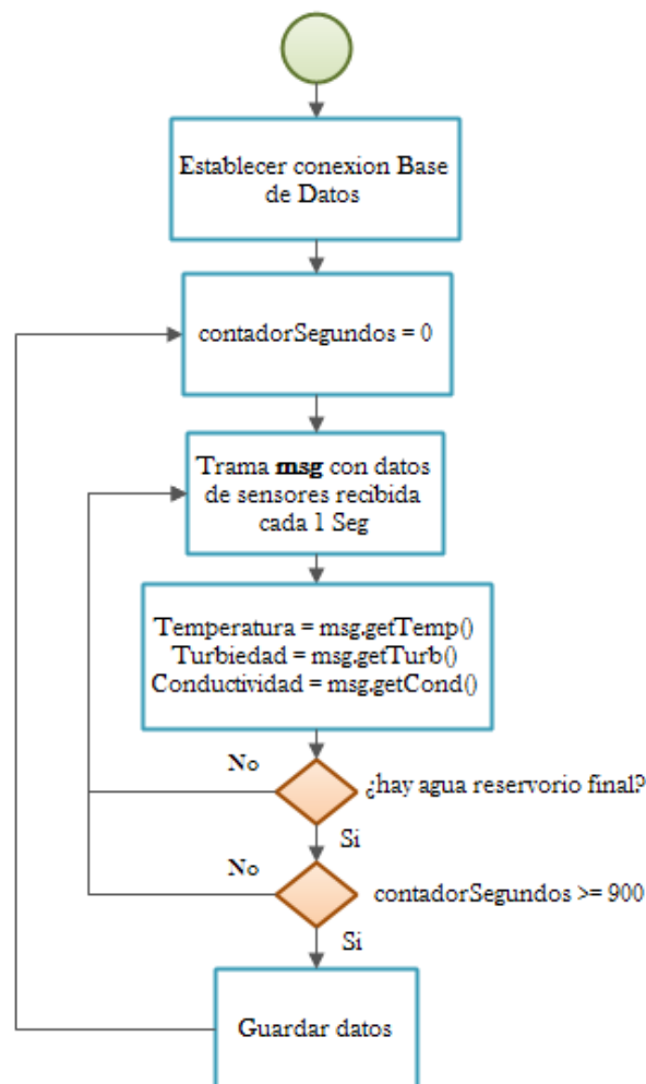
Figura 2.26: Diagrama de flujo del proceso de almacenamiento de datos
