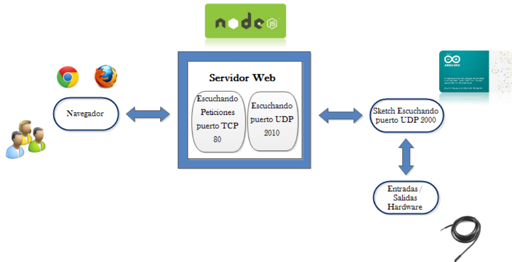
Figura 2.24: Diagrama de bloques de comunicación entre los componentes de software
