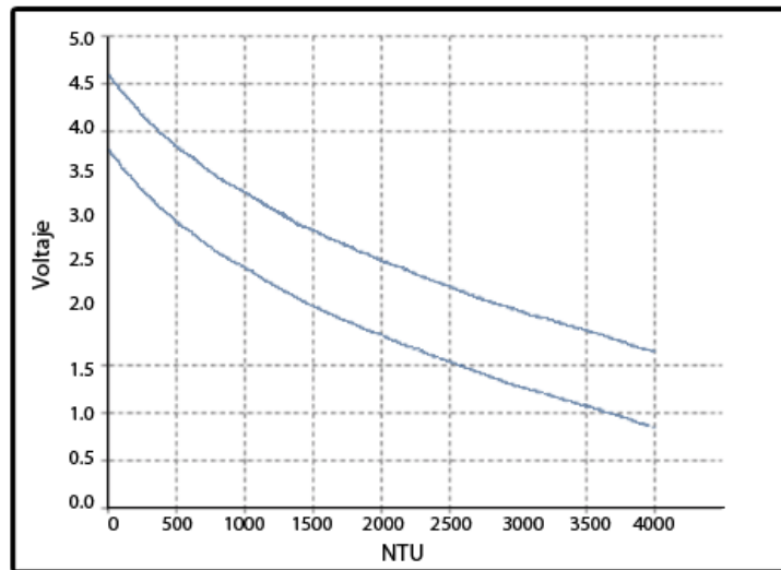
Figura 2.50: Gráfica de calibración del sensor de turbidez
