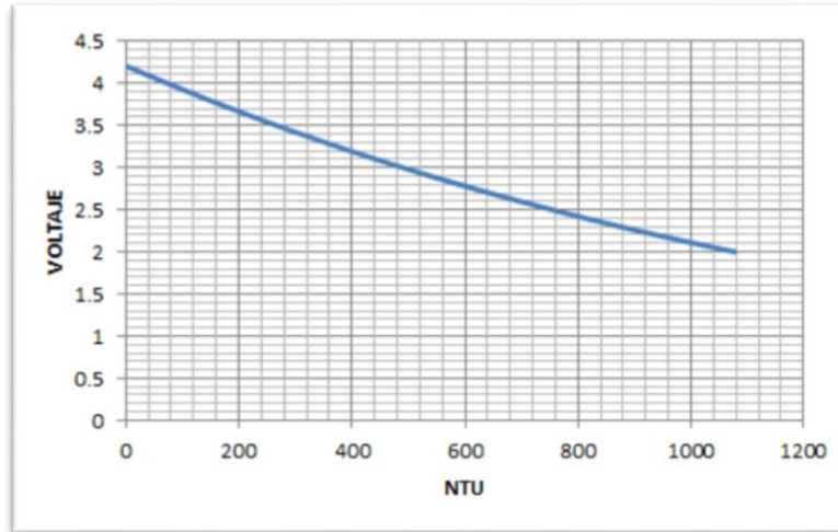
Figura 4.6: Gráfica de los valores obtenidos durante la calibración.
