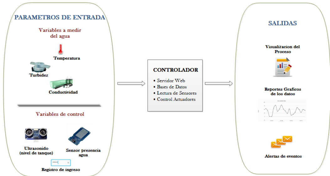
Figura 2. 18: Diagrama de bloques del sistema de potabilización
