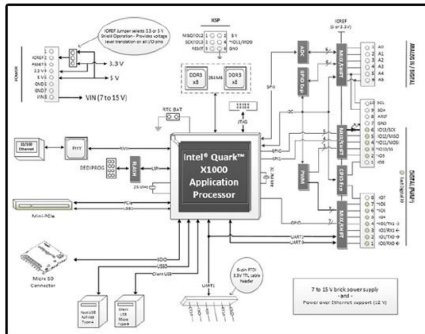
Figura 2.36: Diagrama de bloque Intel galileo gen 2.
