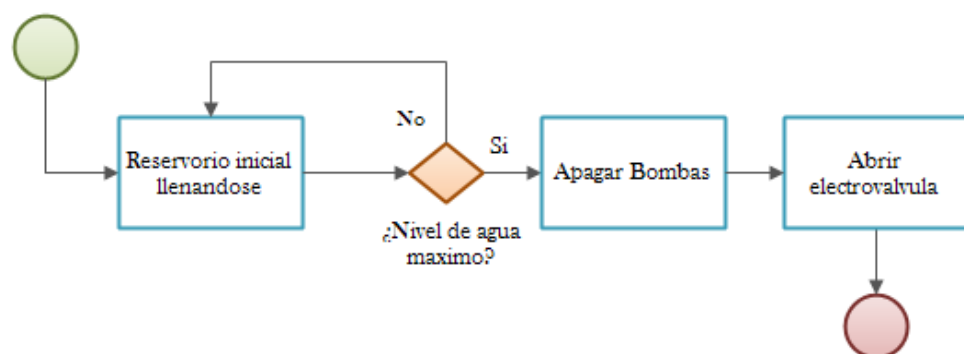
Figura 2. 22: Diagrama del proceso de llenado del reservorio inicial
