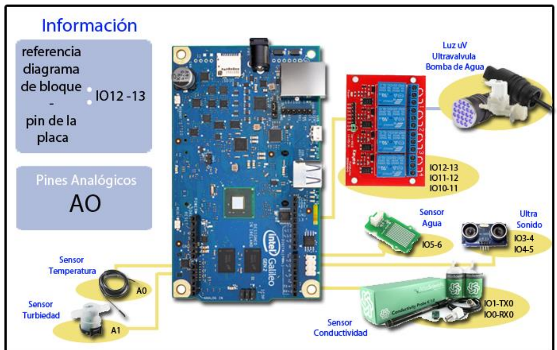
Figura 2. 47: Esquema básico de como es el sistema.
