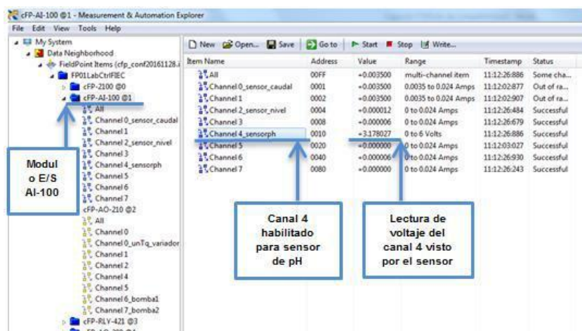
Figura 3.3: Habilitación del canal 4 del AI-100 para lectura del sensor de pH
