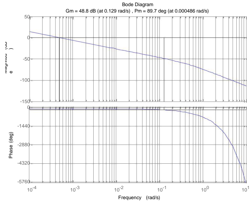
Figura 3.15: Diagramas de Bode de subida con control PD, K_c=1 y polo en -0.3510
