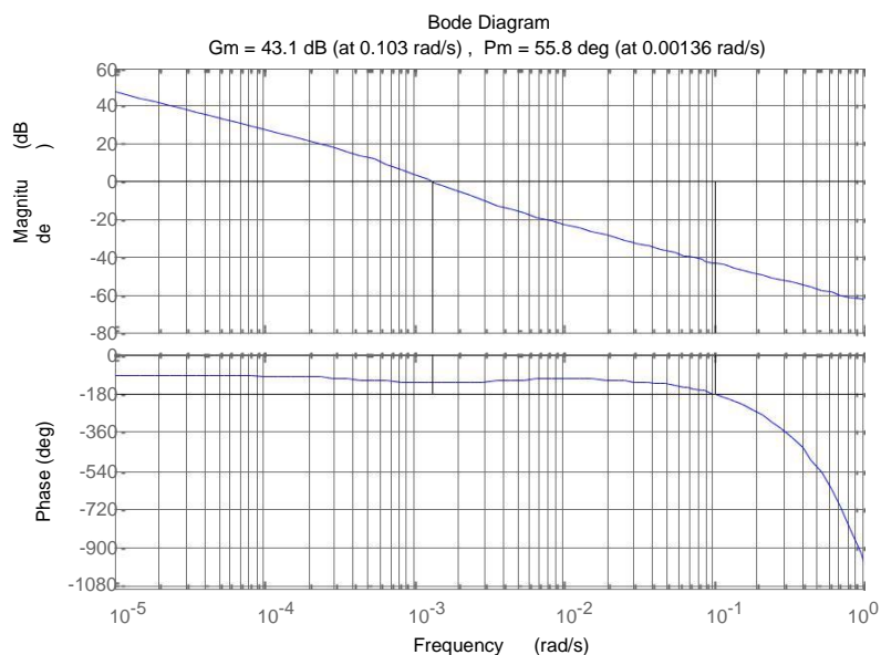
Figura 3.18: Diagramas de Bode del modelo de bajada
