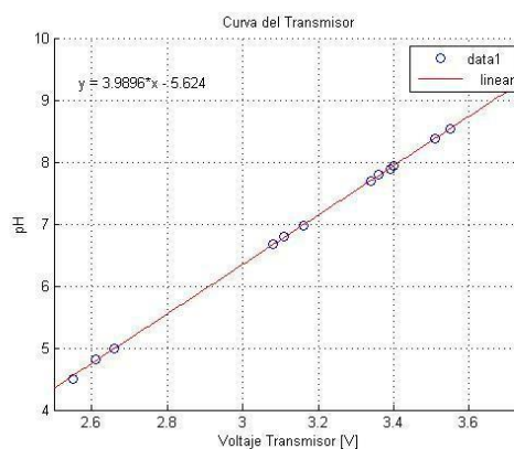
Figura 3.7: Curva del sensor de pH
