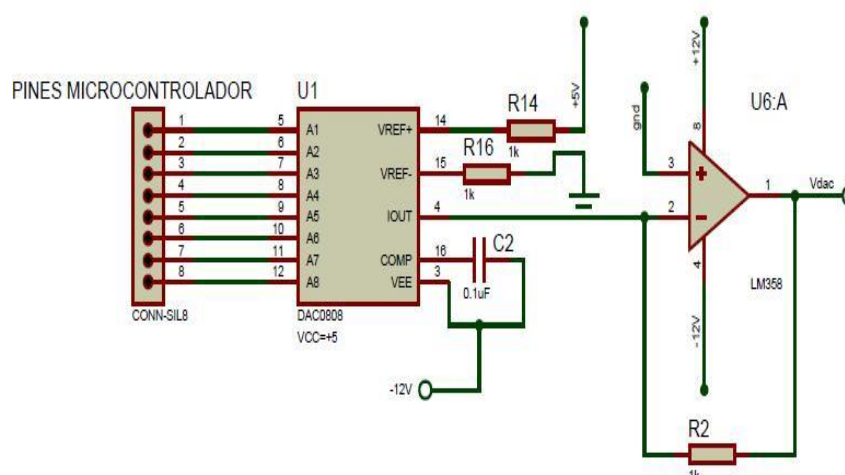
Figura 3.21: Conversor digital a analógico
