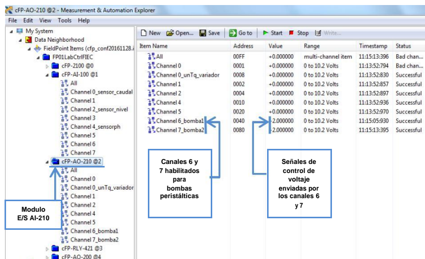
Figura 3.4: Habilitación del canal 6 y 7 del AO-210 para enviar señales de control a las bombas
