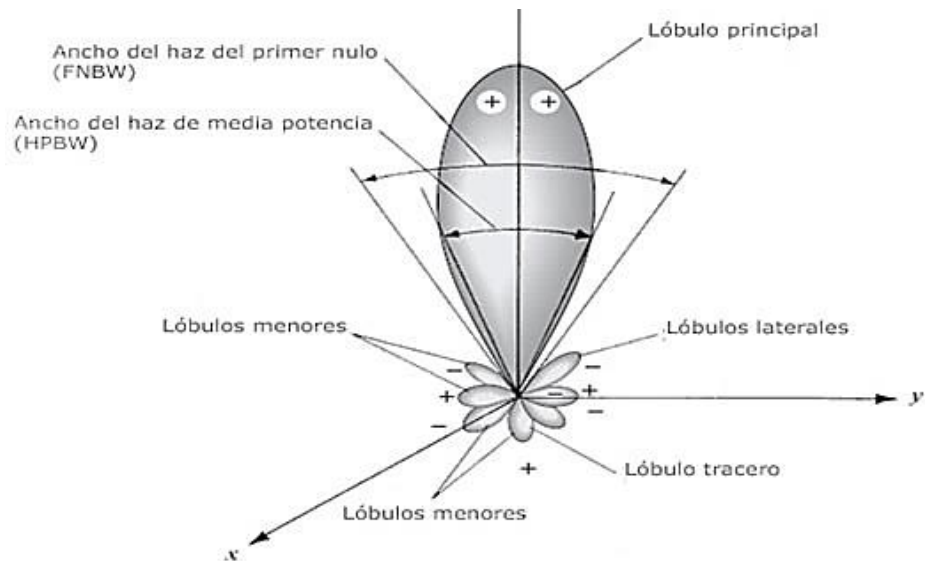
Figura 2.2 FNBW y HPBW junto con red de lóbulos [17].
