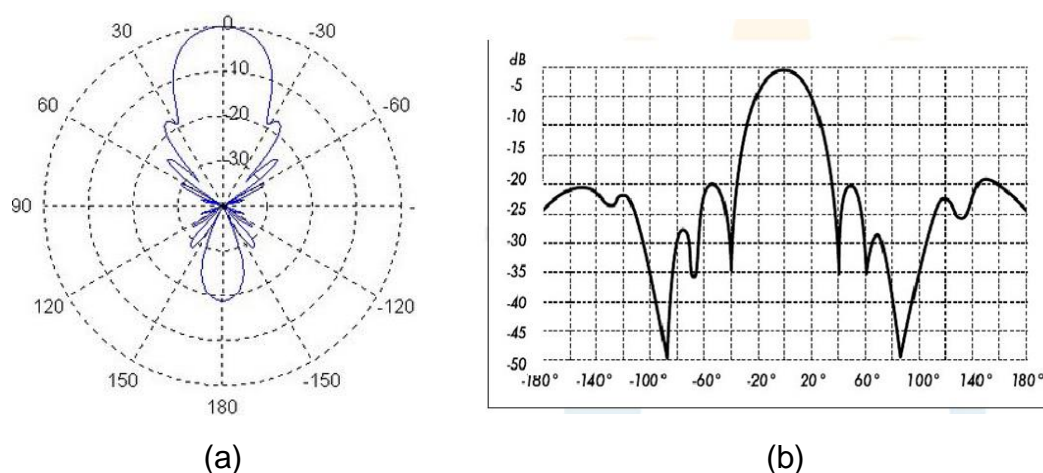
Figura 2.1 Patrón de radiación: (a) en coordenadas polares (b) en coordenadas rectangulares
