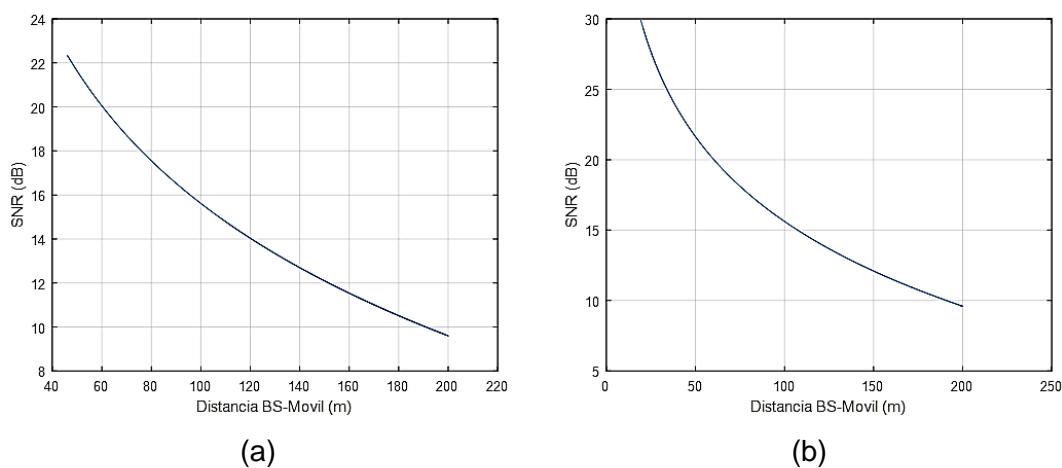
Figura 3.7 Curvas SNR vs Distancia entre la Base y el móvil (a) Primer recorrido (b) Segundo recorrido
