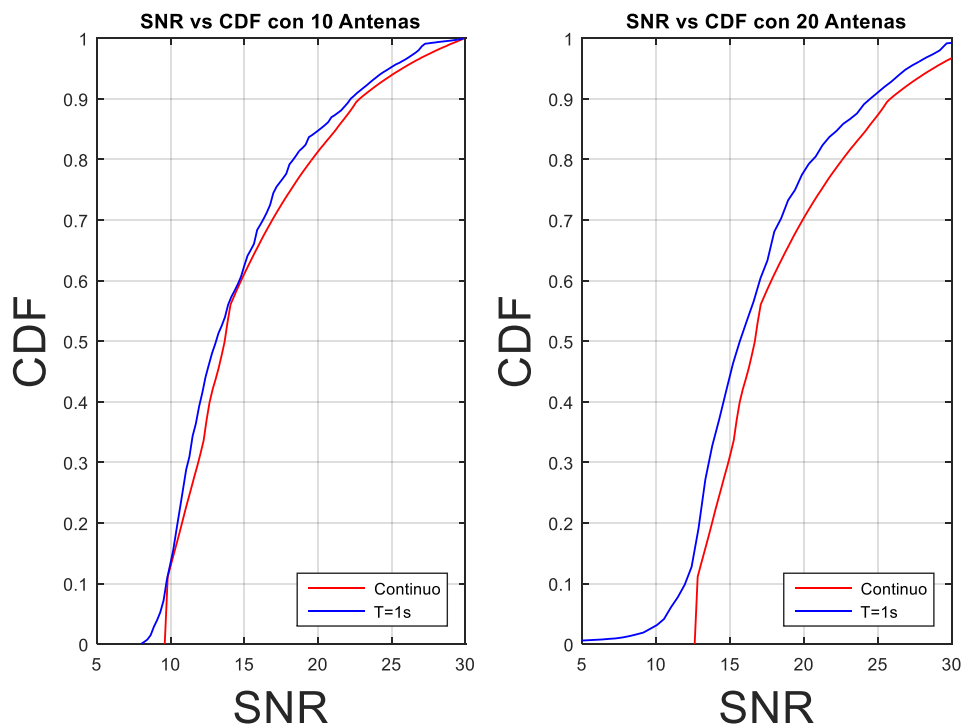
Figura 3.23 Comparación de CDF vs SNR para una ULA con 10 y 20 elementos hacia un móvil con una velocidad de 50Km/h
