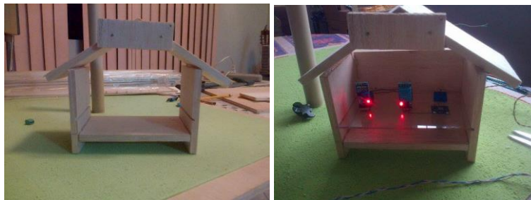
Figura 4.2 Garita Meteorológica con sus respectivos sensores.
