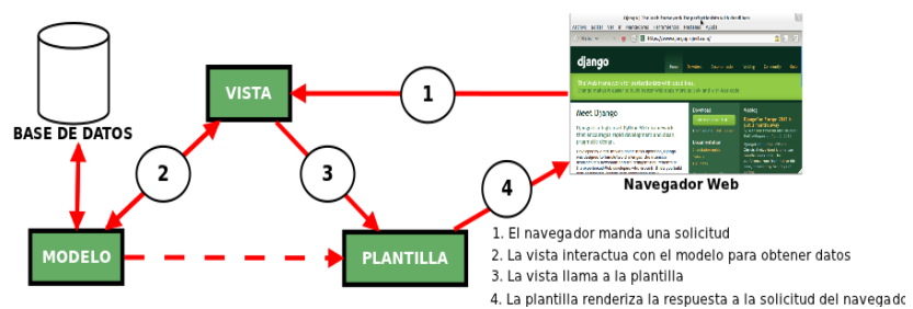
Figura 3.6 El patrón de diseño MVT.
