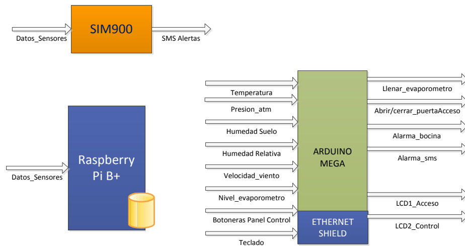
Figura 3.2 Diagrama de bloques de la estación meteorológica.
