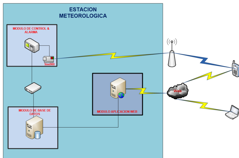
Figura 3.33 Diagrama del sistema con cada uno de sus módulos.
