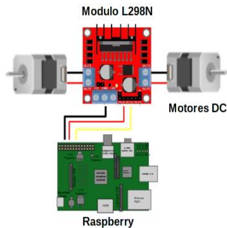
Figura 2.3. Esquema de conexión módulo 298 – raspberry.
