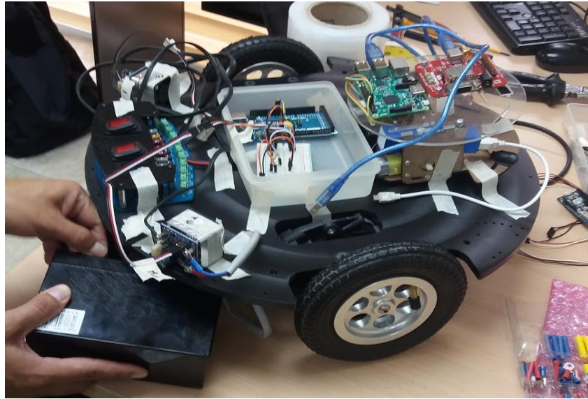
Figura 3.7. Integración de módulo en “Mashi”.
