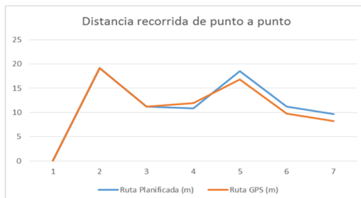
Fig 3.4. Distancia a recorrer vs Distancia recorrida.
