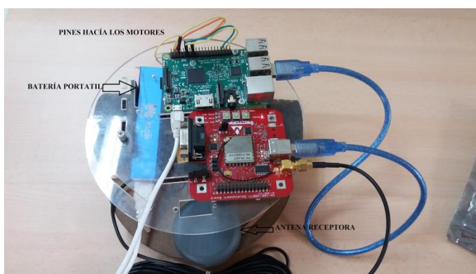
Figura 3.1. Dispositivo embebido y GPS montado en chasis.
