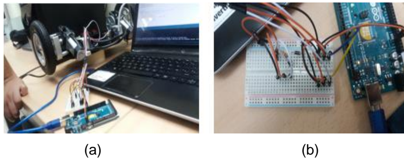
Figura 3.6. (a) Conexión interfaz de comunicación y encoders. (b) Conexión interfaz de comunicación y arduino.
