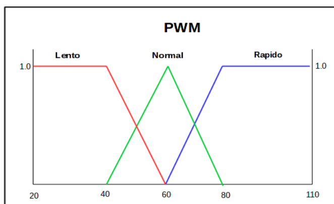
Figura 2.14 Variable de salida que representa el valor de PWM a asignar a cada motor para llevar a cabo el giro correspondiente.
