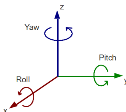
Figura 2.7. Ángulos de navegación.
