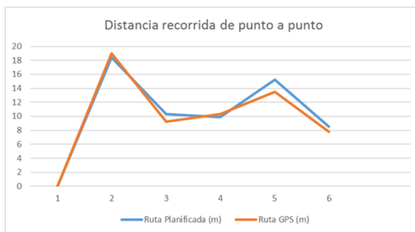
Fig 3.9. Distancia a recorrer vs Distancia recorrida (“Mashi”).
