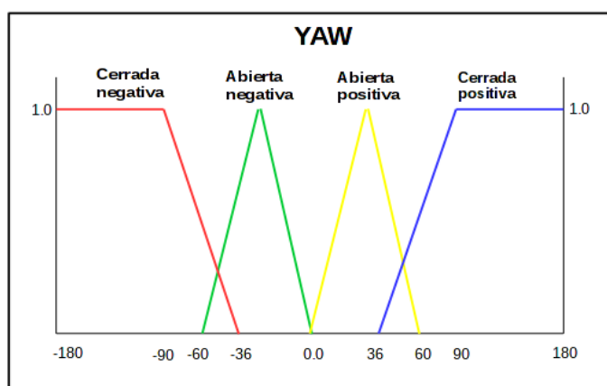
Figura 2.13 Variable de entrada YAW la cual representa los grados del robot hacia su objetivo.
