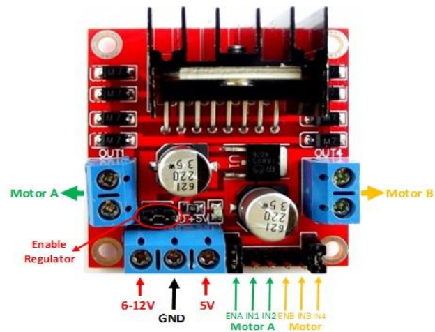
Figura 2.2. Módulo L298N.
