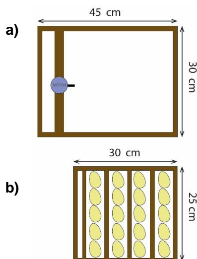
Figura 2.8: Dimensiones de las volteadoras, a) Base
