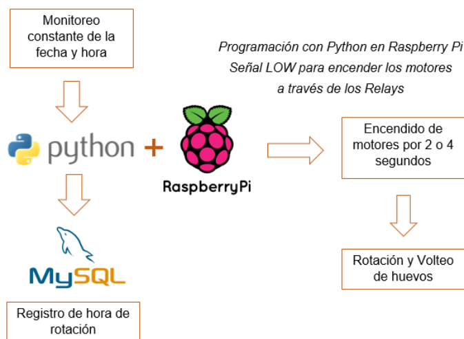
Figura 2.9: Esquema de funcionamiento del Sistema de Rotación y Volteo de Huevos
