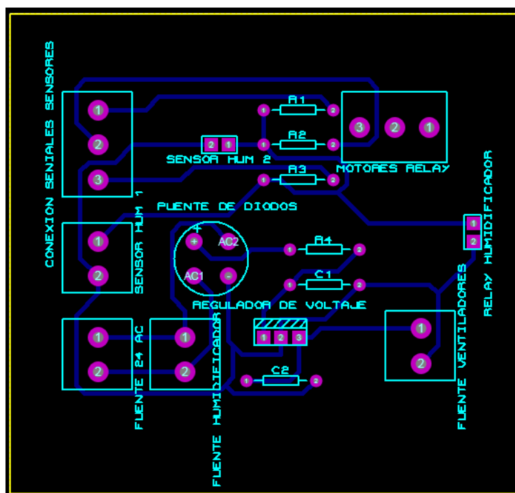
Figura 3.3: Diseño del circuito previo a su impresión
