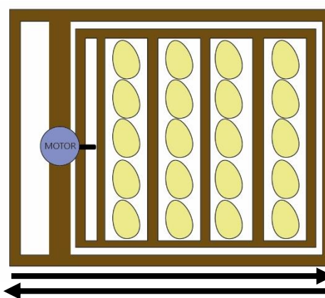
Figura 2.7: Diseño de volteadora con capacidad de 20 huevos, y dirección de movimiento [8]
