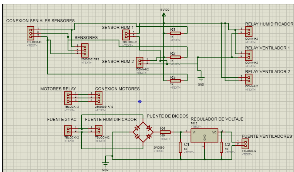
Figura 3.2: Esquemático en Isis del circuito electrónico
