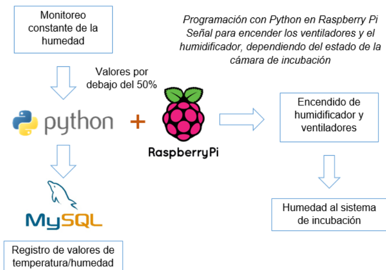
Figura 2.11: Esquema de funcionamiento del Sistema de Generación y Control de humedad
