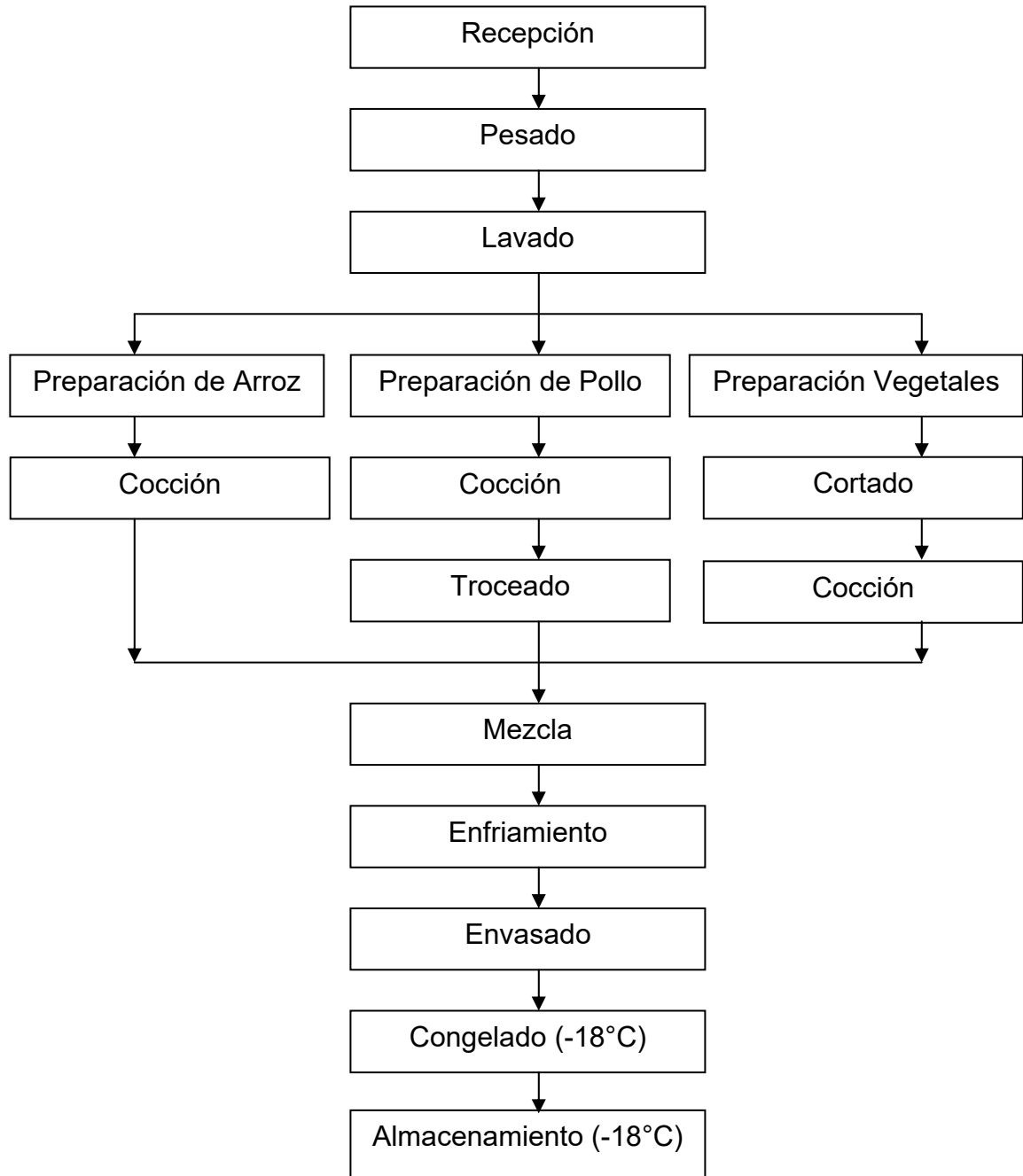
GRÁFICO 3.3 DIAGRAMA DE FLUJO DE ARROZ CON POLLO
