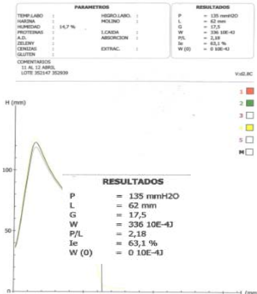
Figura 2.7: Alveogramas
