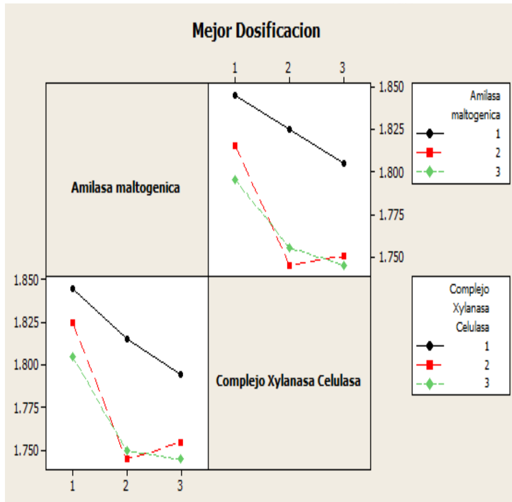
Figura 3.1: Mejor Dosificación
