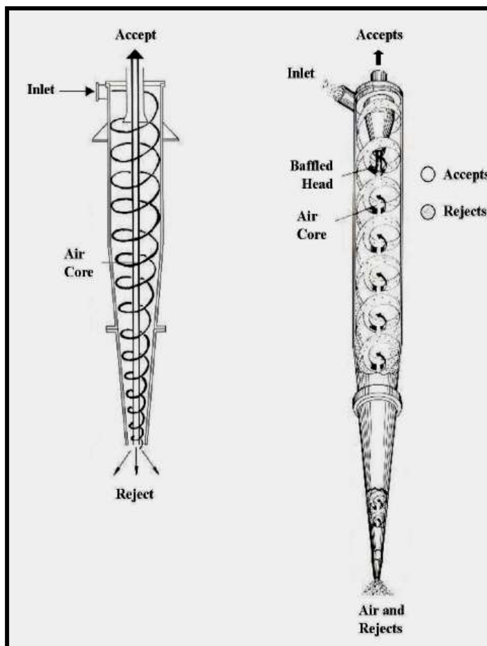
FIGURA 1.12 DEPURADORES CENTRÍFUGOS
