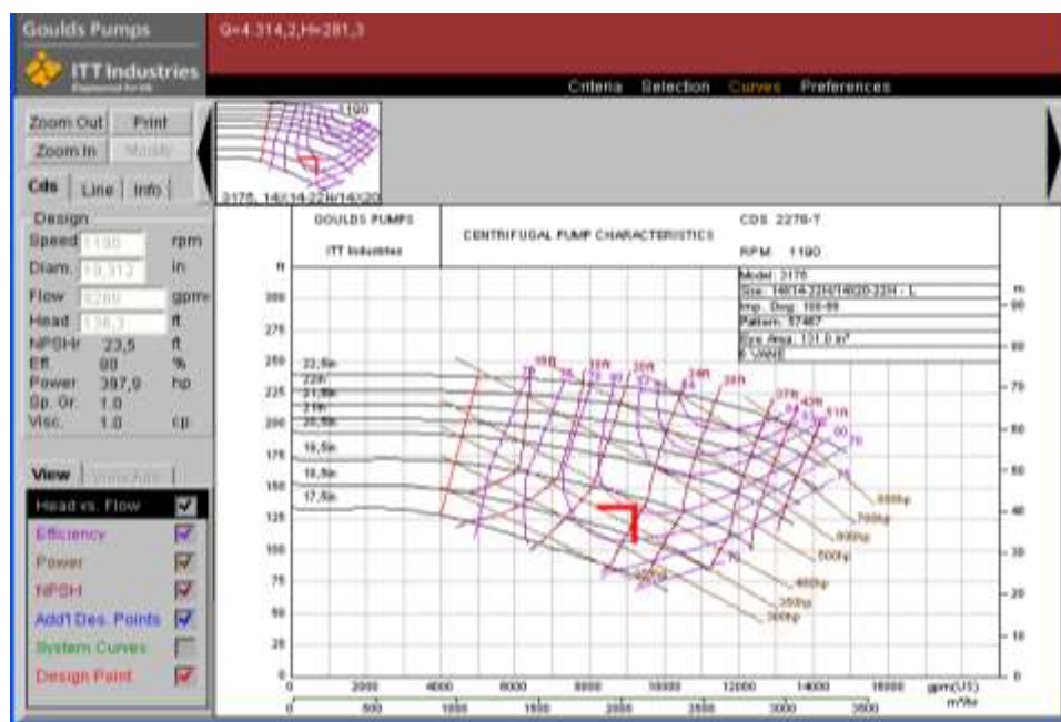
FIGURA 2.21 CURVA DE OPERACIÓN DE BOMBA LIMPIADORES PRIMARIOS UNIFLOW (P15)
