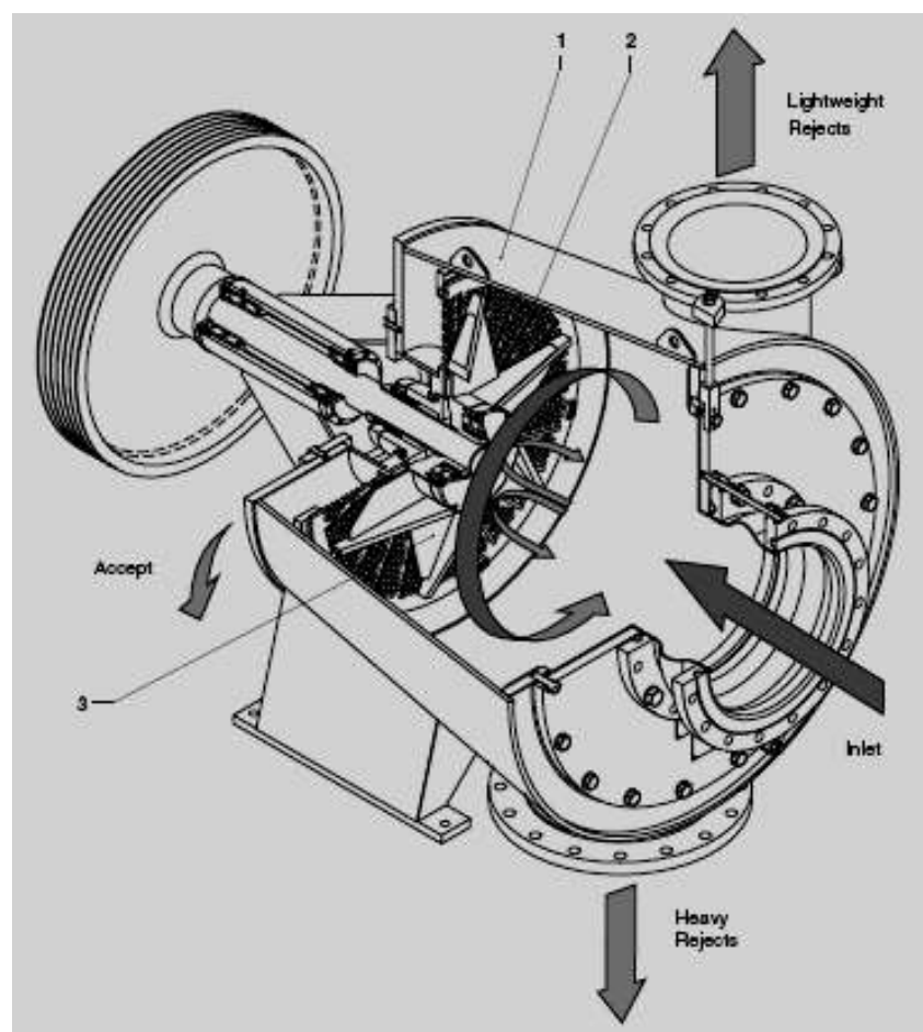
FIGURA 2.2 PRINCIPIO DE OPERACIÓN DEL FIBERIZER
