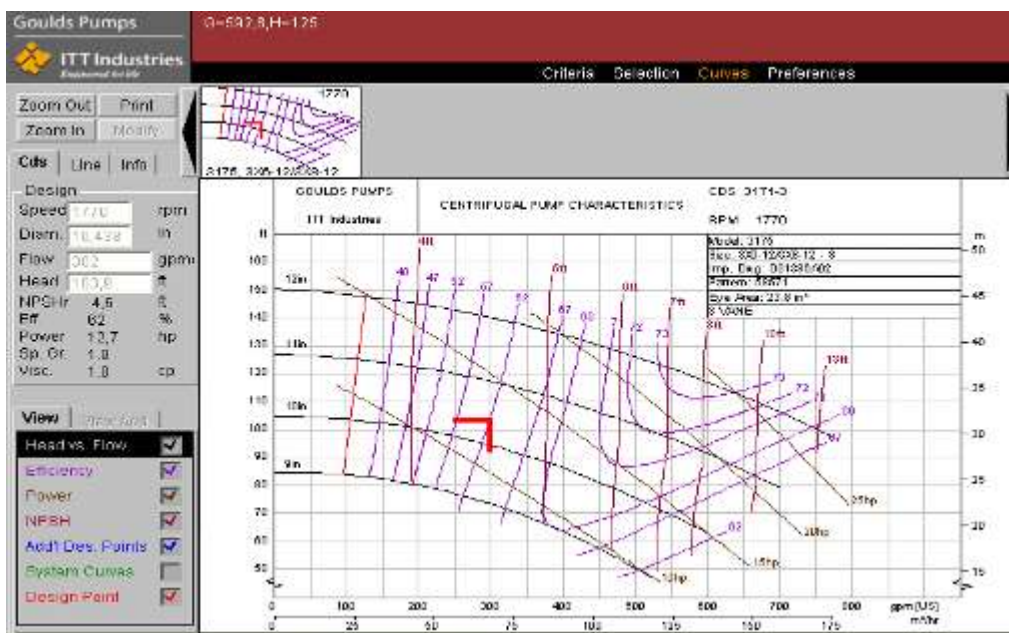
FIGURA 2.23 CURVA DE OPERACIÓN DE BOMBA LIMPIADORES PRIMARIOS UNIFLOW (P13)
