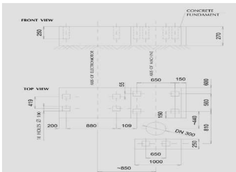
FIGURA 2.11 CIMENTACIÓN DEL PSN-31
