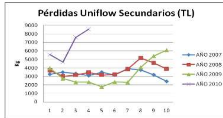
FIGURA 3.26 PÉRDIDAS DE FIBRA UNIFLOW TEST LINER
