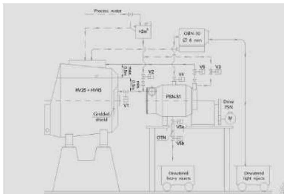
FIGURA 2.10 ESQUEMA DE PROCESO DEL PSN-31
