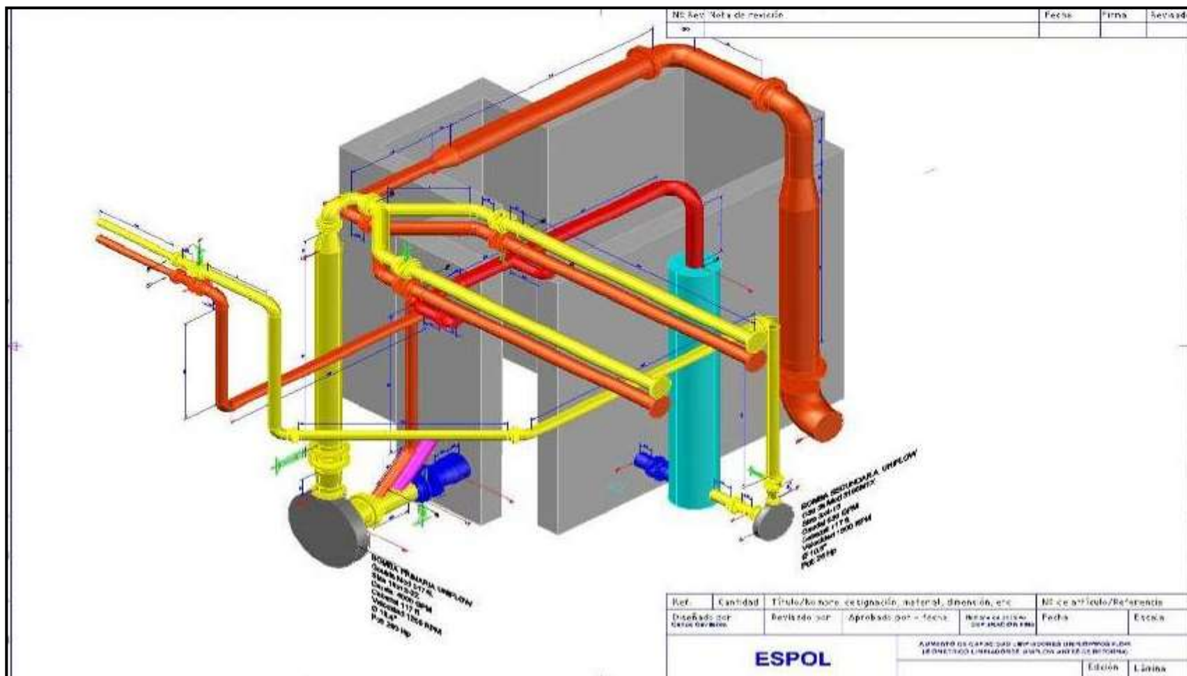
FIGURA 2.17 ESQUEMA DE LIMPIADORES UNIFLOW PREVIO AL PROYECTO
