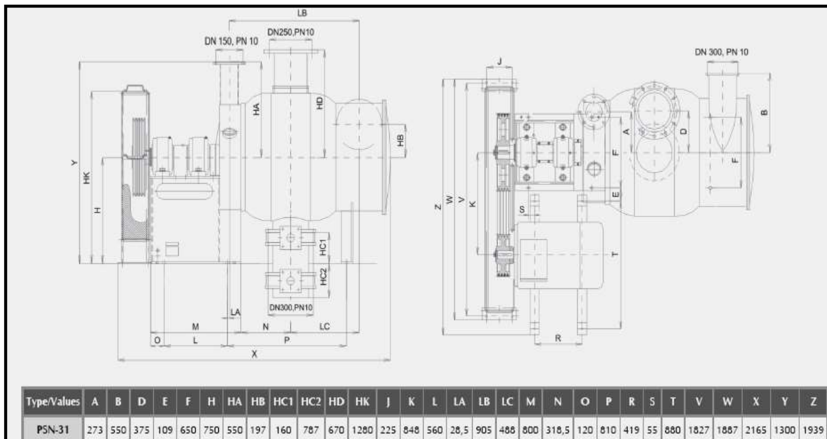
FIGURA 2.6 DIMENSIONES DEL PSN 31
