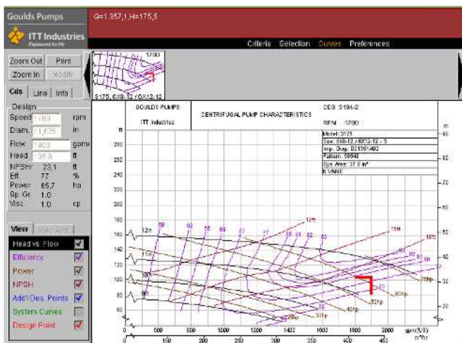
FIGURA 2.22 CURVA DE OPERACIÓN DE BOMBA LIMPIADORES PRIMARIOS UNIFLOW (P16)
