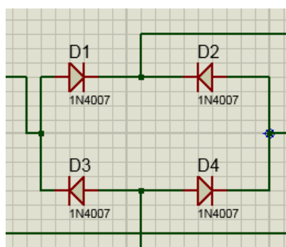
Figura 3.4: Puente Rectificador.
