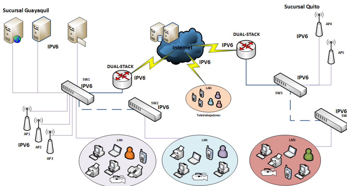
Figura 2.3 Tener IPV6 en el mundo y tener IPV6 en la red local.
