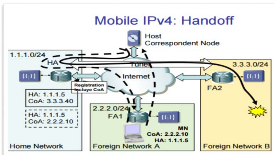
Figura 1.5: Fases de Mobile IPv4 en una red Diferente
