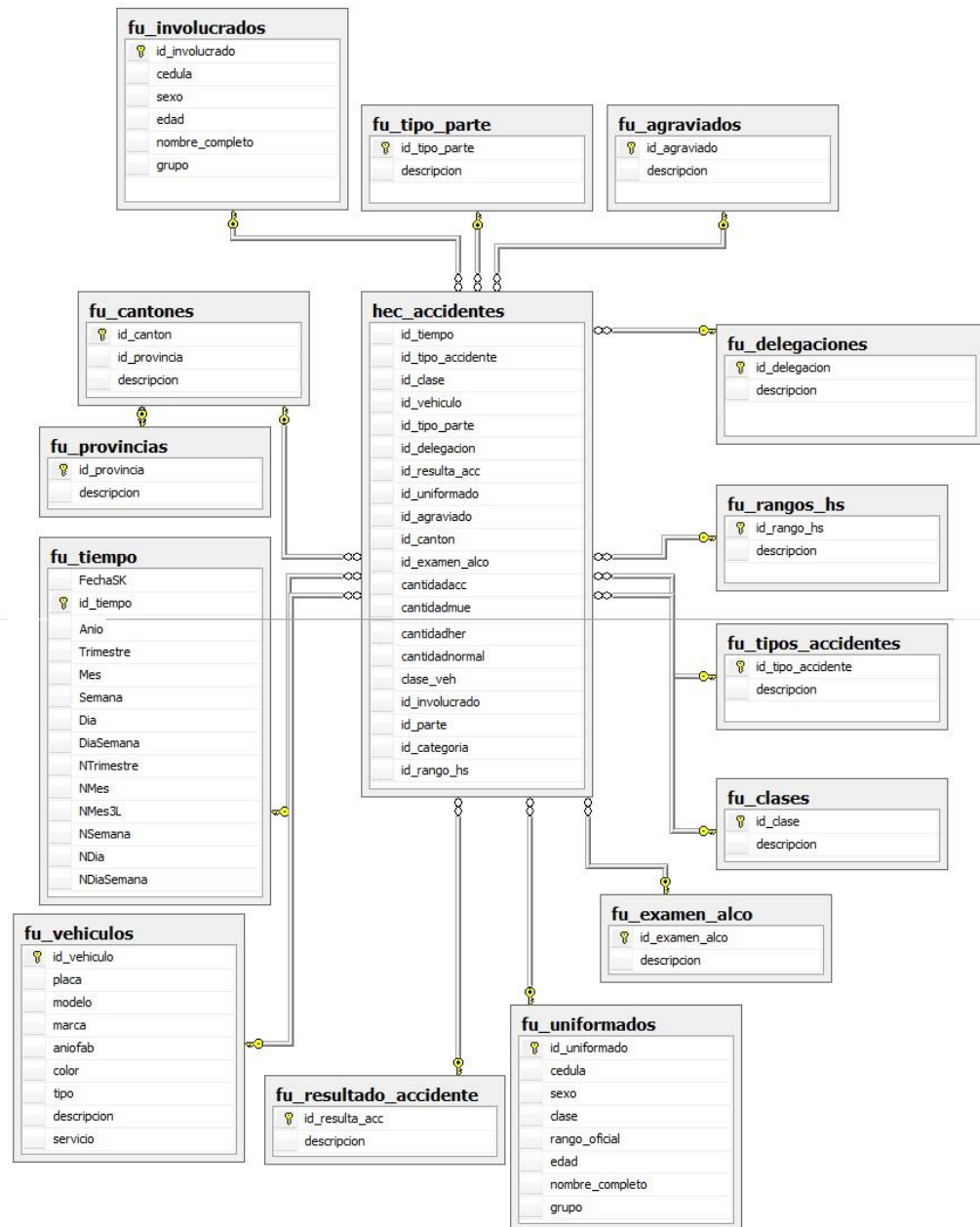
Figura 4.1 Modelo Entidad Relación de Base de Datos Destino
