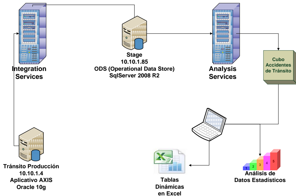
Figura 3.5 Arquitectura para el Datamart de Accidentes de Tránsito CTE
