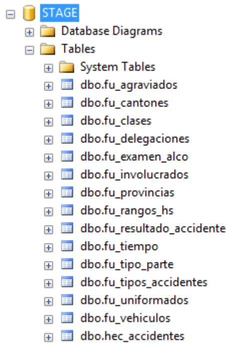
Figura 4.2 Detalle de Tablas de Base de Datos Destino
