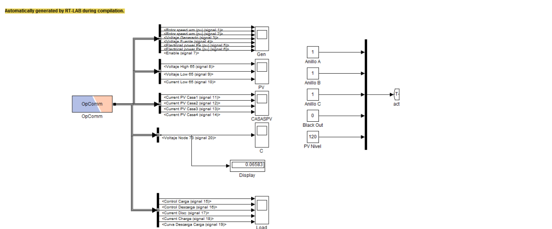
Figura 4.14: Consola de la Microgrid generada por RT-LAB
