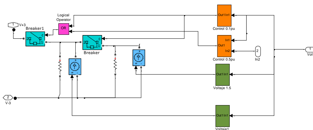
Figura 3.7: Modelo Paneles Fotovoltaicos
