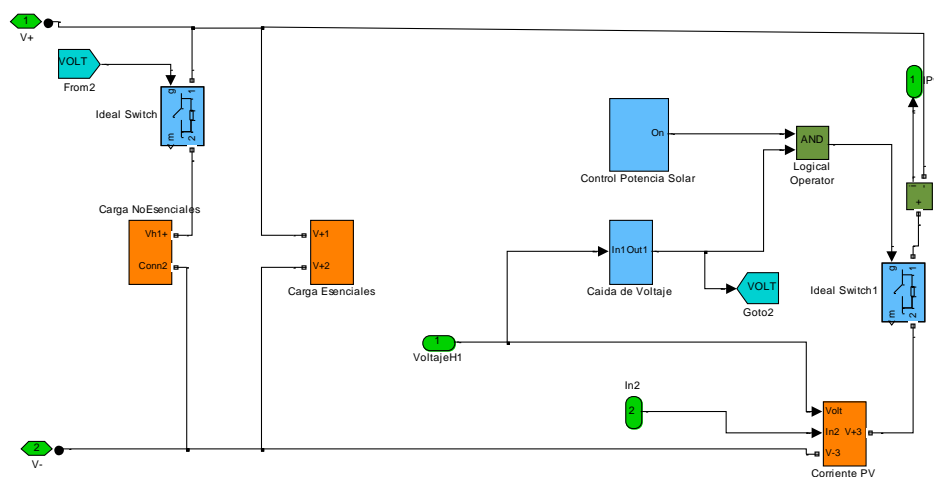
Figura 3.6: Casa modelada en Simulink
