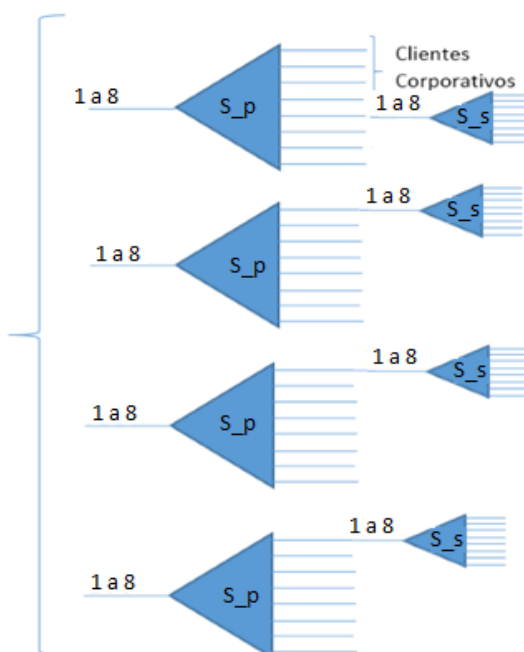
Figura 3.4: Esquema de Splitter Armario 1 – Sinsao
