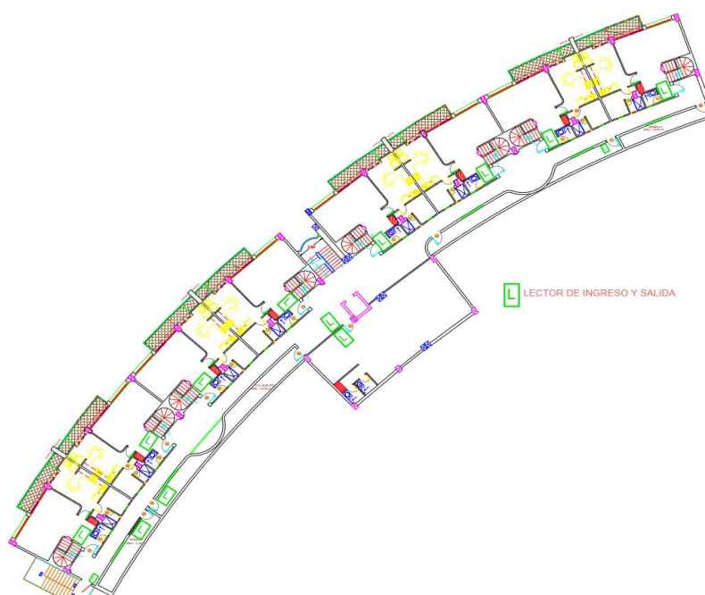
Figura 3.10 Implantación sensores segundo piso
