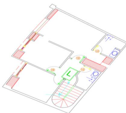
Figura 4.3 Departamento piso 1
