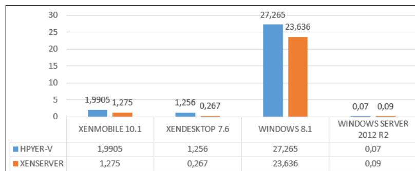
Figura 3.13: Gráfico promedios de uso de procesador con carga de trabajo.
