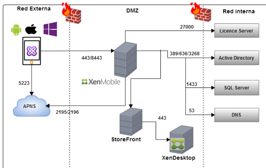
Figura 2.11: Puertos usados en XenMobile y XenDesktop [11].
