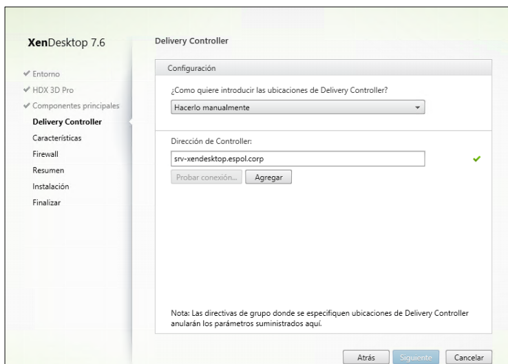
Figura C-8: Configuración de Delivery Controller en Windows 8.1.
