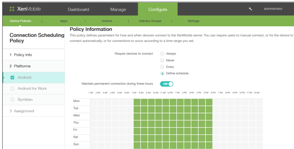
Figura F-24: Configuración de política Scheduling.
