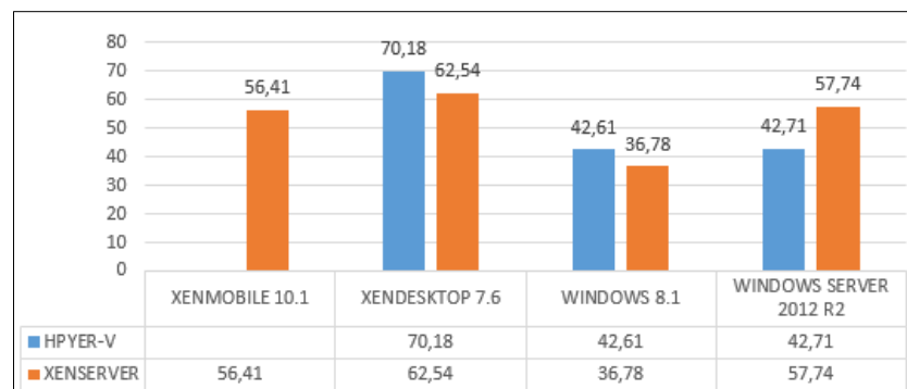
Figura 3.14: Gráfico promedios de uso de memoria RAM sin carga de trabajo.
