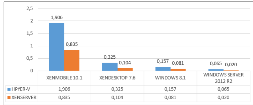
Figura 3.12: Gráfico promedios de uso de procesador sin carga de trabajo.
