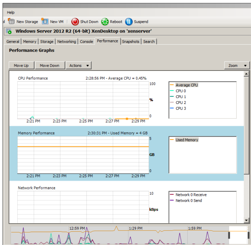
Figura 3.4: Opción Performance en XenCenter.
