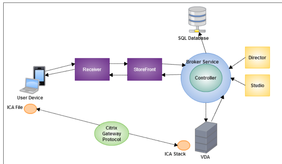
Figura 2.13. Comunicación de XenDesktop y sus componentes [44].
