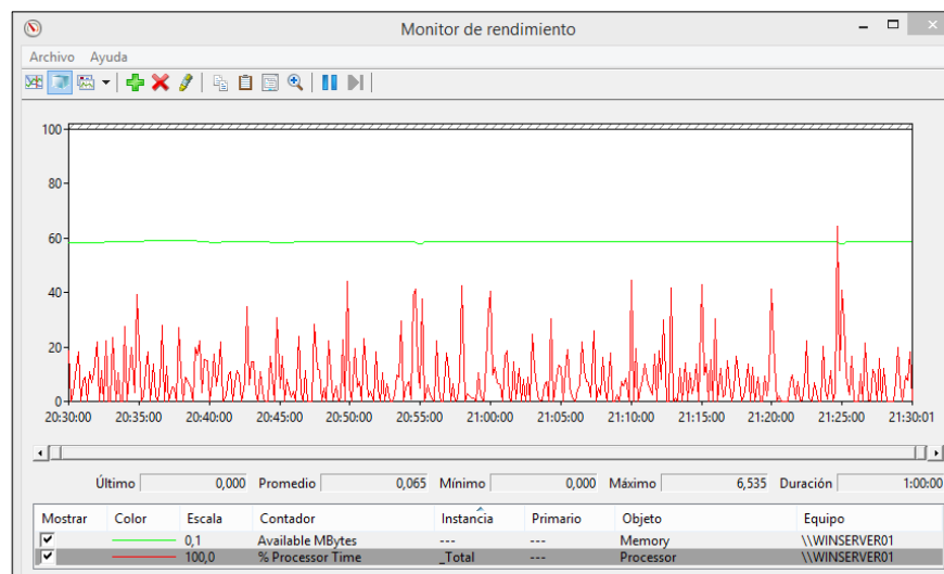
Figura G-2: Windows Server 2012R2 sin carga de trabajo en Hyper-V
