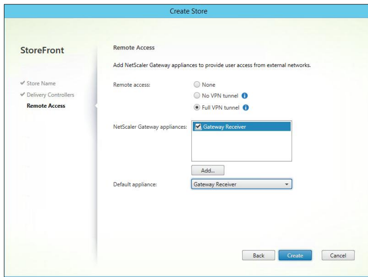
Figura C-13: Configuración de acceso remoto en StoreFront.
