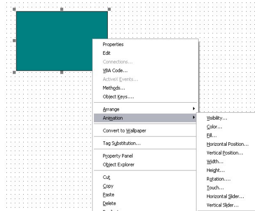
Imagen 3.- Animación de objeto
