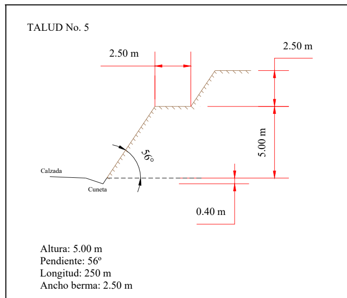
Figura 2.2.5 Talud No. 5
