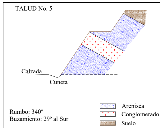
Figura 2.4.5 Perfil Geotécnico, Talud No. 5
