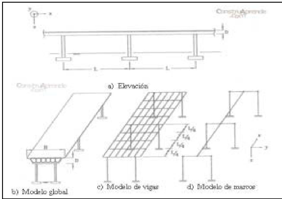
Figura 7. Estructura Básica Puentes
