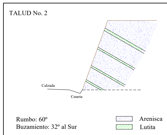
Figura 2.4.2 Perfil Geotécnico, Talud No. 2
