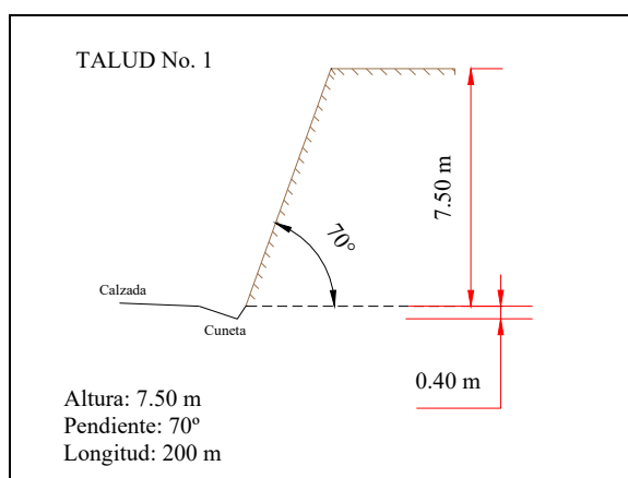
Figura 2.2.1 Talud No. 1.
