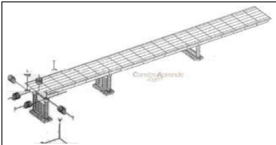
Figura 8. Modelo en SAP de la estructura básica de un Puente
