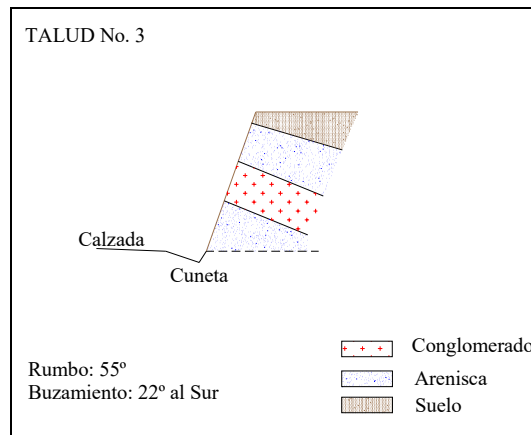
Figura 2.4.3 Perfil Geotécnico, Talud No. 3
