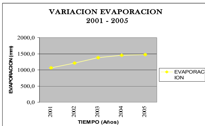
Figura 3.1.3 Variación anual Evaporación (Estación Chongón)
