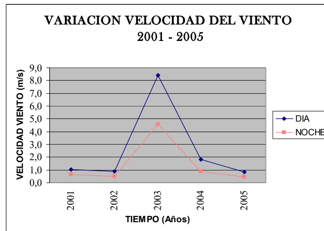
Figura 3.1.2 Variación Anual Velocidad del Viento (Estación Chongón)
