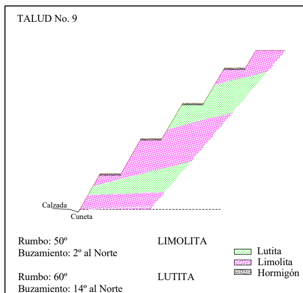
Figura 2.4.9 Perfil Geotécnico, Talud No. 9
