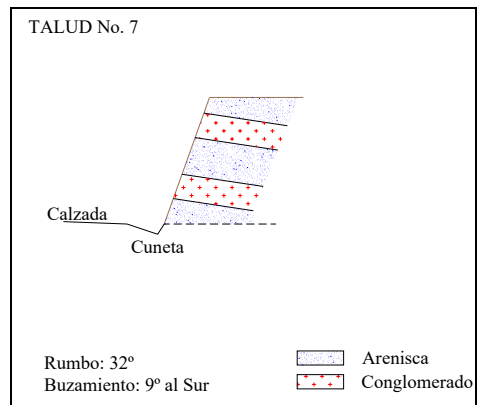
Figura 2.4.7 Perfil Geotécnico, Talud No. 7
