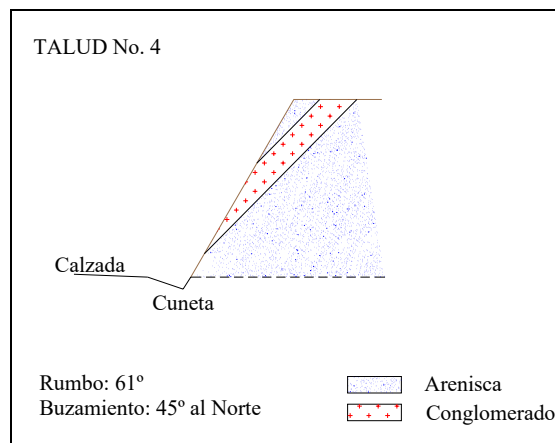
Figura 2.4.4 Perfil Geotécnico, Talud No. 4
