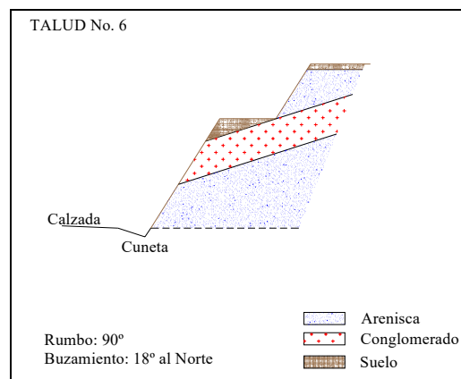
Figura 2.4.6 Perfil Geotécnico, Talud No. 6
