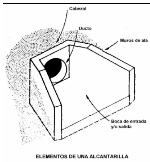
Figura 2.7.1 Elementos de una alcantarilla
