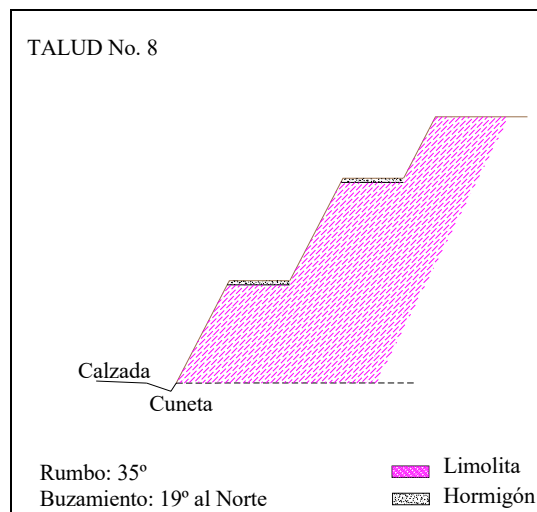
Figura 2.4.8 Perfil Geotécnico, Talud No. 8
