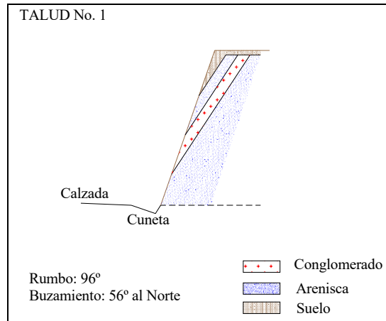
Figura 2.4.1 Perfil Geotécnico, Talud No. 1
