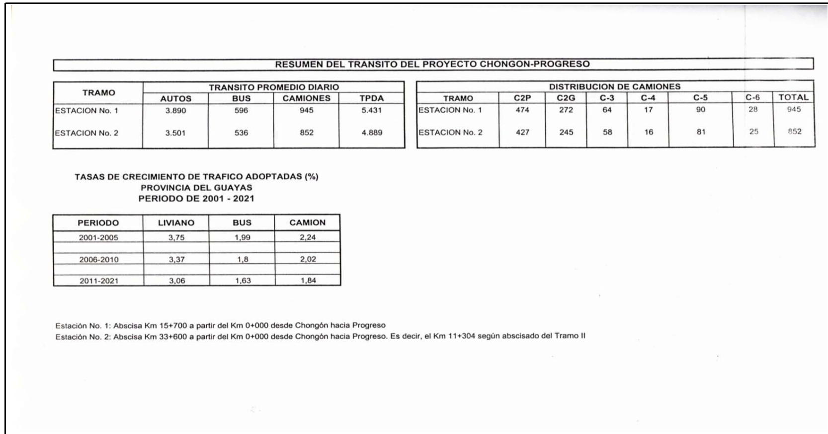
Figura 11. Resumen de Tránsito Vía Chongón - Progreso
