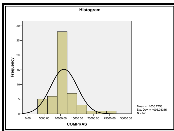
Figura 2.4.2 Histograma-normal (Compras)
