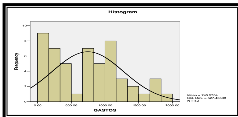
Figura 2.4.3 Histograma-normal (Gastos)
