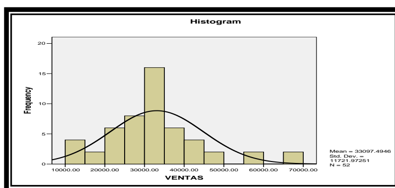
Figura 2.4.1 Histograma-normal (Ventas)
