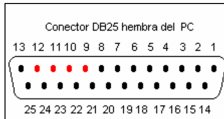
Fig. 40. Numeración de pines del PP.
