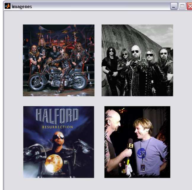
Programa Imágenes.
