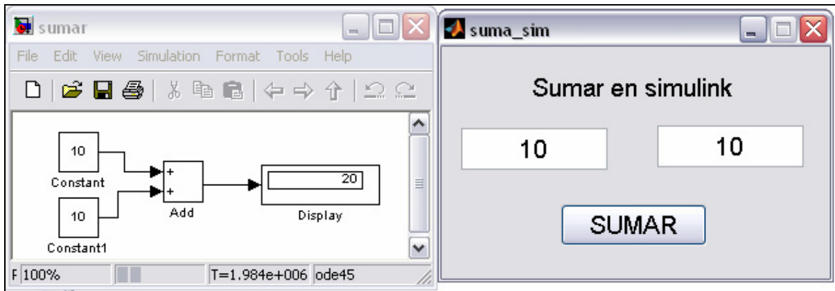
Programa suma_sim .
