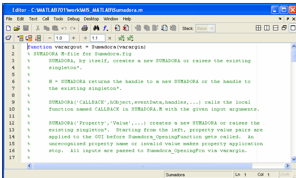
M-file asociado.
