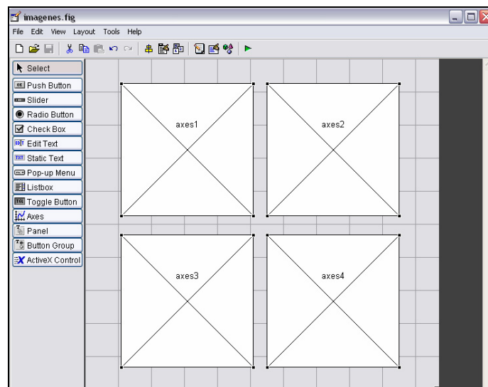
Programa Imágenes.
