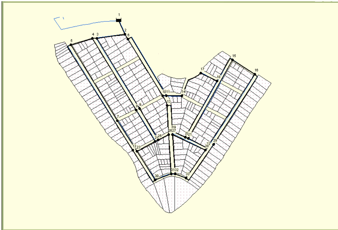
Figura 2.- Plano de la Red, se puede visualizar los nudos de la misma.
