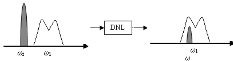
Figura 2.1 Efecto de intermodulación en un dispositivo no lineal (DNL) donde \omega = 2\omega_1 \pm \omega_2 .
