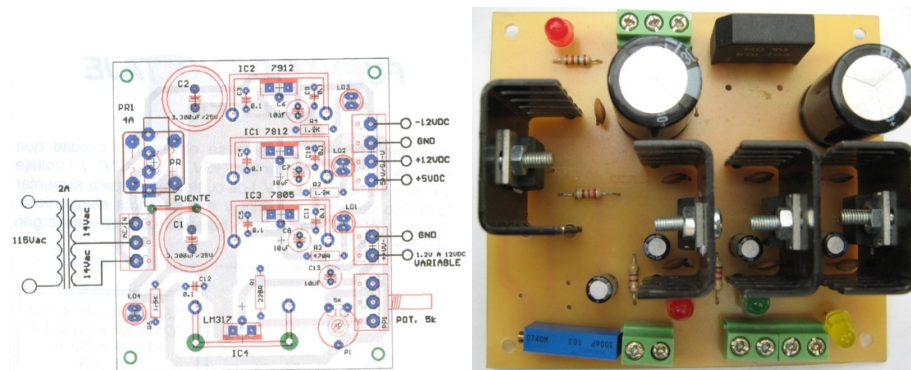
Figura 5.4 Fuente de Voltaje.
