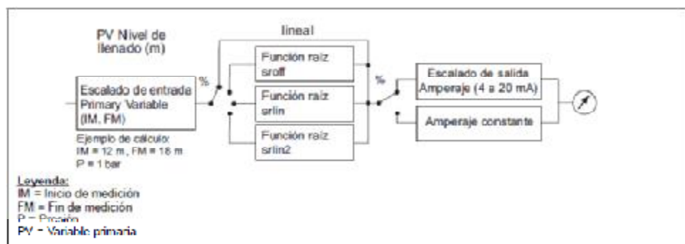
Figura 3.52.- Acondicionamiento de la señal del sensor a señal de corriente 4 – 20 mA.
