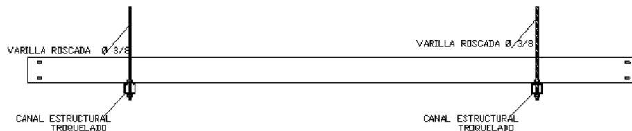
FIGURA B.2 Instalación de bandeja porta-cables
