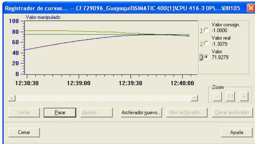
Figura 5.45.- Curvas que muestran la estabilización del controlador PID para el ingreso de amoniaco.
