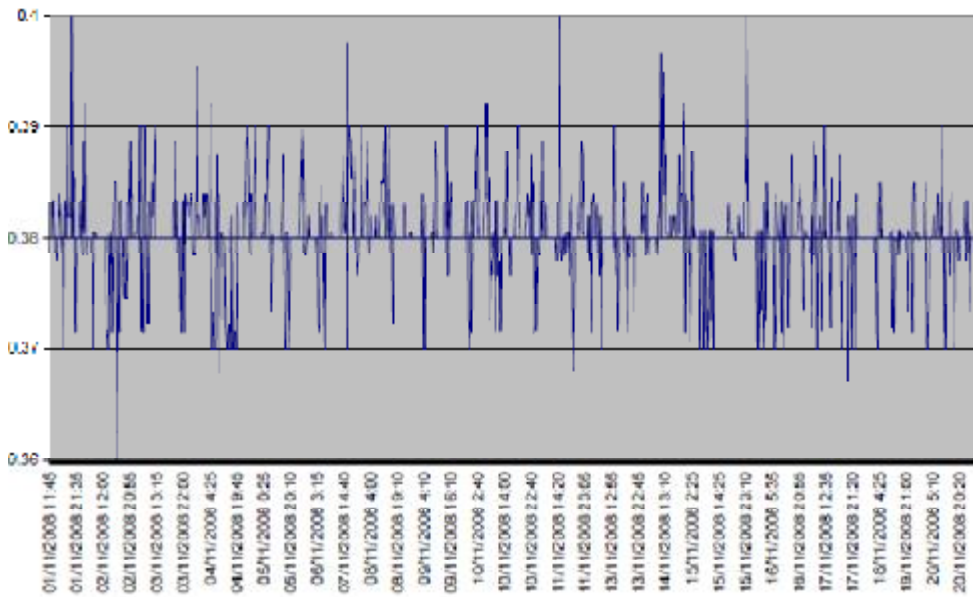
Fig. b.- Desviación producto B – antes de implementado el proceso automatizado
