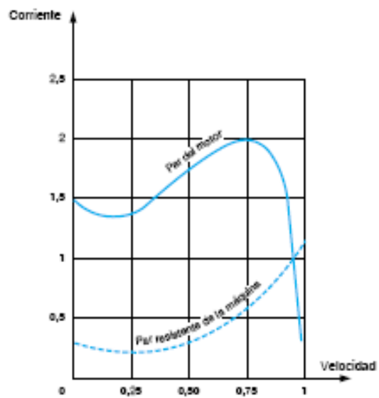
Figura 3.29.- Curva de corriente vs velocidad del arranque directo.
