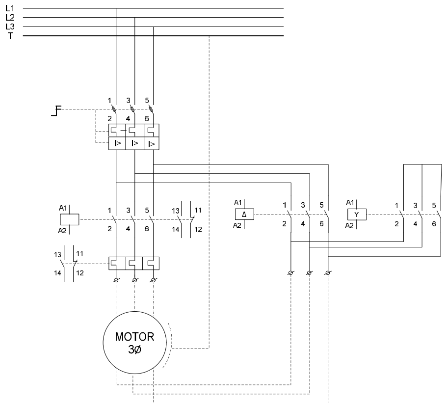
Figura 3.30.- Esquema eléctrico para representar el arranque estrella triángulo de un motor trifásico.
