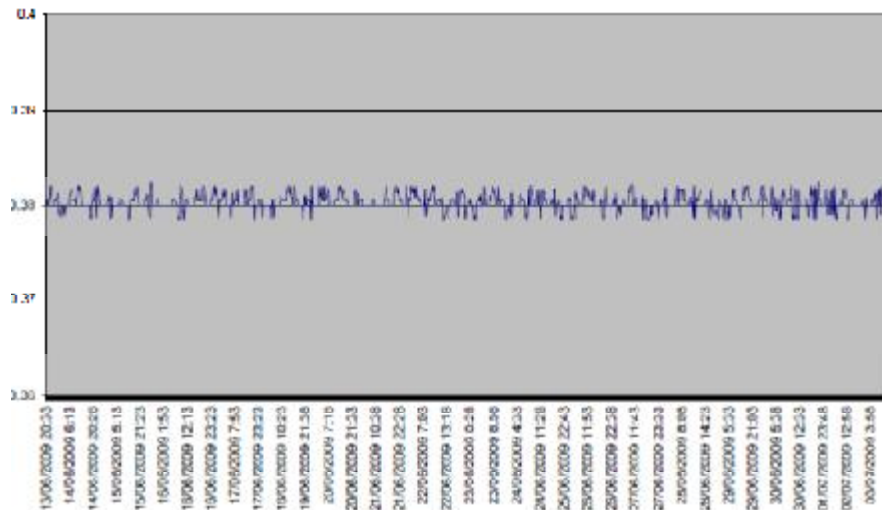
Fig. d.- Desviación producto B – luego de implementado el proceso automatizado
