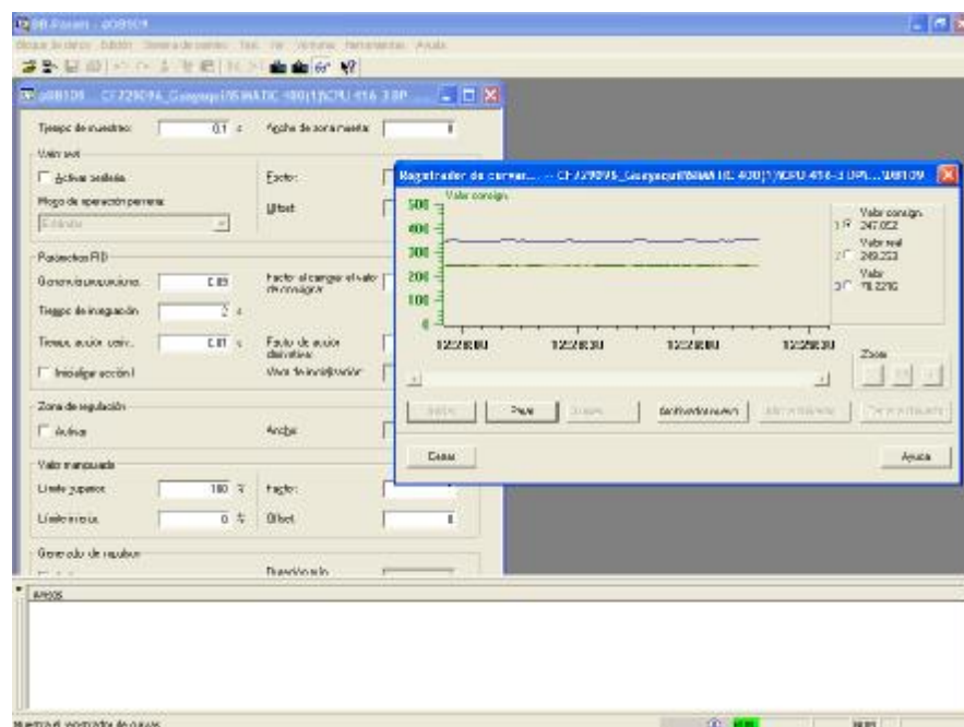
Figura 5.38.- Curvas que muestran la estabilización del controlador y los parámetros de ajuste del controlador PID para la dilución.
