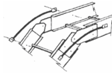
FIGURA 5 Placas de unión vertical regulables
