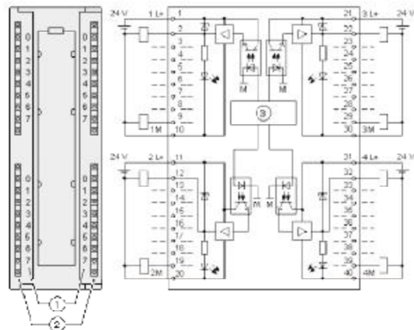
Figura 3.11.- Esquema de conexiones y de principio del modulo de salidas digitales SM 322; DO 32 X DC 24 V.
