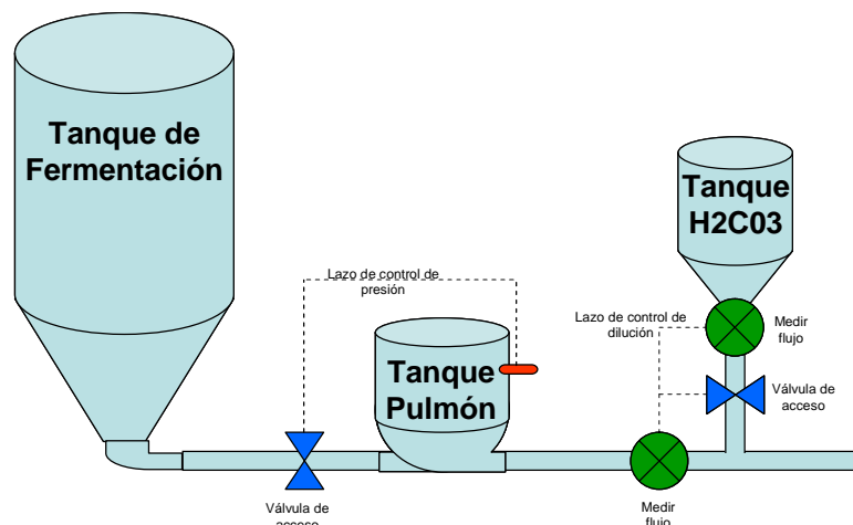
Figura 1.3.- Representación grafica del lazo de control realizado para la dilución de la cerveza.
