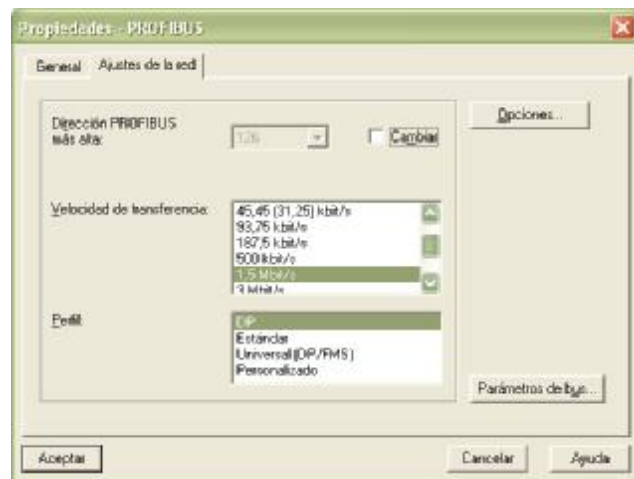
Figura 3.41.- Configuración del puerto PROFIBUS DP de la CPU.
