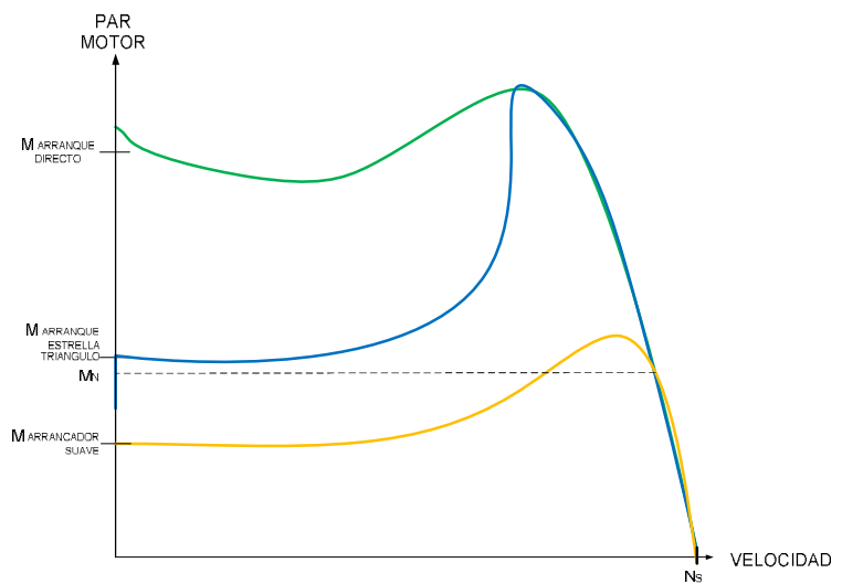
Figura 3.32.- Curva de par motor vs velocidad de un motor con arrancador suave.
