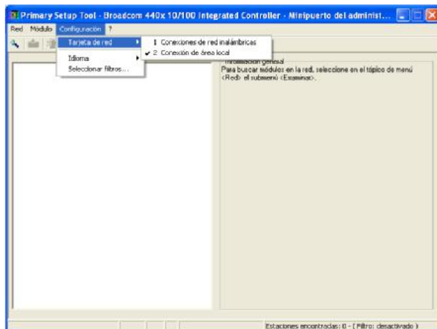
Figura 3.53.- Configuración en software del tipo de red a operar.
