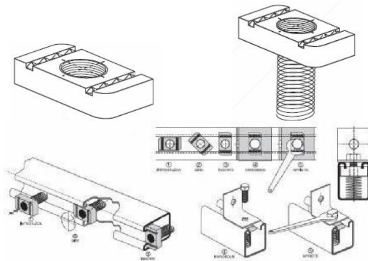
FIGURA A.2 Soporte con canal estructural
