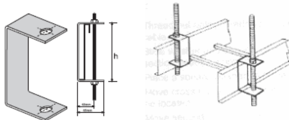
FIGURA A.6 Soporte tipo c simple
