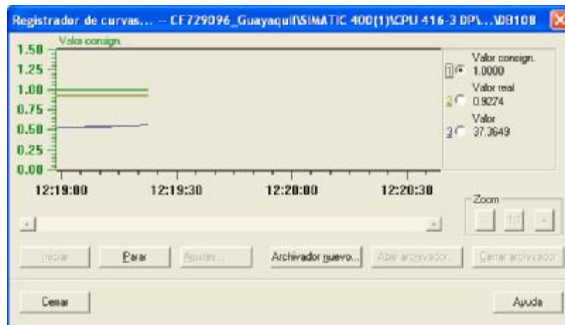
Figura 5.32.- Curvas que muestran el funcionamiento del controlador, el valor de consigna o set point, la variable de proceso o valor real y el valor de salida del controlador.
