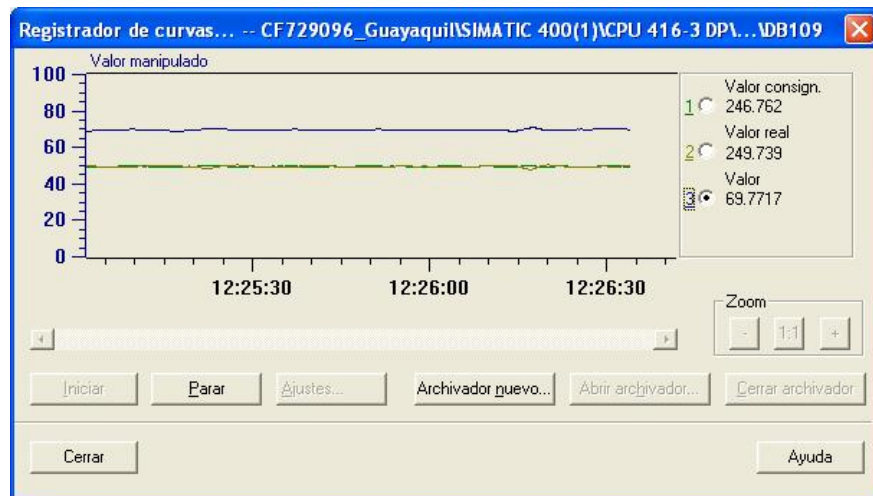
Figura 5.37.- Curvas que muestran la estabilización del controlador PID para la dilución.
