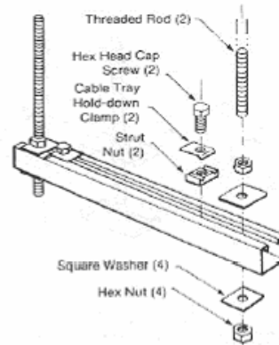
FIGURA A.4 Despiece del soporte con canal estructural
