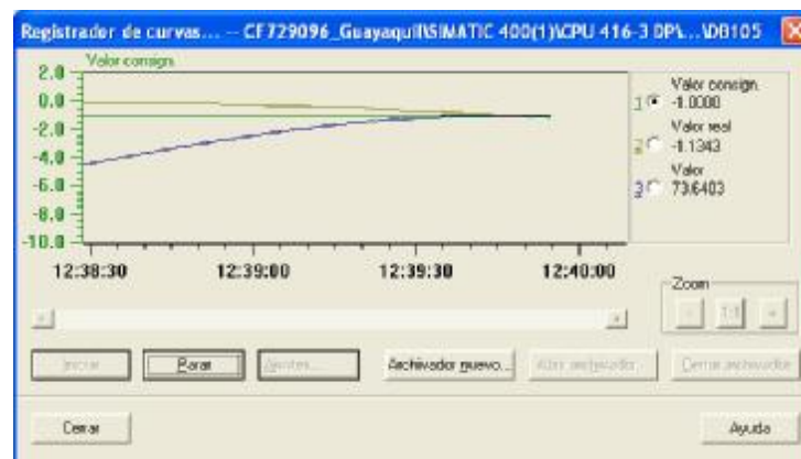
Figura 5.44.- Funcionamiento del controlador PID, el valor de consigna o set point, la variable de proceso y el valor de salida.
