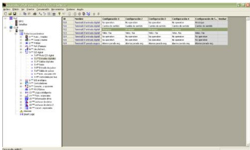
Figura 3.65.- Configuración de la entrada digital de RUN para el DRIVE.
