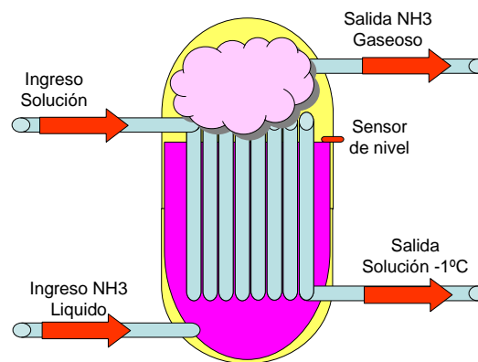
Figura 1.5.- Esquema de funcionamiento de un sistema inundado de enfriamiento.
