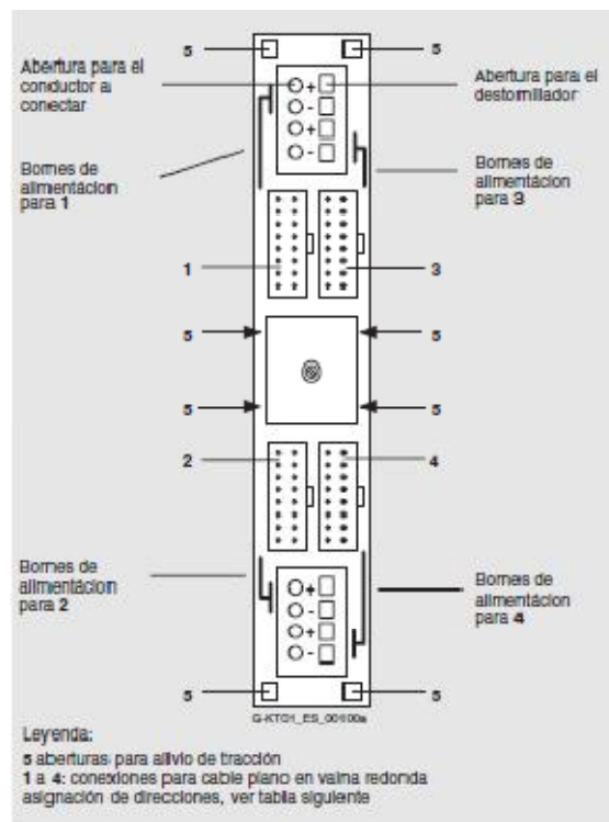
Figura 3.16.- Modulo de conexión frontal 6ES7-921-3AA20-0AA0 de SIEMENS.
