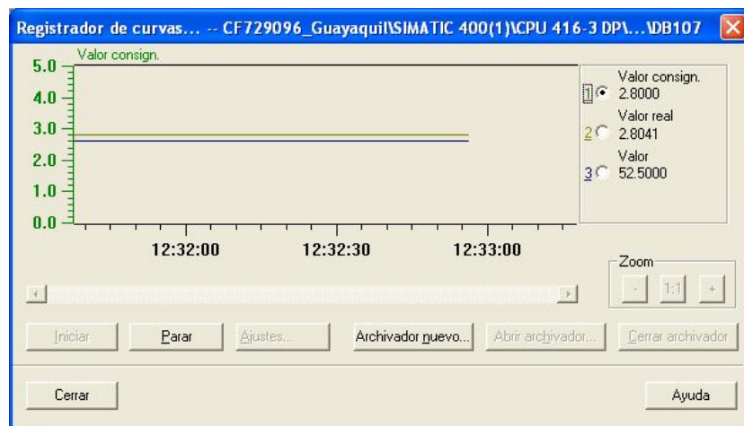
Figura 5.40.- Las curvas que muestran el funcionamiento del controlador, el valor de consigna o set point, la variable de proceso o valor real y el valor de salida del controlador.
