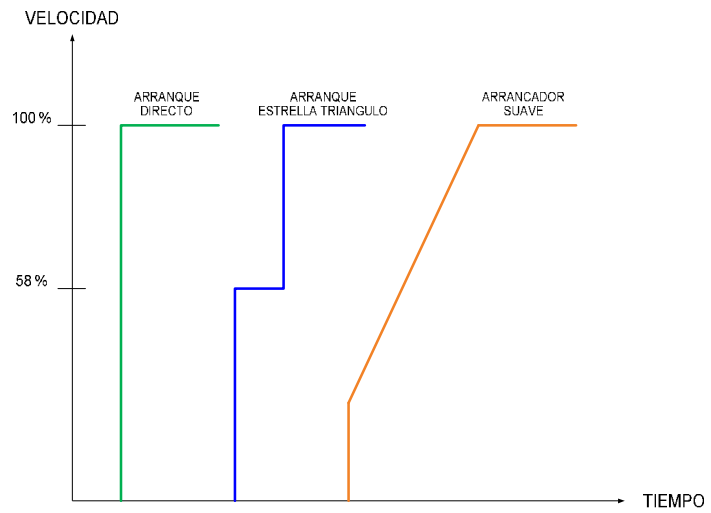
Figura 3.31.- Curva de velocidad vs tiempo de un motor con arrancador suave.
