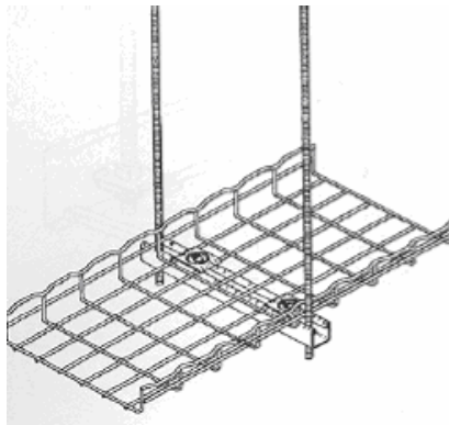
FIGURA A.5 Soporte colgante
