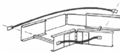
FIGURA 3 Placas de unión horizontal regulables
