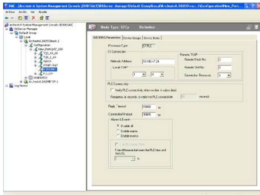
Figura 5.15.- Ventana de Configuración de parámetros del SIDirect.
