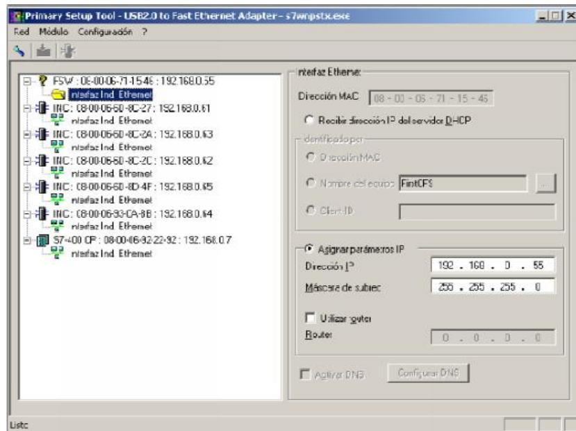
Figura 3.56.- Introducción de la nueva dirección IP del switch XCALANCE X 212-2.
