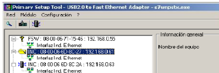
Figura 3.57.- Carga de la configuración al hardware de comunicación.
