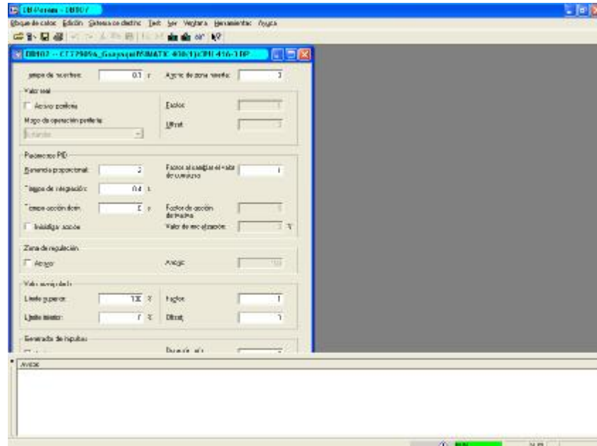
Figura 5.39.- Se observan los parámetros del controlador PID, K_p=2 , T_i=0.4 Seg, T_d=0 Seg.
