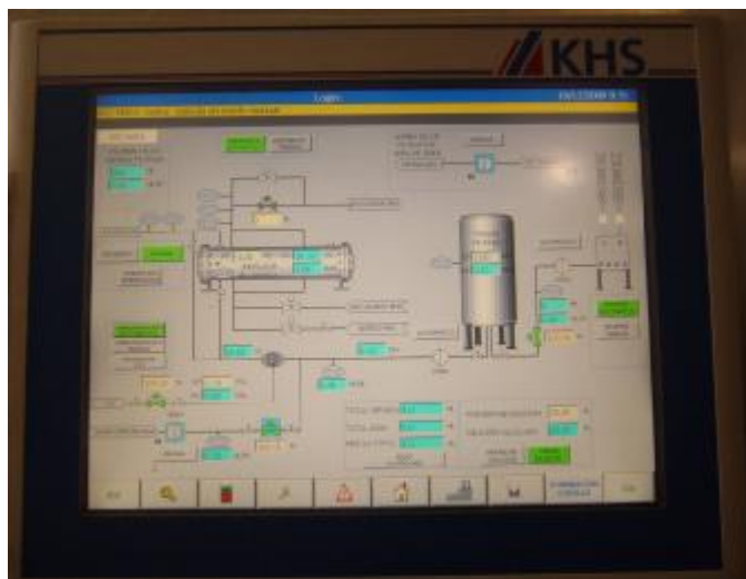
Figura 2.8.- Pantalla HMI Interacción Hombre Maquina.
