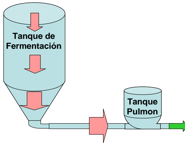
Figura 1.1.- Representación grafica del principio de funcionamiento de tanque Pfuffer.
