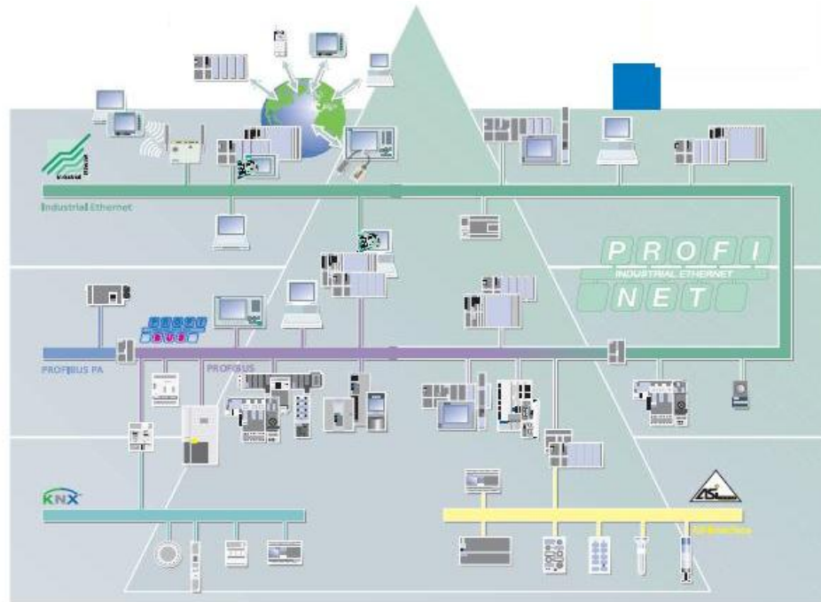
Figura 3.1.- Grafica representativa de los niveles de automatización disponibles con la plataforma SIEMENS
