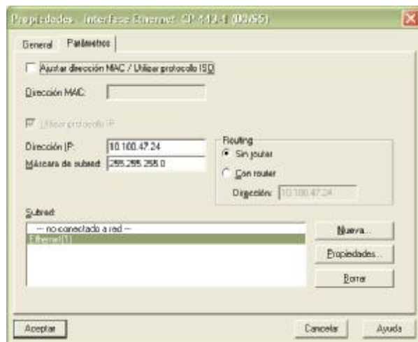
Figura 3.43.- Configuración de la tarjeta Ethernet de la CPU S7-400.
