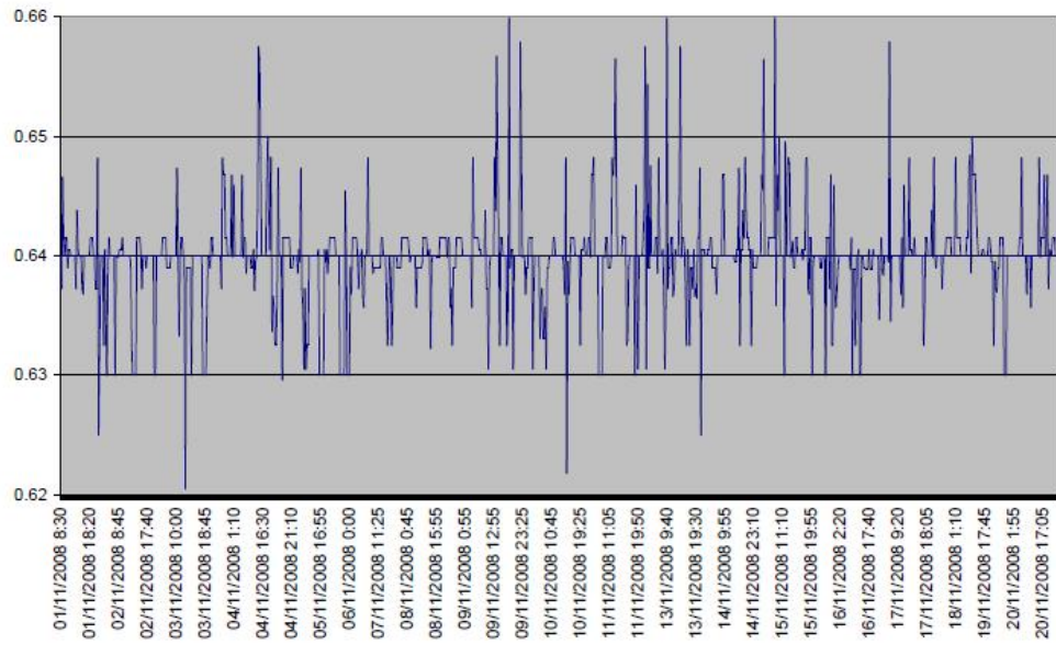
Fig. a.- Desviación producto A – antes de implementado el proceso automatizado
