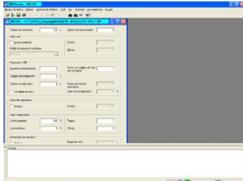
Figura 5.31.- Se observan los parámetros del controlador PID, K_p=3 , T_i=2 Seg, T_d=0 Seg.
