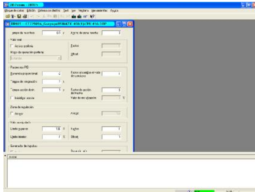
Figura 5.43.- Se observan los parámetros del controlador PID, K_p=-2 , T_i=3 Seg, T_d=1 Seg.
