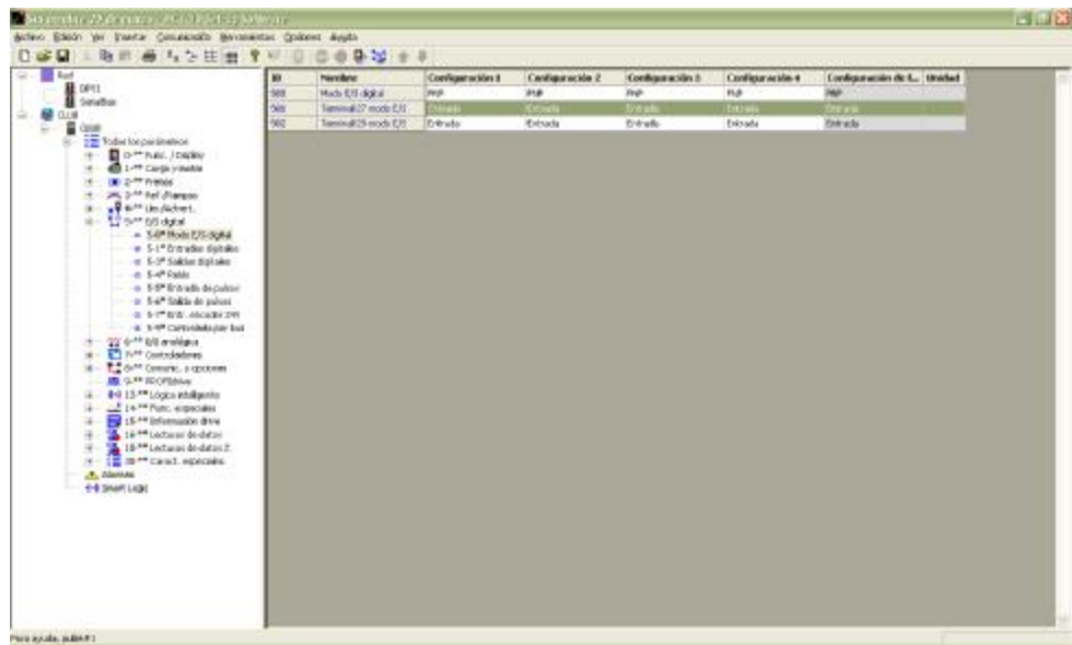
Figura 3.64.- Configuración de las entradas digitales.
