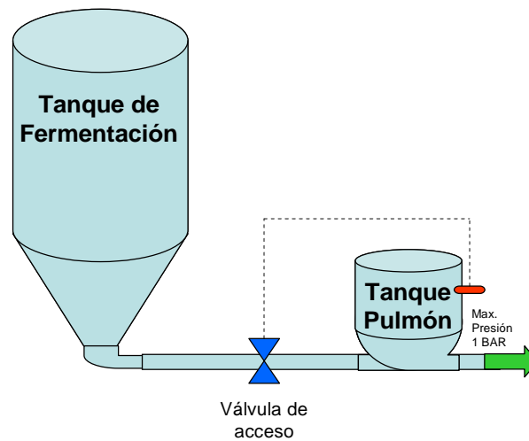
Figura 1.2.- Representación grafica del lazo de control realizado sobre el tanque Puffer.
