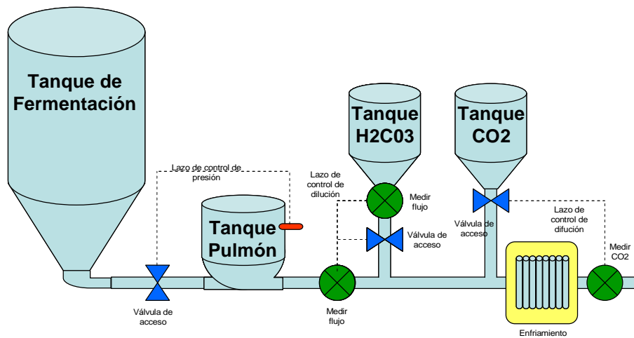
Figura 1.4.- Representación grafica del lazo de control para el proceso de inyección de CO 2 al sistema.
