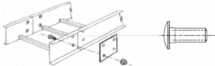
FIGURA B.4 Sujeción de la placa de expansión
