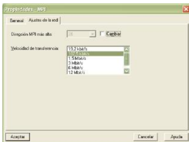
Figura 3.42.- Configuración del puerto MPI de la CPU.
