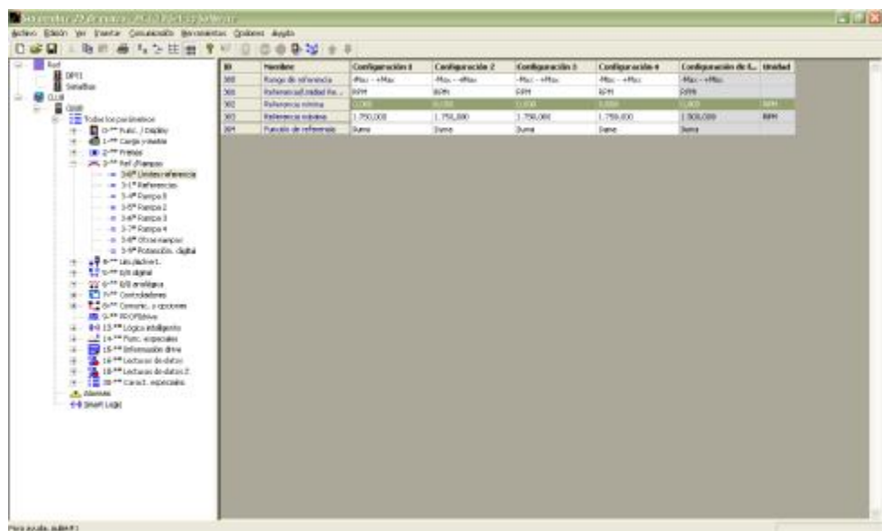
Figura 3.69.- Configuración de la referencia máxima y mínima de la velocidad del motor.
