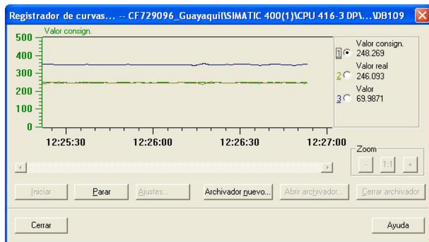
Figura 5.36.- Funcionamiento del controlador PID, el valor de consigna o set point, la variable de proceso y el valor de salida.
