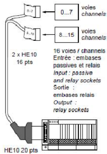
Figura 3.22.- Cable de conexión de 16 canales 2 x HE 10 16 puntos, con dos conectores uno para cada 8 canales.
