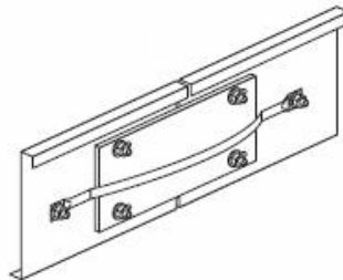
FIGURA B.5 Instalación de las placas de expansión
