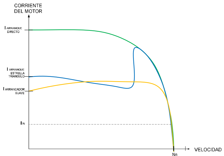
Figura 3.33.- Curva de par motor vs velocidad de un motor con arrancador suave.
