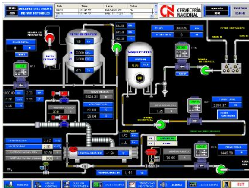
Figura 5.18.- Pantalla de visualización general del proceso de dilución de cerveza (SCADA).
