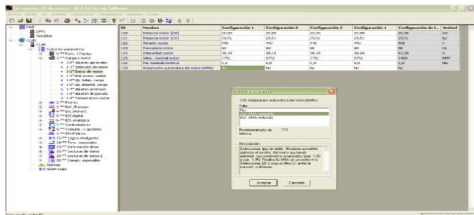
Figura 3.68.- Configuración de la Adaptación Automática del Motor del DRIVE.
