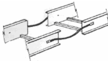
FIGURA 4 Unión discontinua
