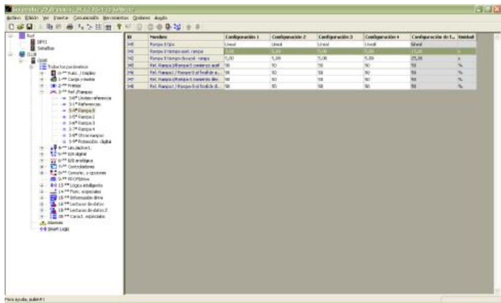
Figura 3.70.- Ajuste de rampas de aceleración y desaceleración.
