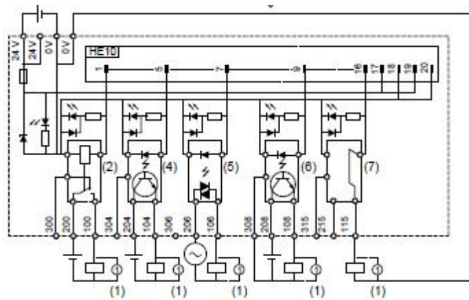
Figura 3.26.- Esquema de conexiones y de principio del modulo de salida digital TELEFAST 16 relay OUT ABE7R16T330.
