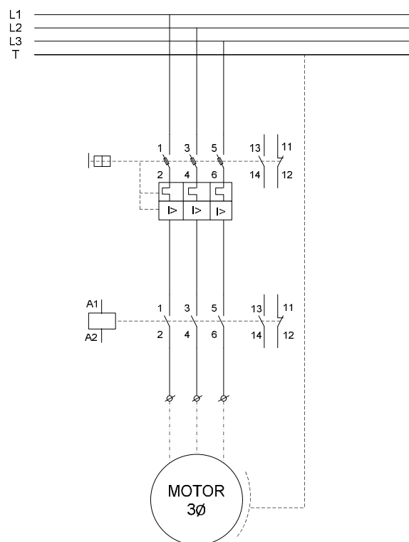
Figura 3.27.- Esquema eléctrico para representar el arranque directo de un motor trifásico.
