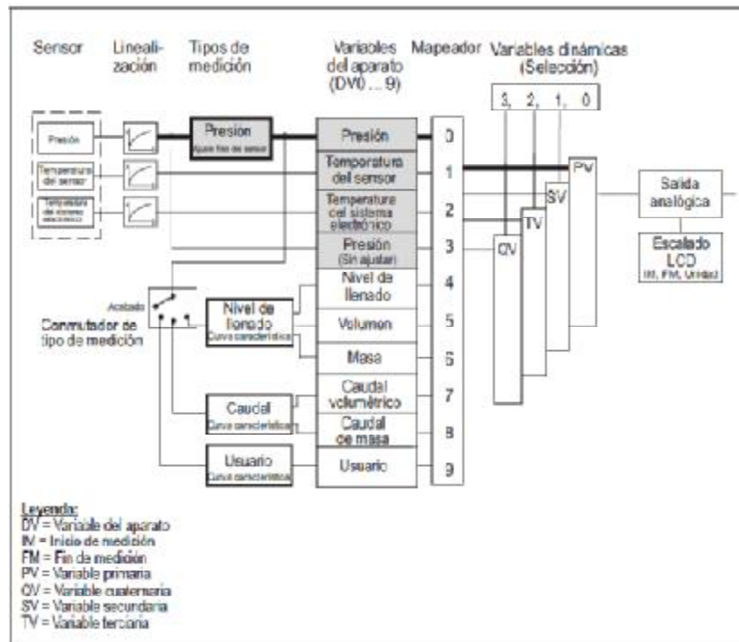
Figura 3.51.- Diagrama de bloques que representa los pasos para la configuración del instrumento.
