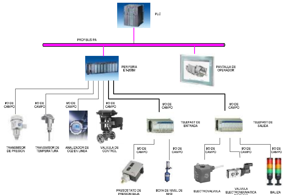
Figura 3.2.- Arquitectura de control implementada.
