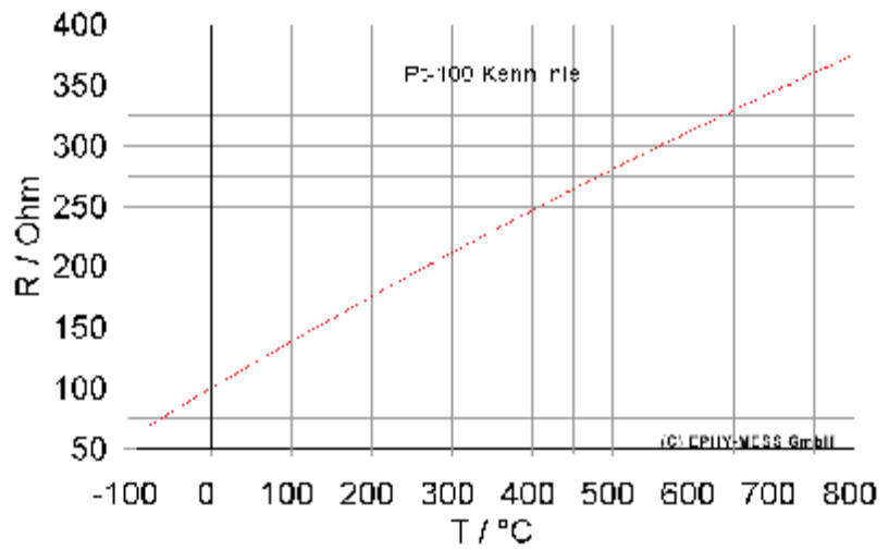
Figura 2.12.- Relación Resistencia Vs Temperatura.
