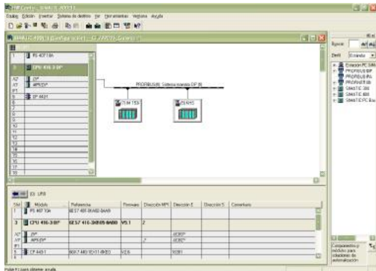
Figura 3.40.- Declaracion de la configuracion de hardware.
