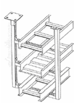
FIGURA A.3 Instalación típica de un soporte con canal estructural
