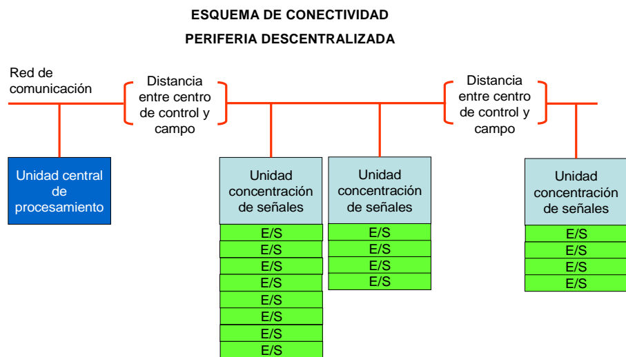
Figura 2.7.- Esquema de conectividad Periferia descentralizada.
