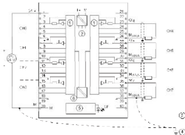
Figura 3.15.- Esquema de conexiones y de principio del modulo de salida analógica SM 332; AO 8 X 12 BIT.
