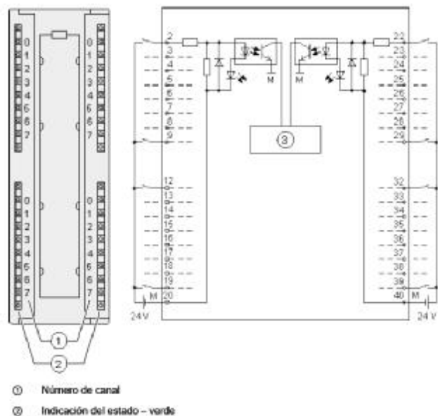
Figura 3.9.- Esquema de conexiones y de principio del modulo de entradas digitales SM 321; DI 32 X DC 24 V.
