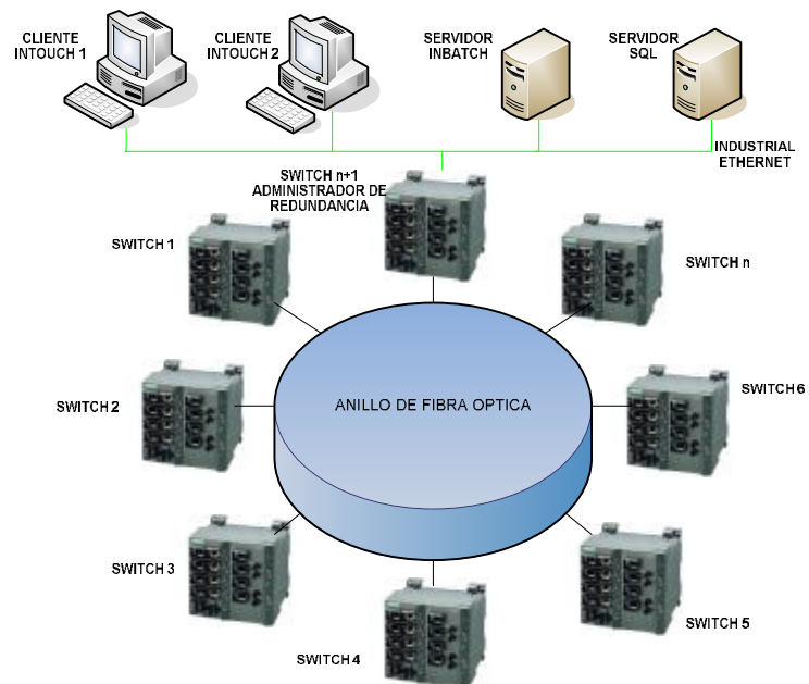
Figura 3.35.- Topología de red industrial Ethernet y de una anillo de fibra óptica.
