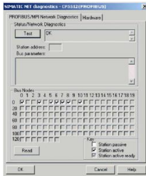
Figura 5.11.- Resultado del diagnóstico de la red.
