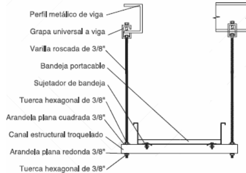
FIGURA A.2 Soporte con canal estructural
