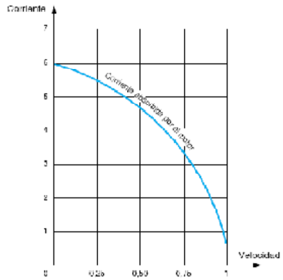
Figura 3.28.- Curva de corriente vs velocidad del arranque directo.
