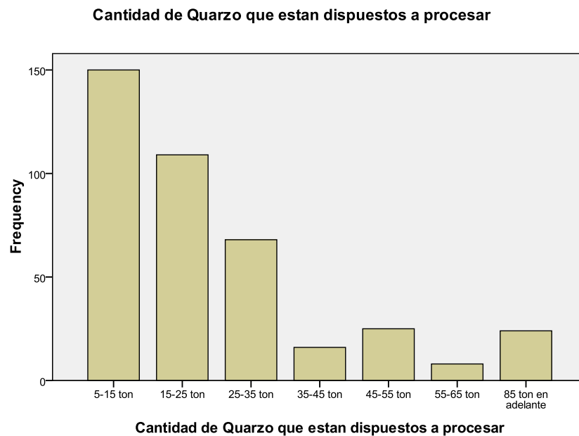
Ilustración 1: Histogramas - Preg 1
