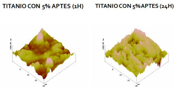
Figura 9. Imágenes de Titanio con 5% APTES 1 hora y 24 horas, obtenidas por AFM
