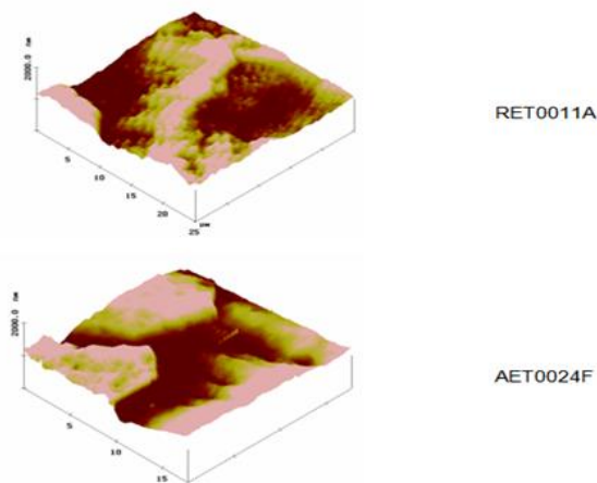
Figura 5. Imágenes de superficie modificada en solución con AEMA (AET0024-F) y en solución sin AEMA (RET0011-A) obtenidas por microscopía de fuerza atómica.
