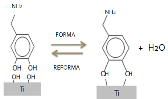
Figura 2. Mecanismo de reacción de la deposición de la dopamina
