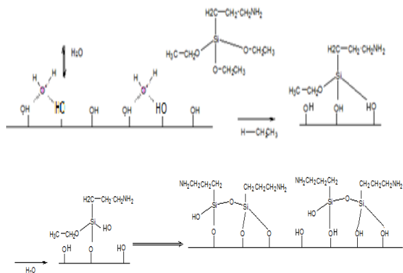
Figura 1. Mecanismo de reacción de la silanización
