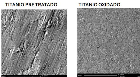
Figura 7. Imágenes de Titanio pretratado y oxidado obtenidas por SEM
