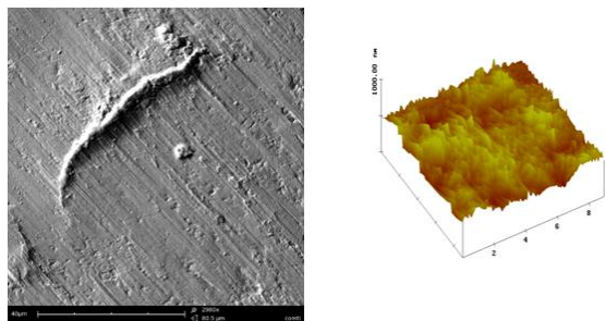
Figura 6. Imágenes de Titanio comercial, antes de ser sometido a tratamiento químico, SEM y AFM
