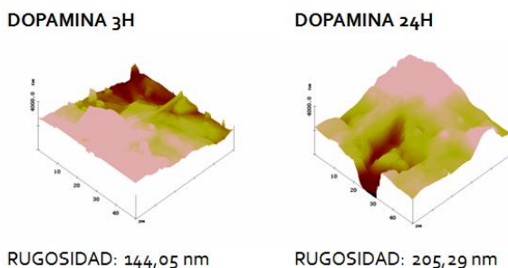
Figura 10. Imágenes de Titanio con dopamina 3 horas y 24 horas, obtenidas por AFM
