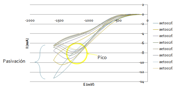
■ Figura 3. Voltamograma cíclico registrado en solución acuosa que contiene monómero AEMA, entre Vca y -1.6 V. velocidad de barrido 20 mV/s. AET0026A
