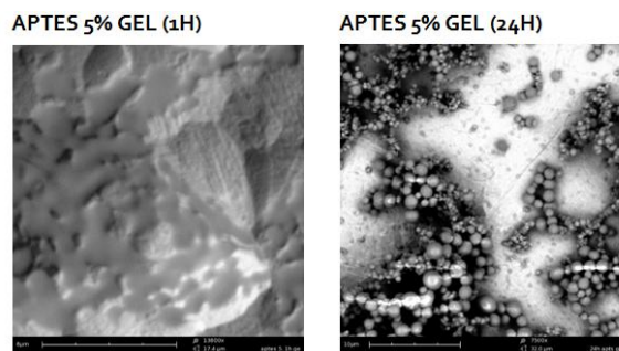
Figura 11. Imágenes de Titanio con 5% APTES 1 hora y 24 horas en incubación de 1 y 24 horas en gelatina, obtenidas por SEM
