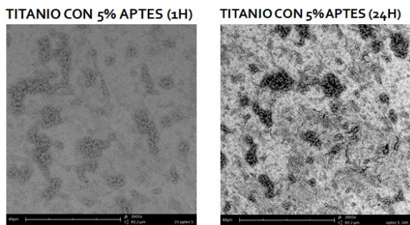
Figura 8. Imágenes de Titanio con 5% APTES 1 hora y 24 horas, obtenidas por SEM
