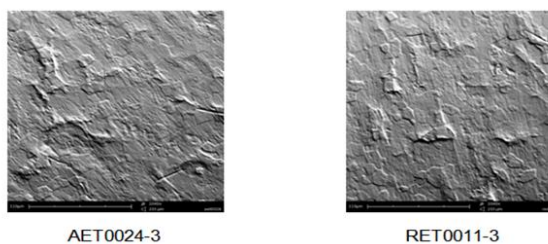
Figura 4. Imágenes de superficie modificada en solución con AEMA (AET0024-3) y en solución sin AEMA (RET0011-3) obtenidas por microscopía electrónica de barrido.
