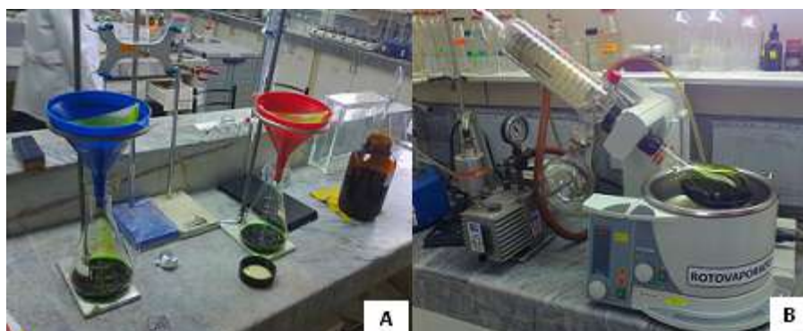
FIGURA. 2.6 (A) FILTRADO DE LA MEZCLA HOMOGENIZADA. (B) ELIMINACIÓN DEL SOLVENTE EN EL ROTOEVAPORADOR.
