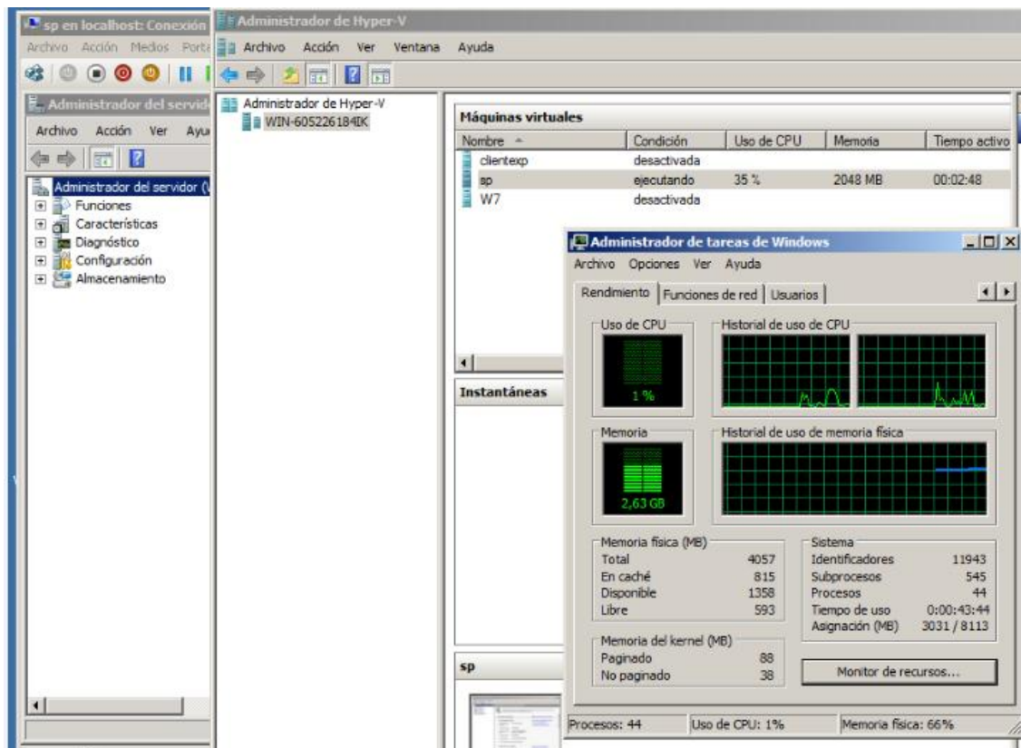
FIG 48.- INDICADORES.
