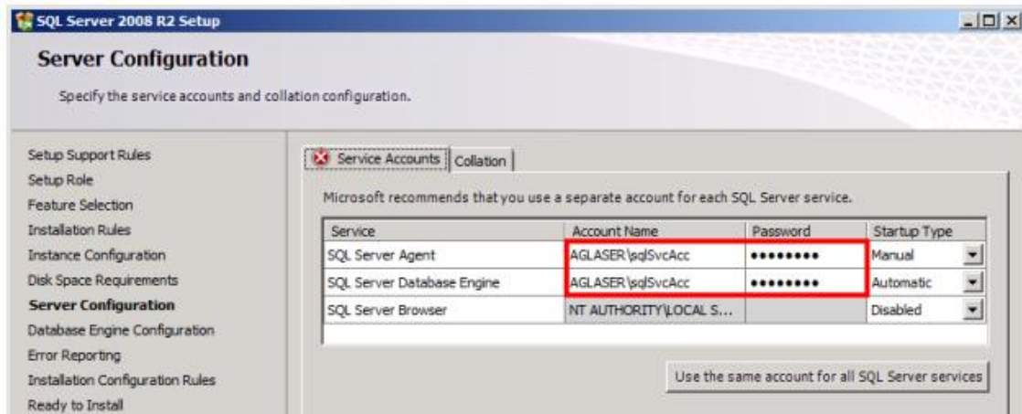
FIG 30.- SQL USER.
