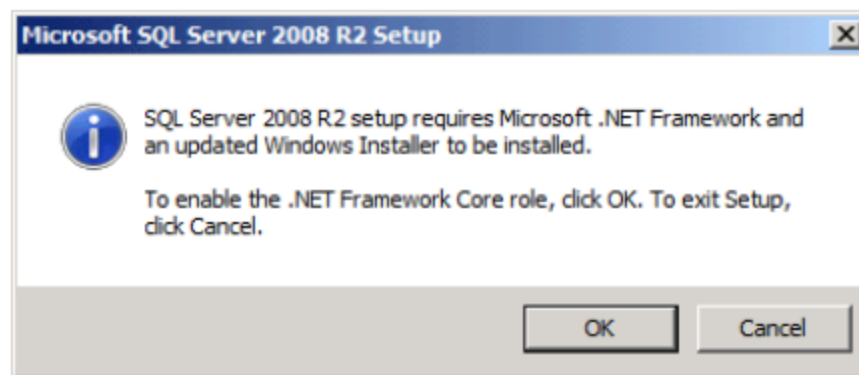
FIG 25.- INSTALAR FRAMEWORK
