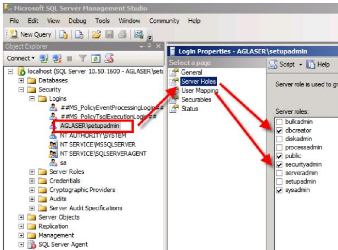
FIG 33.- ASIGNAR PERMISOS.
