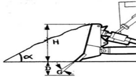
Figura 39. Forma de llenar la cuchilla del tractor al momento de cortar. (Fuente: Publicaciones del Departamento de Ingeniería de la Construcción de la Universidad de La Laguna).
