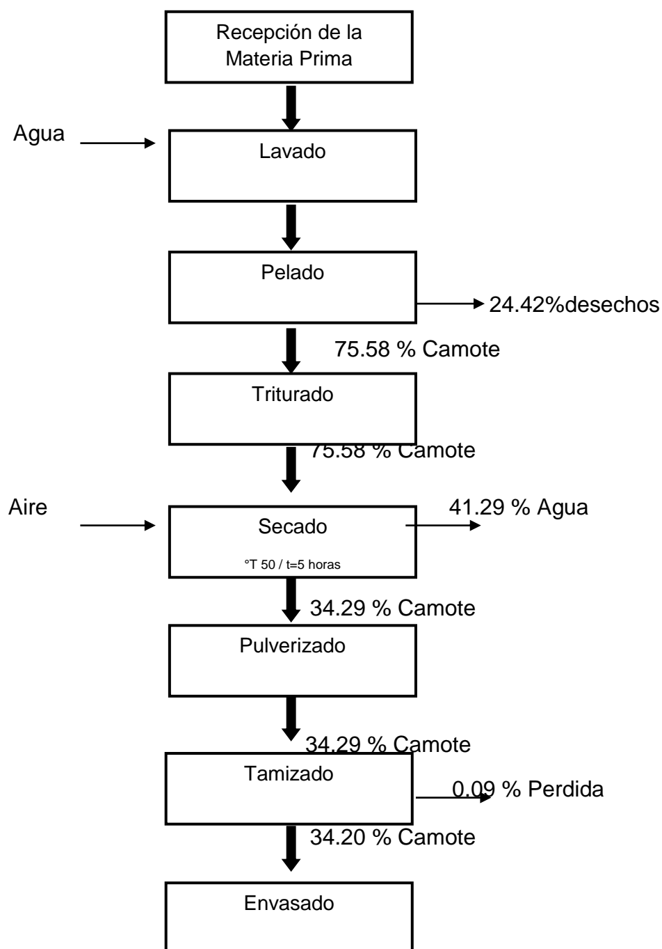
FIGURA 2.2. DIAGRAMA DE FLUJO DEL PROCESO DE ELABORACIÓN DE HARINA DE CAMOTE
