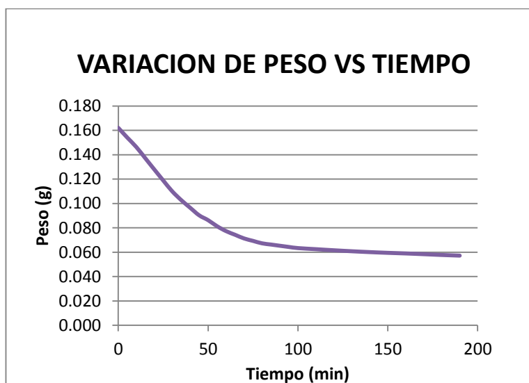
FIGURA 2.6.- VARIACIÓN DEL PESO CON RESPECTO AL TIEMPO
