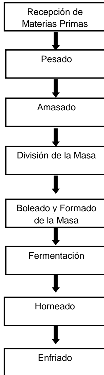
FIGURA1.2 DIAGRAMA DE FLUJO DEL PROCESO DE ELABORACIÓN DE PAN
