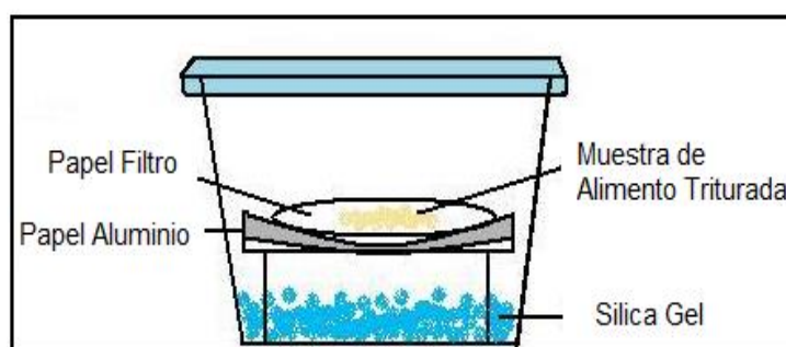
FIGURA 2.3 SISTEMA DE ADSORCION
