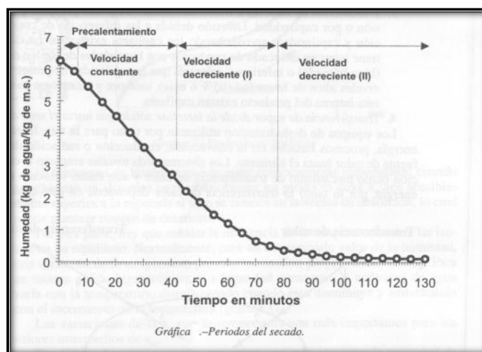
FIGURA 1.1 PERÍODOS DE SECADO
