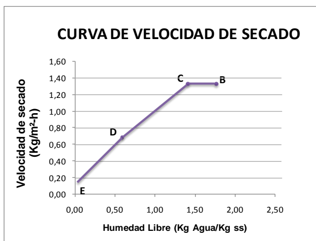
FIGURA 2.8- CURVA DE VELOCIDAD DE SECADO
