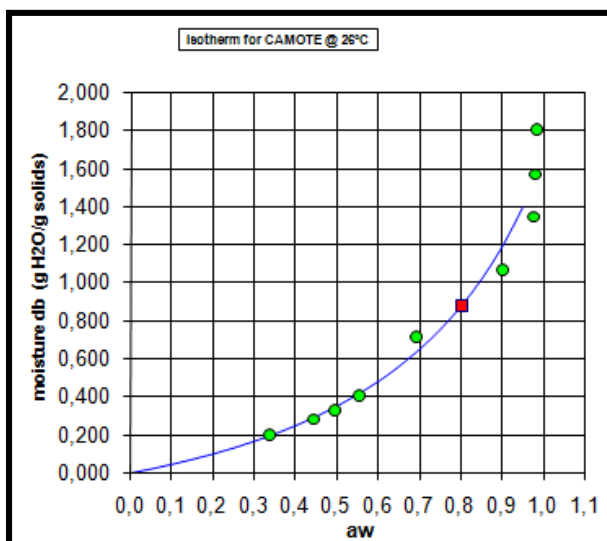
FIGURA 2.4. ISOTERMA DE SORCION
