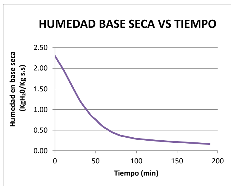
FIGURA 2.5.- VARIACIÓN DE LA HUMEDAD EN BASE SECA CON RESPECTO AL TIEMPO
