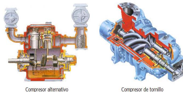
Figura 4.9. Compresores más Usados en el Mercado de la Refrigeración
