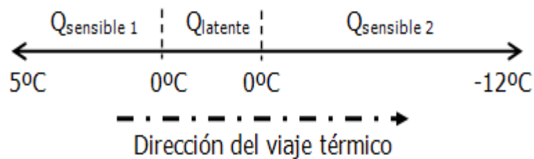
Figura 4.8. Viaje Térmico Realizado por el Camarón al entrar al Equipo de Aspersion por Salmuera
