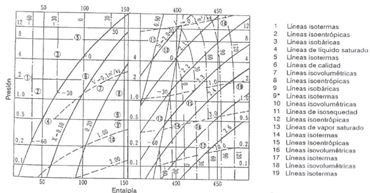
Figura 4.2. Diagrama p-h, Refrigerante Amoniaco
