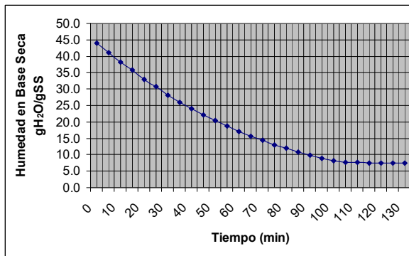
FIGURA 4.13: CURVAS DE SECADO: HUMEDAD VERSUS TIEMPO A 70°C
