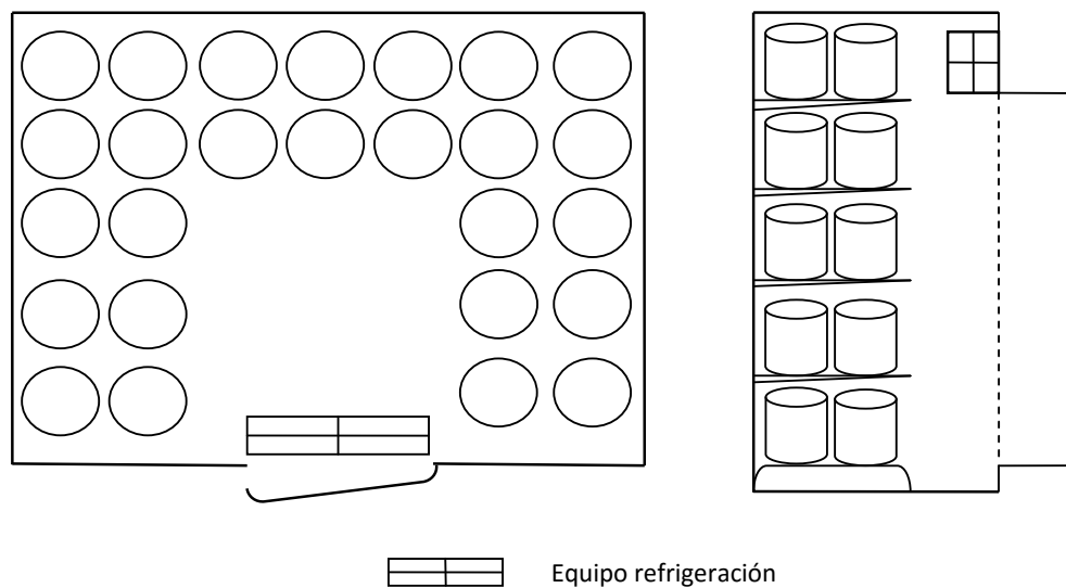
Figura 3.3 Esquema distribución estiva dentro cámara.
