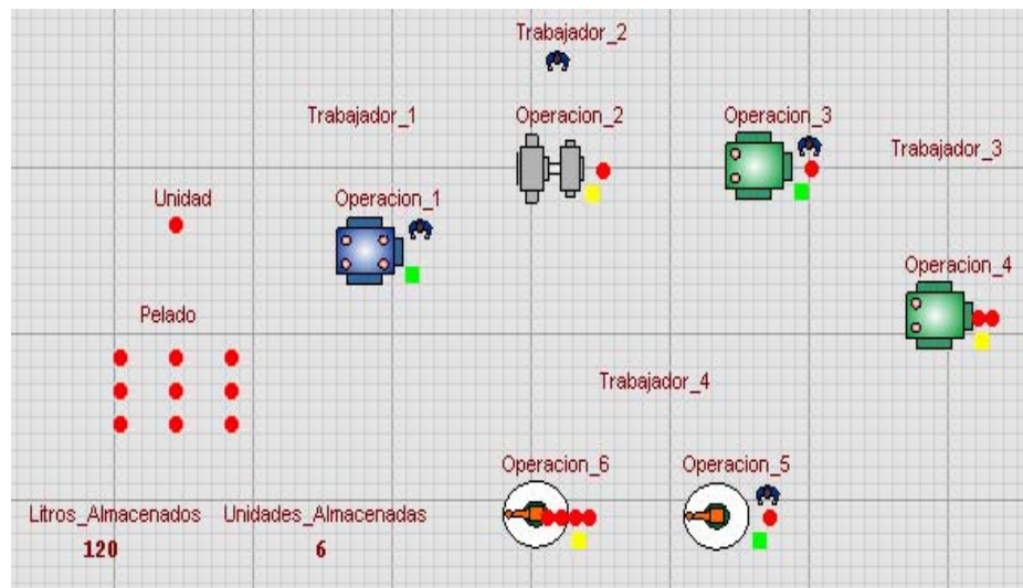
Figura 2.5 Inicio jornada laboral. Simulación línea producción (WITNESS 2008).
