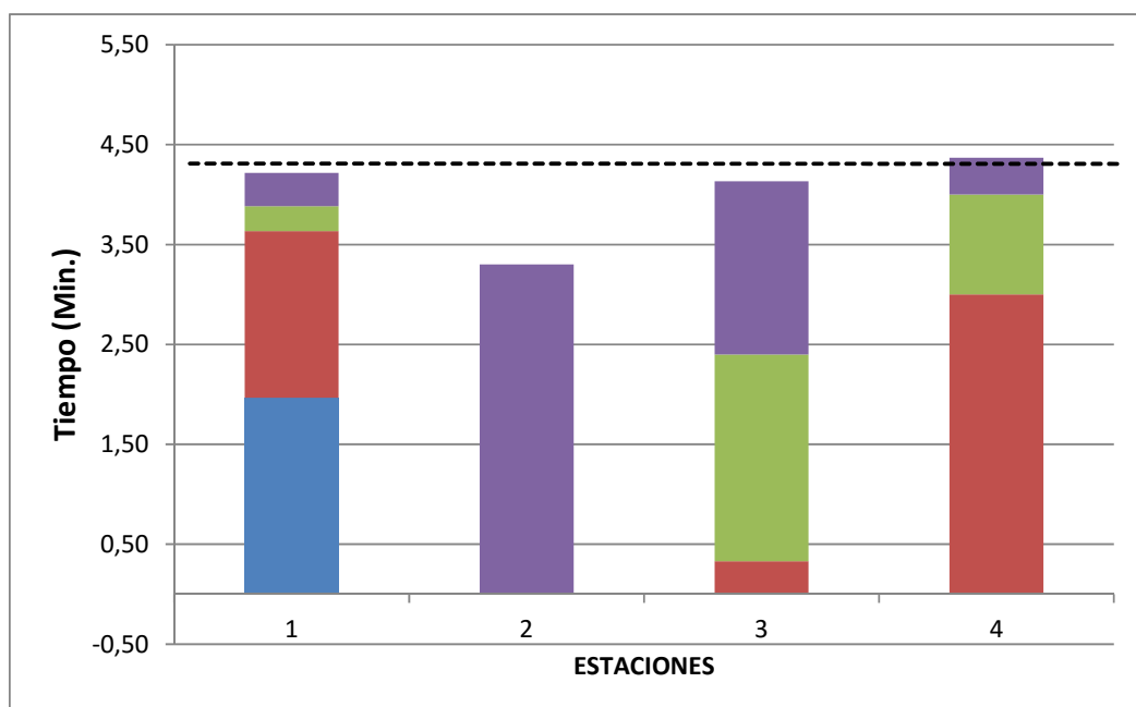
Figura 2.4 Conglomerado tiempos estaciones trabajo balanceada.
