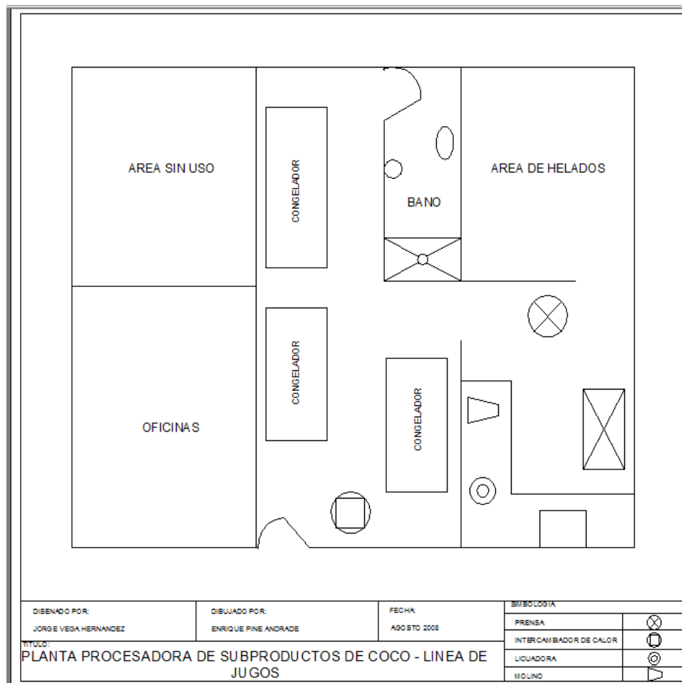
Plano 1. Diseño planta actual (autocad 2008).
