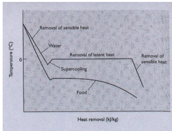
Figura 3.1. Curva de Congelación.
