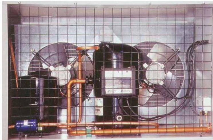
Figura 3.9 Condensador.
