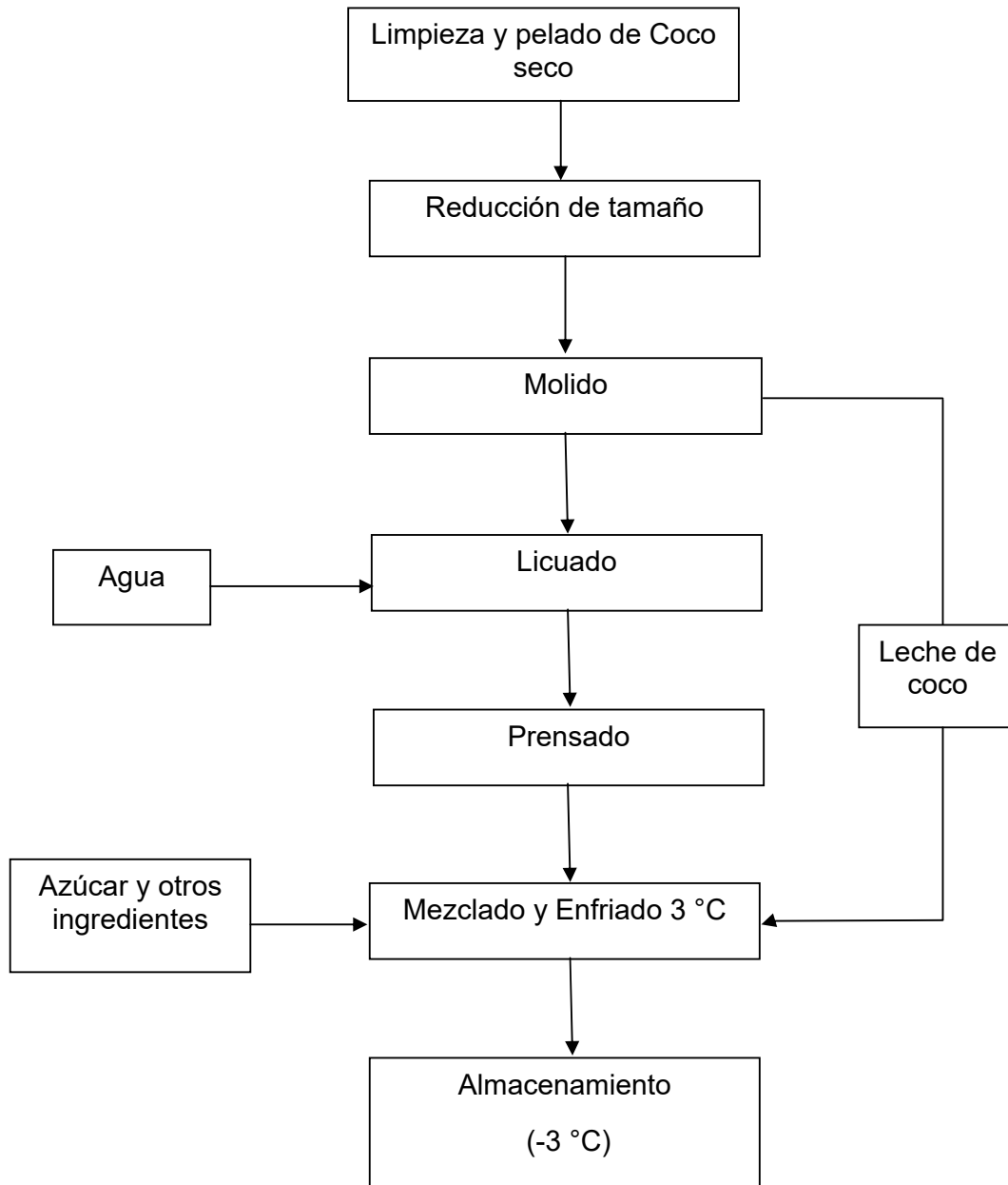
Figura 1.1 Diagrama de flujo de Proceso.
