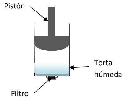
Figura 1.4 Esquema del sistema filtro-prensa.
