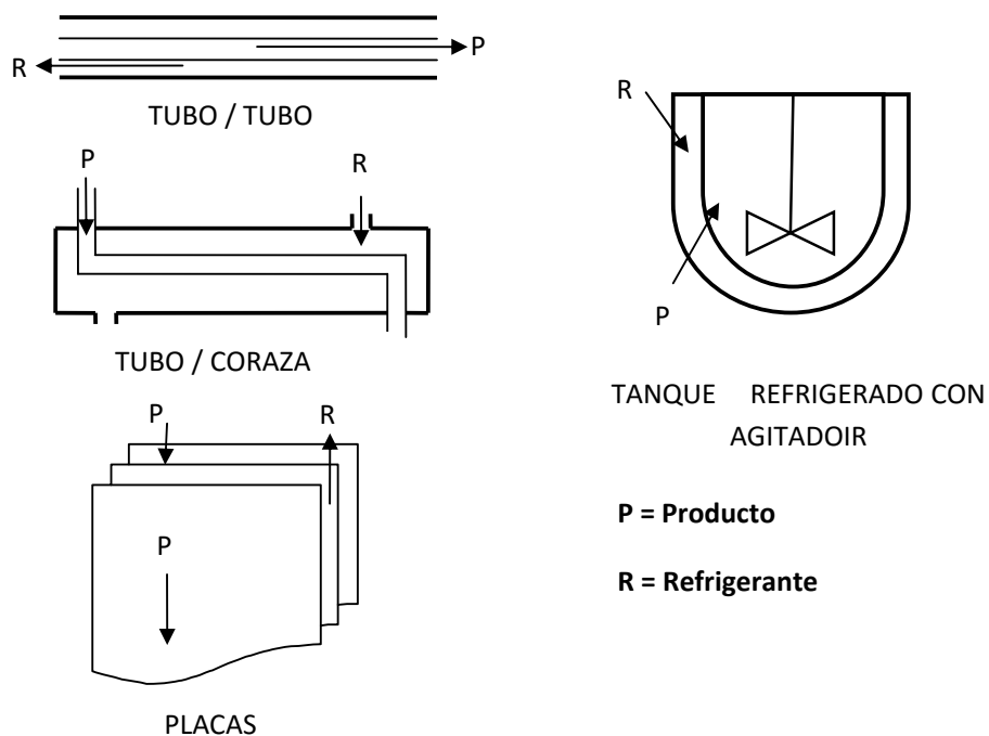
Figura 3.10 Esquema intercambiadores de calor.
