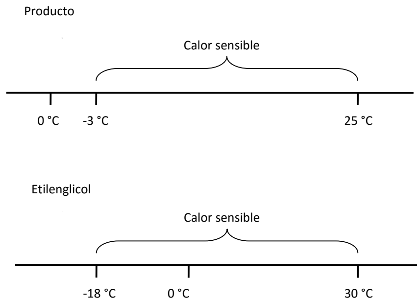
Figura 3.11 Viaje térmico de productos en el intercambiador de calor.
