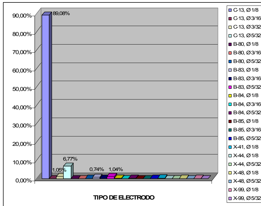
FIGURA 3.1. DIAGRAMA DE PARETO DE ELECTRODOS PRODUCIDOS
