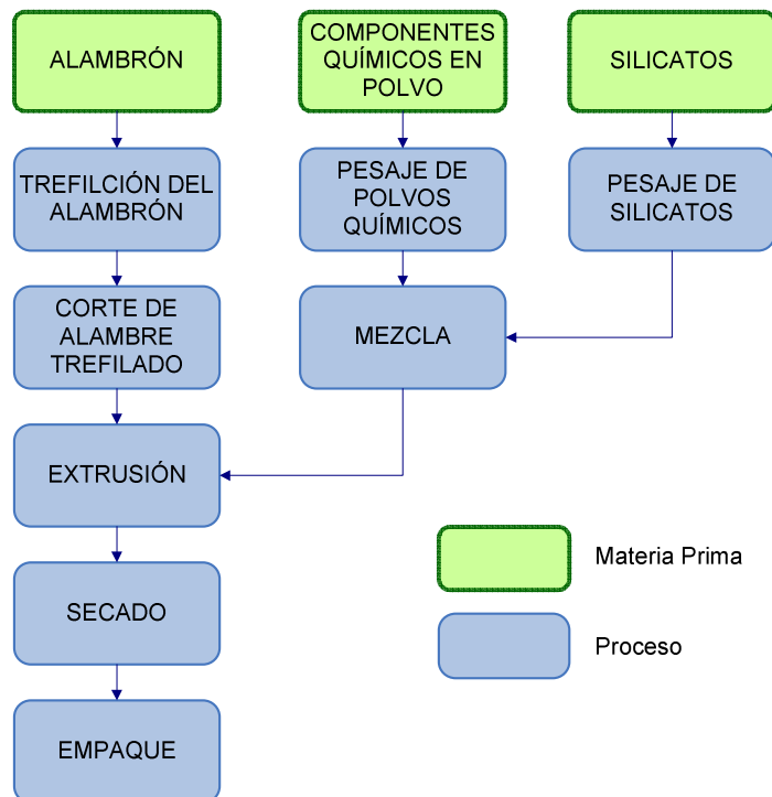
FIGURA 3.2. DIAGRAMA DE FLUJO DEL PROCESO DE FABRICACIÓN DE ELECTRODOS
