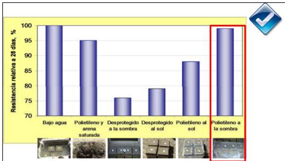
Gráfica 5.22: Influencia de las condiciones de Curado en la Resistencia a los 28 días
