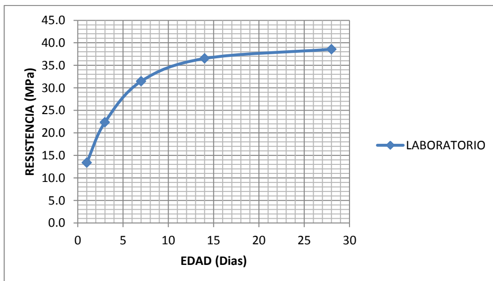
Grafica 4.7: Gráfica Resistencia a la Compresión vs Tiempo para cilindros curados en el Laboratorio
