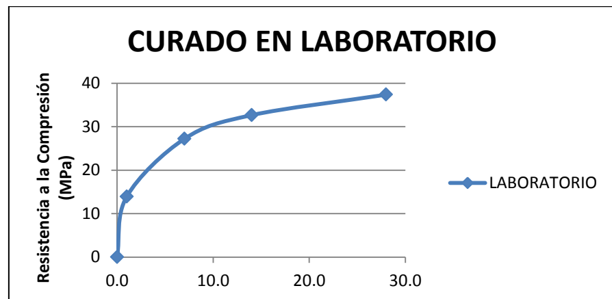
Gráfica 5.17: Desarrollo de la Resistencia de Cilindros curados en Laboratorio
