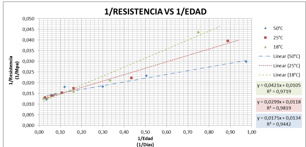
Grafica 4.5: Gráfica 1/Resistencia vs. 1/Edad
