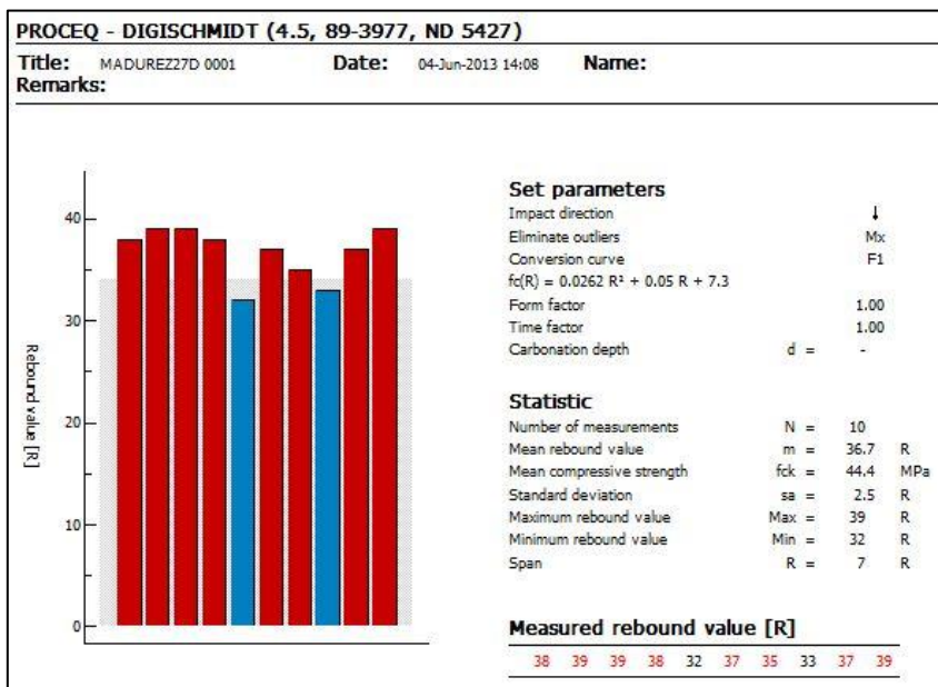
Gráfica 5.25: Gráfica de Numero de Rebotes obtenidos por el Esclerómetro en Prueba Número 1
