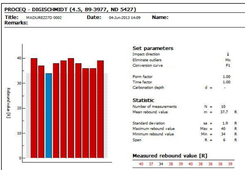
Gráfica 5.26: Gráfica de Numero de Rebotes obtenidos por el Esclerómetro en Prueba Número 2
