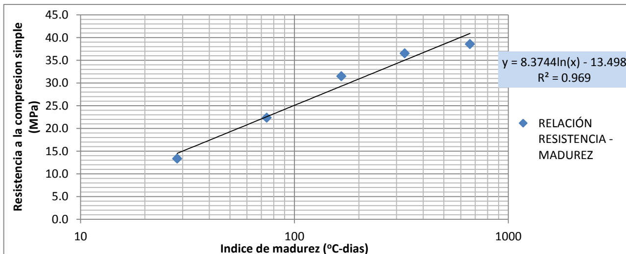
Grafica 4.10: Gráfica Resistencia a la compresión vs índice de madurez
