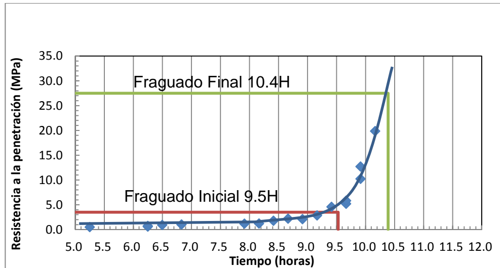
Grafica 4.3: Gráfica Resistencia a la Penetración vs Tiempo para Mortero a 50°C
