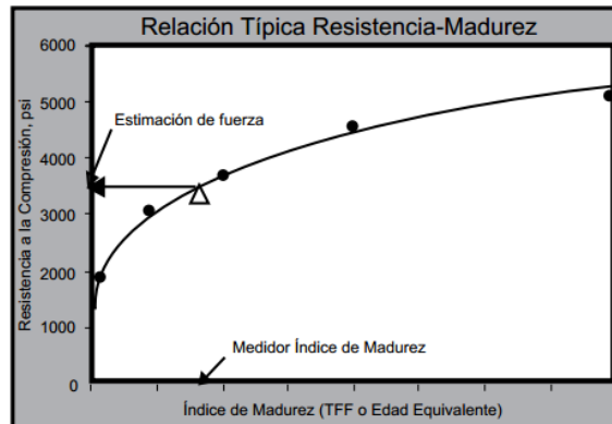
Gráfica 2.2 Relación Resistencia vs. Madurez.
