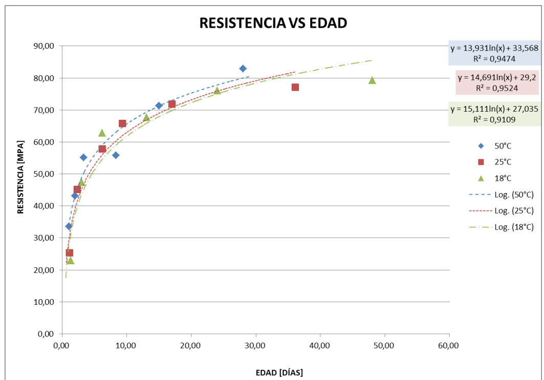
Grafica 4.4: Gráfica Resistencia vs Edad de los cubos de Mortero curados a 18°C, 25°C y 50°C
