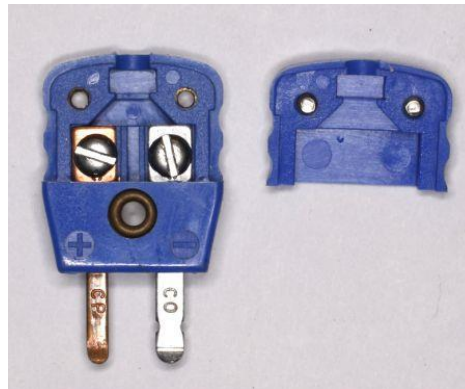
Grafica 3.24: Termocoupla Tipo T
