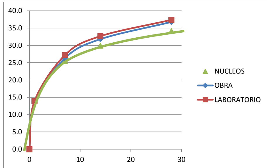
Gráfica 5.21: Gráfico Comparativo de la influencia del curado en el Desarrollo de la Resistencia.
