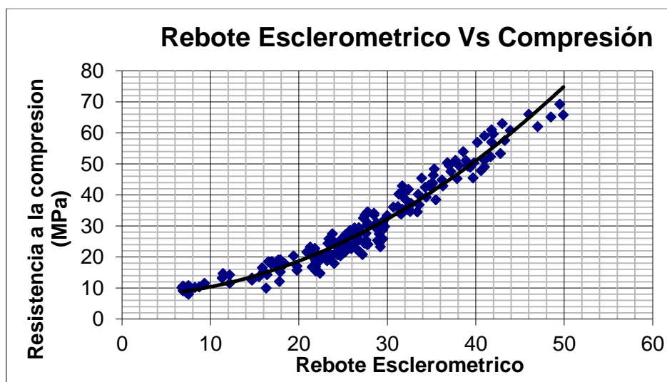
Gráfica 5.27: Gráfica Rebote Esclerométrico vs Resistencia a la Compresión
