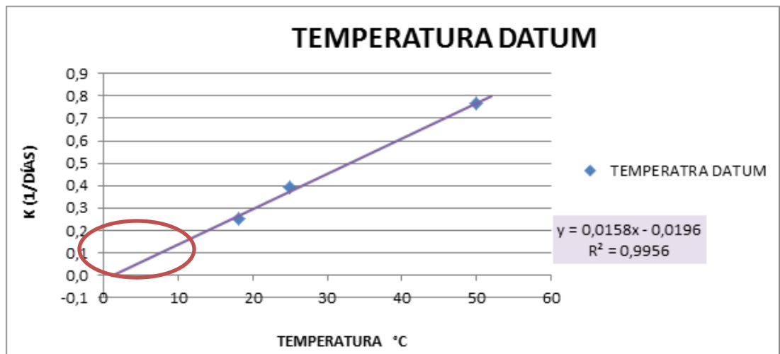
Grafica 4.6: Gráfica Factor K vs Temperatura
