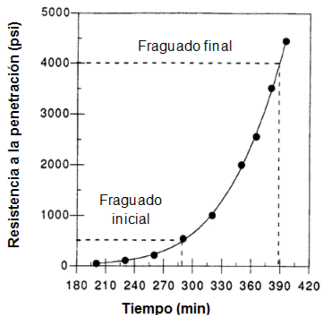
Grafica 3.14: Grafica Resistencia a la Penetración vs. Tiempo (Nota: no se encuentra a escala real)
