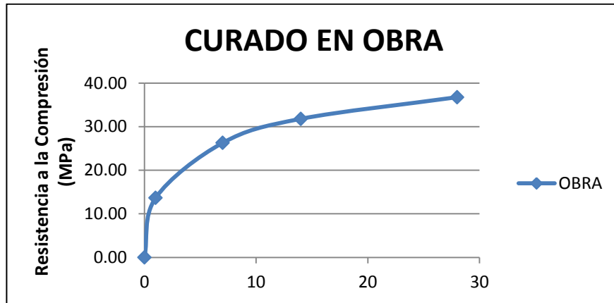
Gráfica 5.15: Desarrollo de Resistencia de cilindros en Obra
