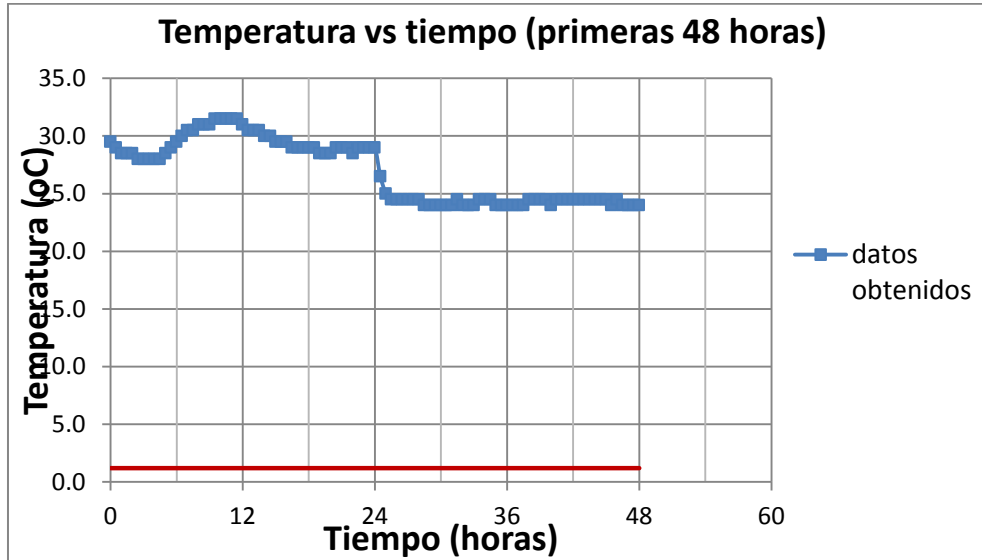
Grafica 4.9: Variación de Temperatura de probetas a las 48 horas, 7 días, 14 días y 28 días
