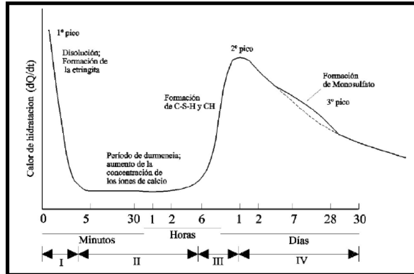
Gráfica 3.1 Producción de calor de un cemento portland Tipo I
