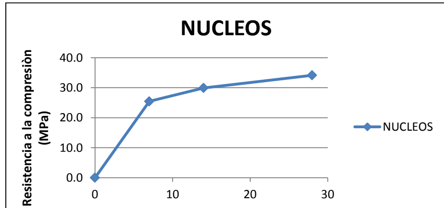
Gráfica 5.19: Gráfica Resistencia a la Compresión vs. Edad de Núcleos Calados
