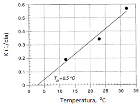
Gráfica 3.5: Ejemplo de un Gráfico de Valores K
