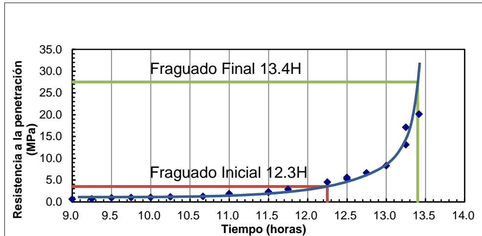
Grafica 4.2: Gráfica Resistencia a la Penetración vs Tiempo para Mortero a 25°C
