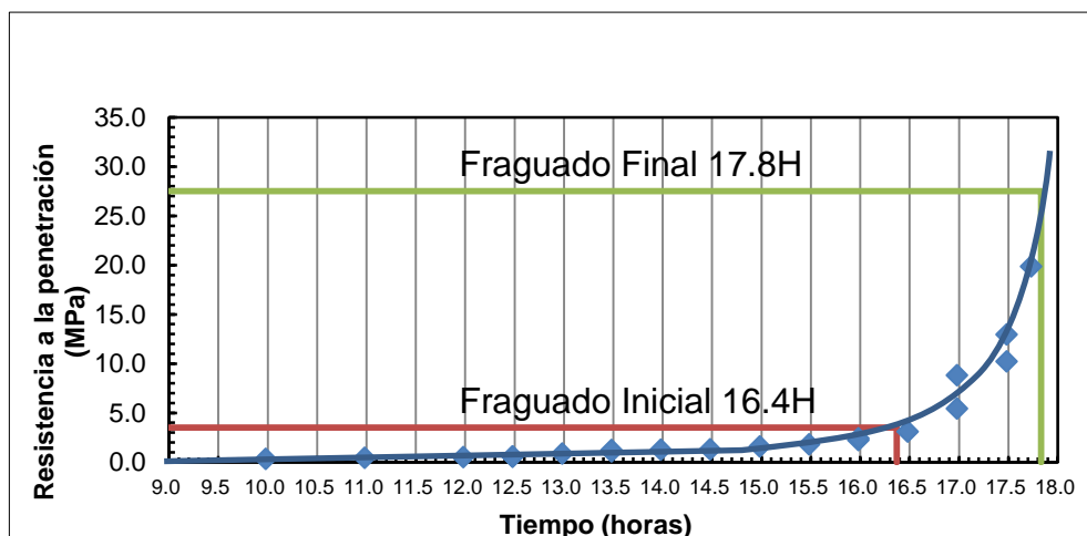
Grafica 4.1: Gráfica Resistencia a la Penetración vs Tiempo para Mortero a 18°C
