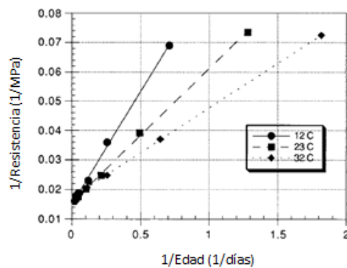
Gráfica 3.4: Inversa de la Resistencia vs. Inversa de la Edad
