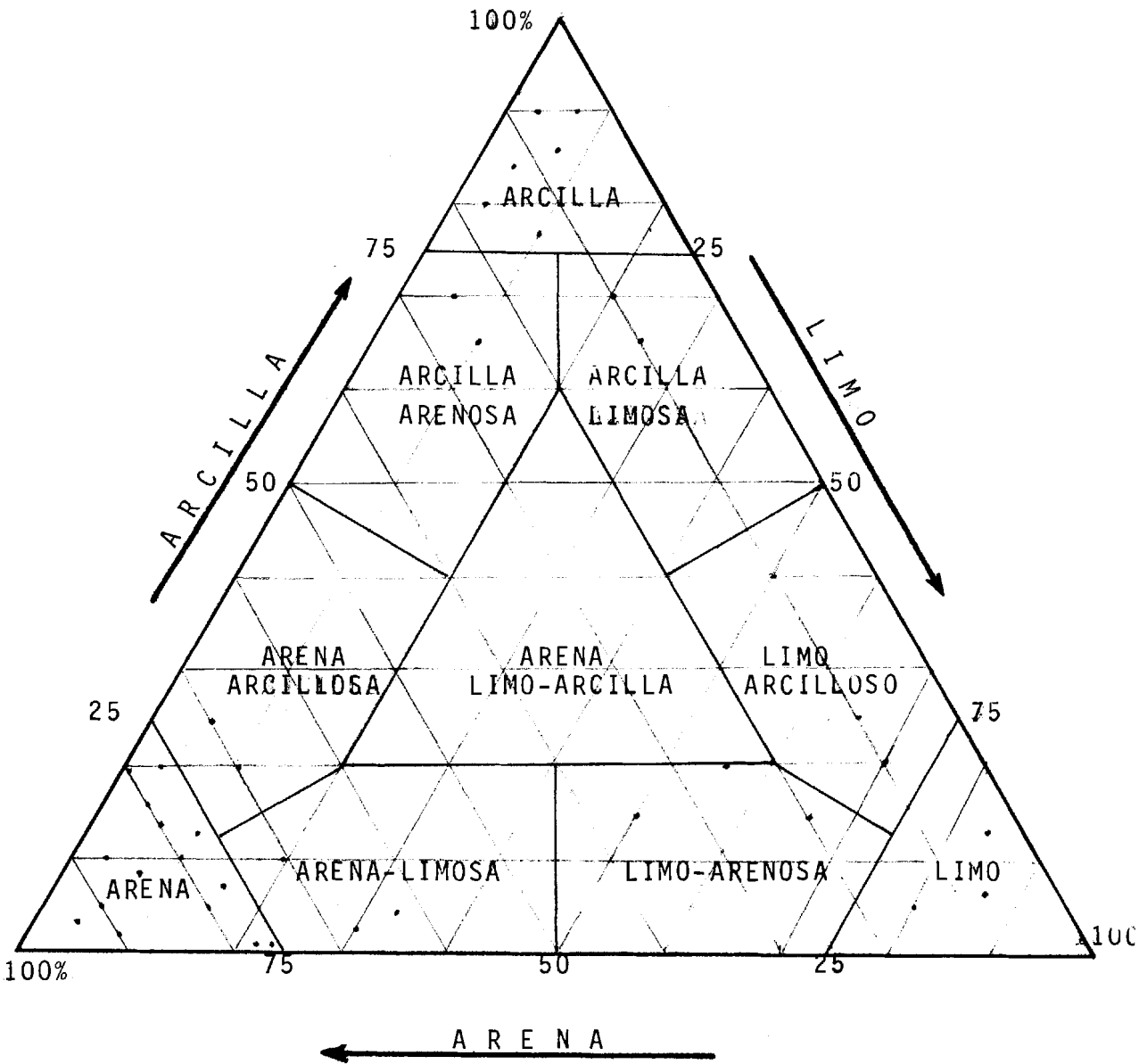
FIG. N°17 Diagrama triangular de Sheppard mostrando la clasificación granulométrica para los sedimentos del Miembro Placer.
