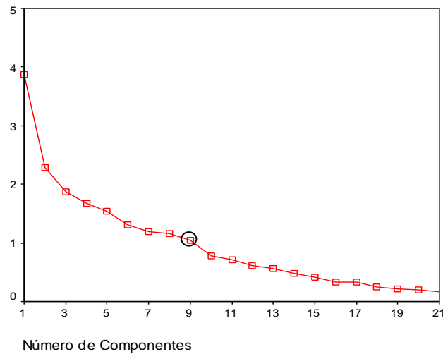
Gráfico de Sedimentación de los Componentes Principales obtenidos a partir de los datos originales
