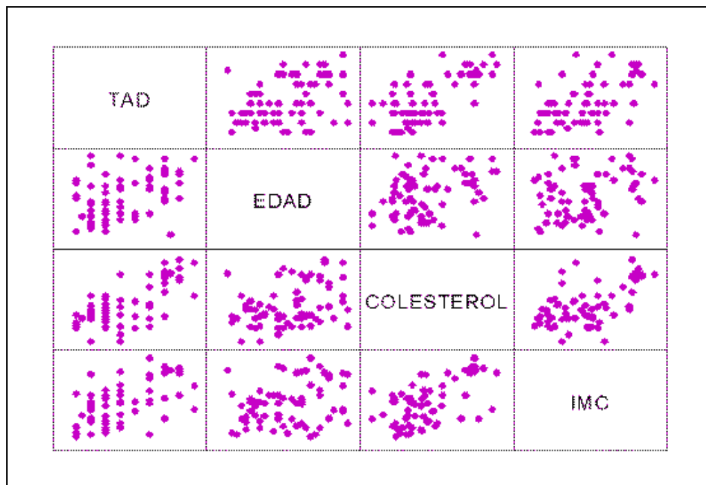
FIGURA 2.9. SALIDA DE SPSS PARA ANALIZAR LA CORRELACIÓN LINEAL ENTRE MÚLTIPLES VARIABLES.
