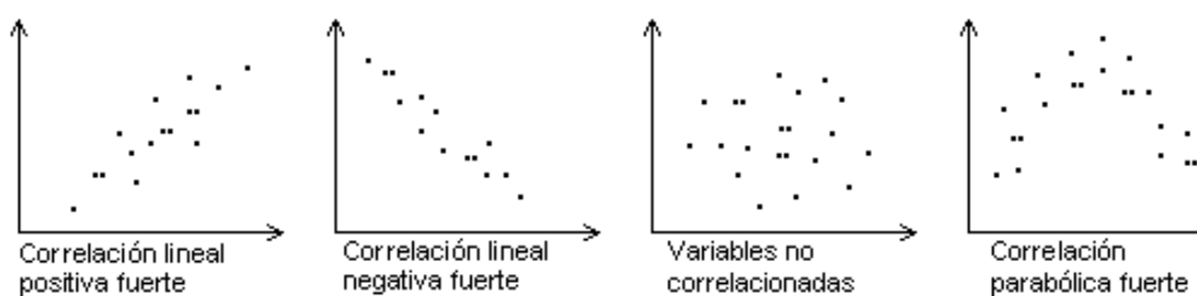
FIGURA 2.5. EXPLICACIÓN GRÁFICA DE LA CORRELACIÓN Fuente: Moore David S., The Active Practice of Statistics .
