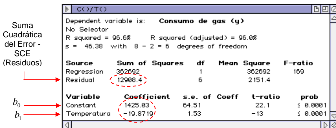
FIGURA 2.6. VENTANA RESULTANTE DE UN CÁLCULO DE REGRESIÓN EN DATA DESK 10.0
