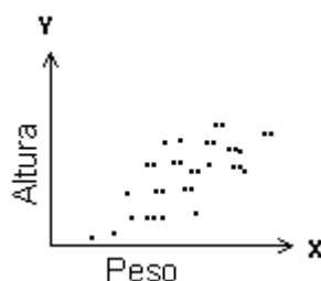
FIGURA 2.4. EJEMPLO DE DIAGRAMA DE DISPERSIÓN Fuente: Moore David S., The Active Practice of Statistics .
