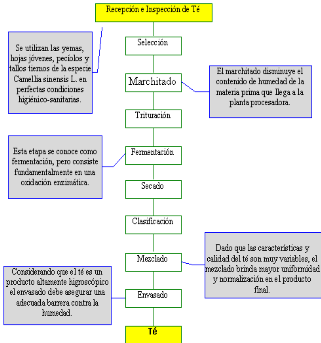
Gráfico XXVIII: Diagrama de Proceso de Post cosecha de Producción de Té
