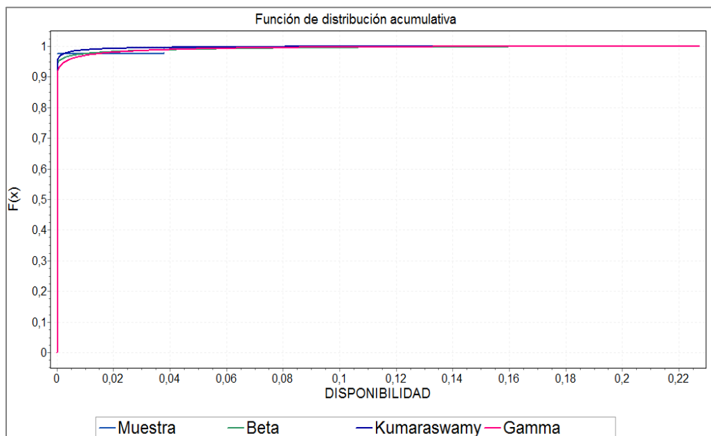
Figura 4.15: Modelado estadístico del canal 23
