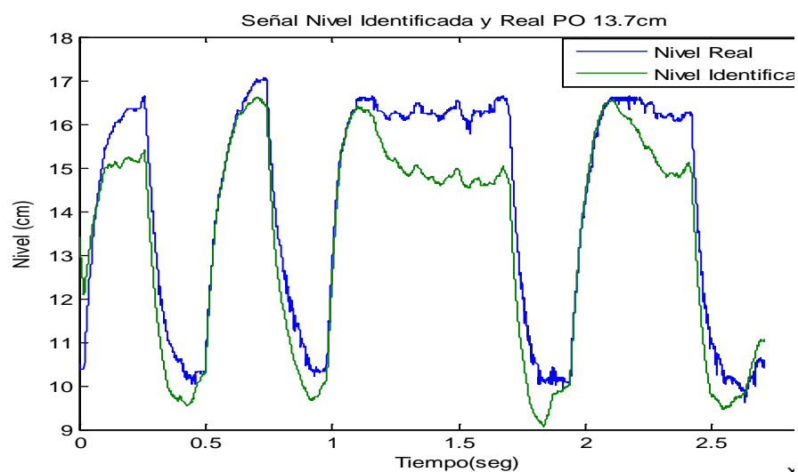
FIGURA 4.17. Respuesta a la simulación del modelo identificado para PO 13.7 cm
