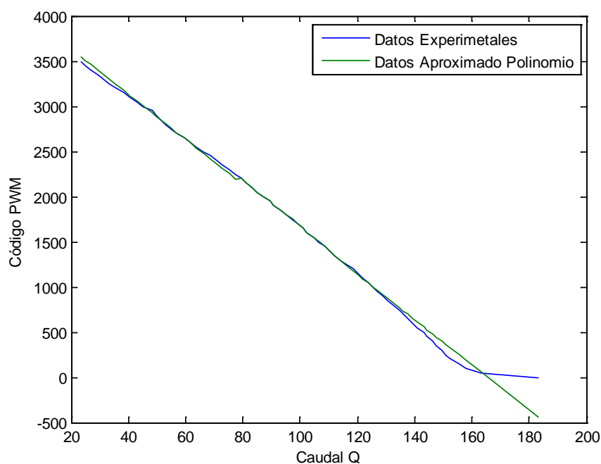
FIGURA 4.1. Grafica del caudal vs PWM suministrado a la planta
