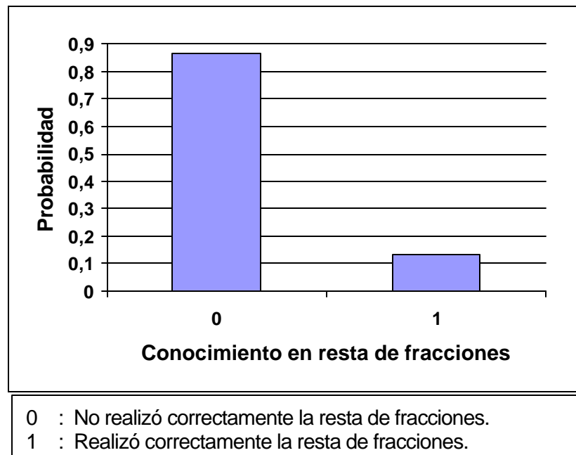
HISTOGRAMA DE PROBABILIDADES PARA LA VARIABLE X_9 (RESTA DE FRACCIONES)
