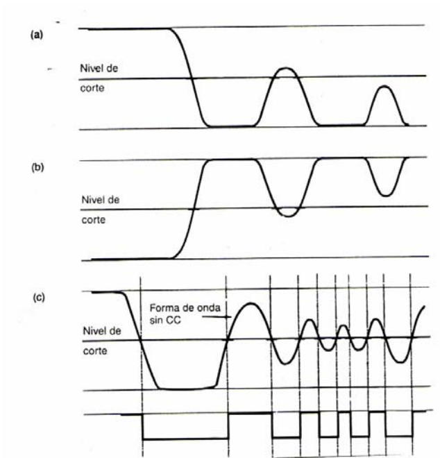
Figura 5.40 La división en secciones, o troceado, de una señal.
