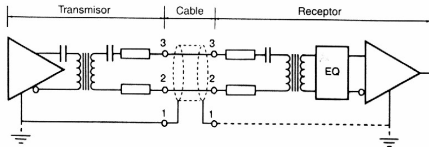
Figura 7.2 Circuito eléctrico recomendado para la interfaz normalizado de dos canales.
