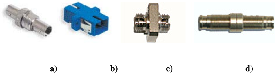
Figura 7.46 Acopladores o Adaptadores para a) ST b) SC c) FC d) DIN
