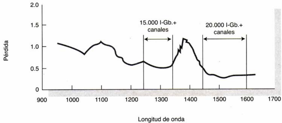
Figura 6.3 Pérdidas en una fibra óptica en función de la longitud de onda
