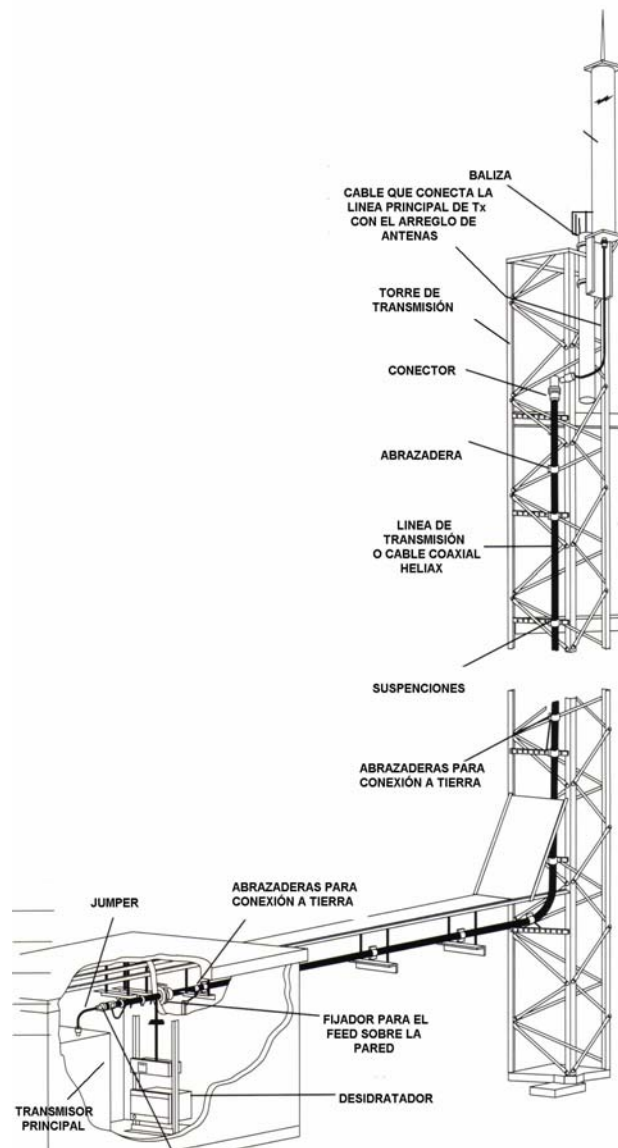
Figura 3.4 Planta Transmisora
