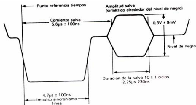
Figura 4.4 Sala de subportadora de color, sistema PAL
