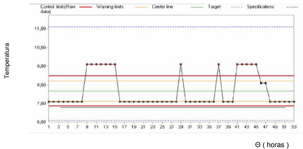
FIG. 3.4.1.6 GRÁFICA DE CONTROL SOBRE LA ENTRADA DE AGUA DEL SECTOR 2
