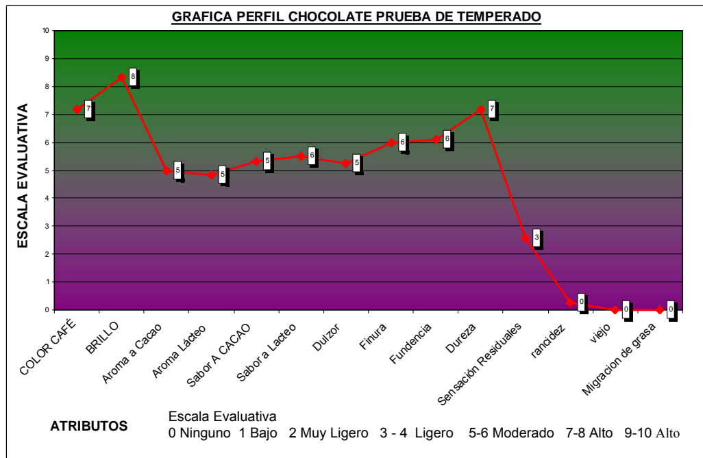
FIG. 4.3.3 PERFIL CHOCOLATE PRUEBA
