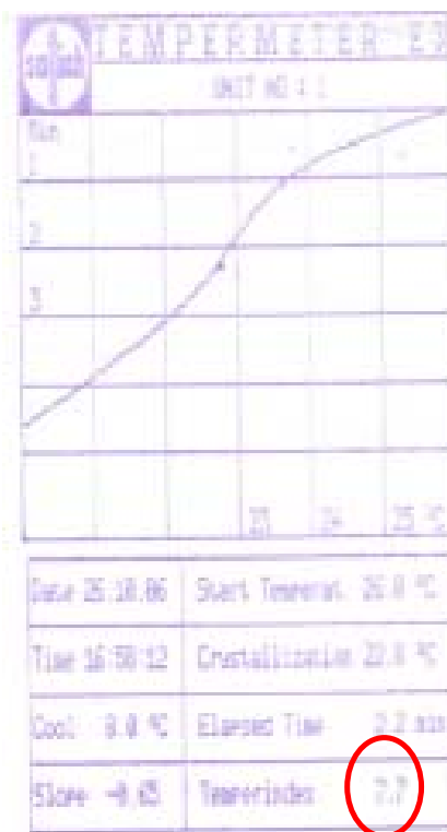
FIG. 4.2.1 CURVA DE TEMPERADO ANTES DE LA PRUEBA DE TEMPERADO CON UN ÍNDICE DE 7.7
