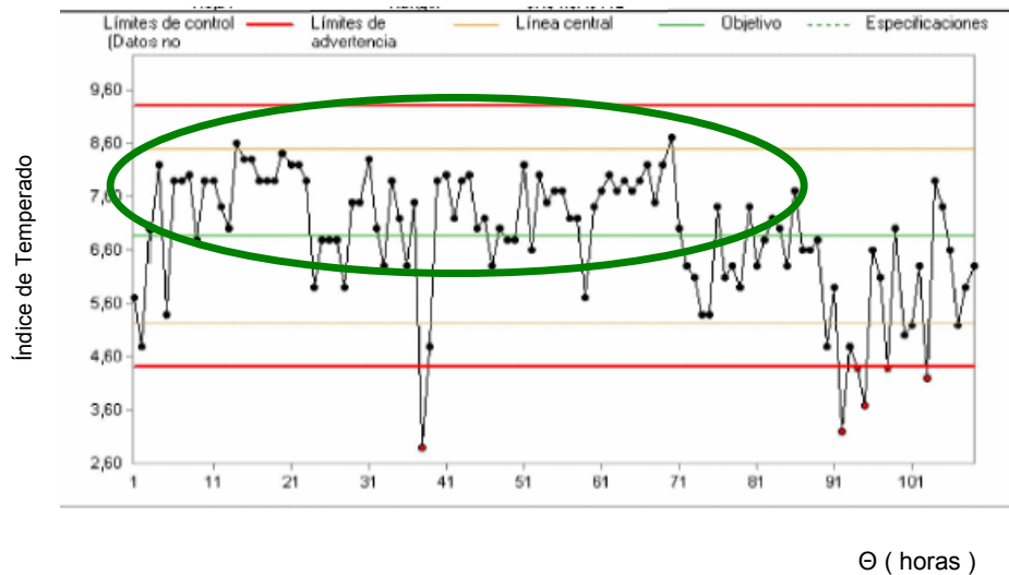
FIG. 3.4.1.1 GRÁFICA DE CONTROL SOBRE EL ÍNDICE DE TEMPERADO EN EL MES DE JULIO
