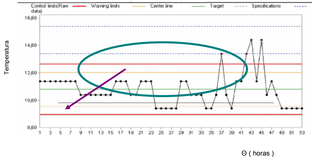
FIG. 3.4.1.7 GRÁFICA DE CONTROL SOBRE LA SALIDA DE AGUA DEL SECTOR 2
