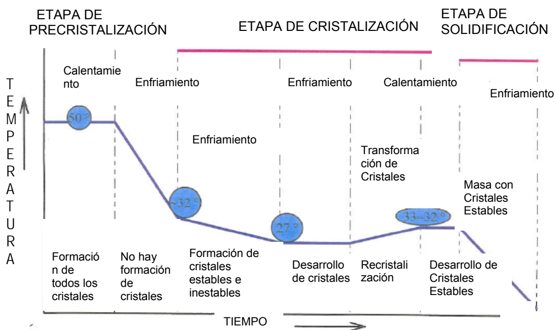
FIG. 3.1 ETAPAS DE FORMACIÓN DE CRISTALES DEL CHOCOLATE.
