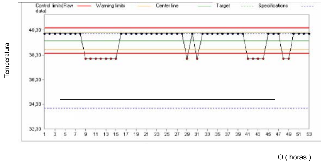
FIG. 3.4.1.9 GRÁFICA DE CONTROL SOBRE LA ENTRADA DE AGUA DEL SECTOR 3
