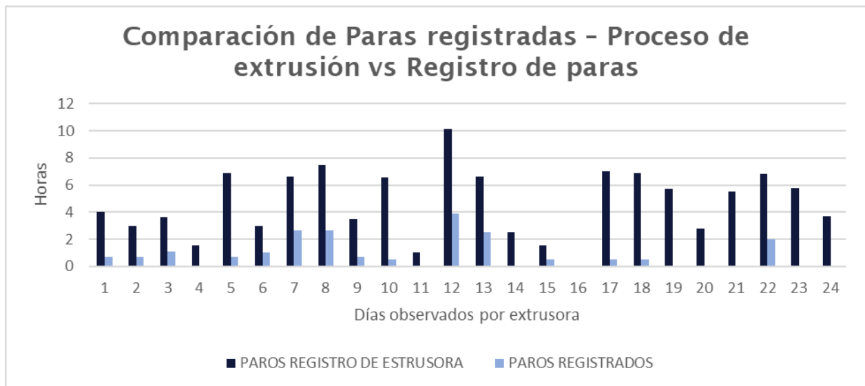
Figura 2.9 Gráfico comparativo entre las horas de para del registro de extrusión y las horas de paros del registro de paradas.
