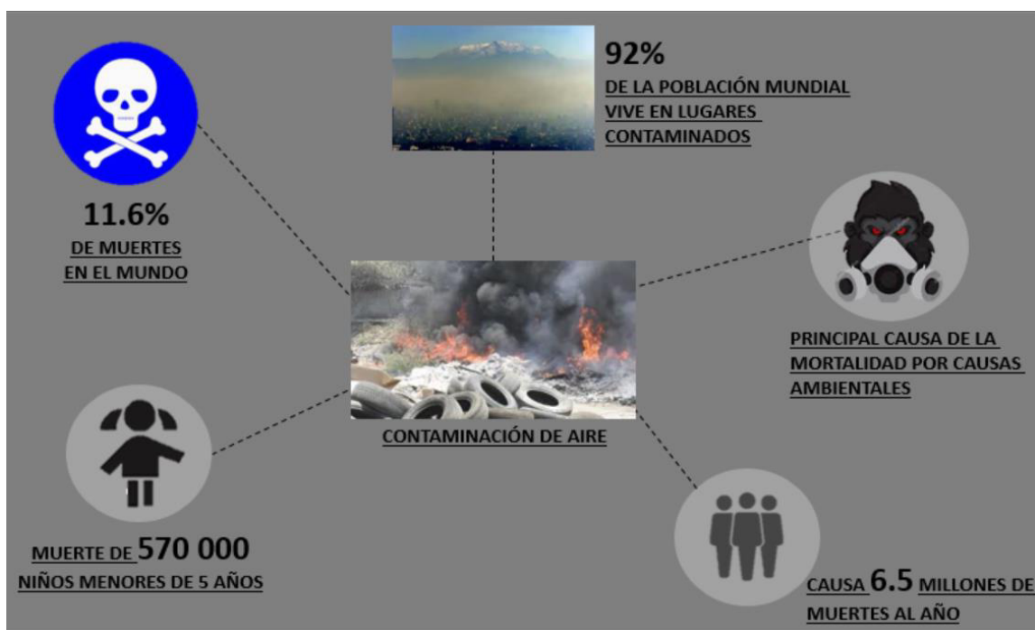
Gráfico 1.1 El 92% de la población mundial sufre por la contaminación del aire (OMS)
