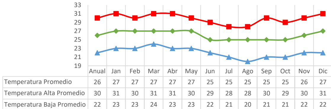
Gráfico 1.2 Temperatura Guayaquil registro de 16 años – Guayaquil
