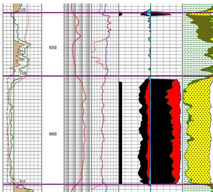
Figura 1.3 Registro Eléctrico del Pozo Sacha 028. en donde se observa el Registro GR de la Arenisca U, mostrando una buena calidad de arena en la u inferior.
