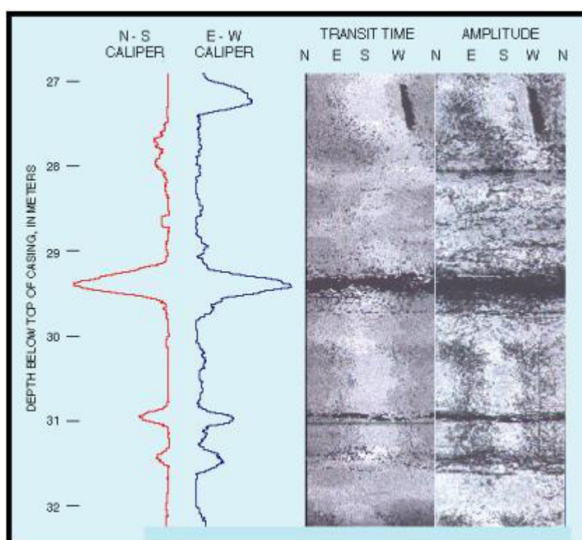
Figura 3.5 Representación de un Registro Caliper (Colores azul y rojo) a la izquierda. Fuente: Foto Tomada de Internet.
