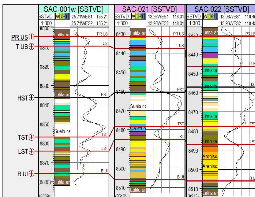
Figura 4.15 Representación de los Ciclos Sedimentarios Menores.
