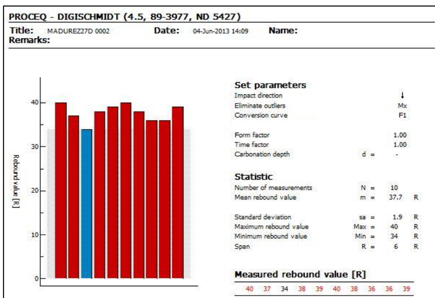
Gráfica 5.26: Gráfica de Numero de Rebotes obtenidos por el Esclerómetro en Prueba Número 2
